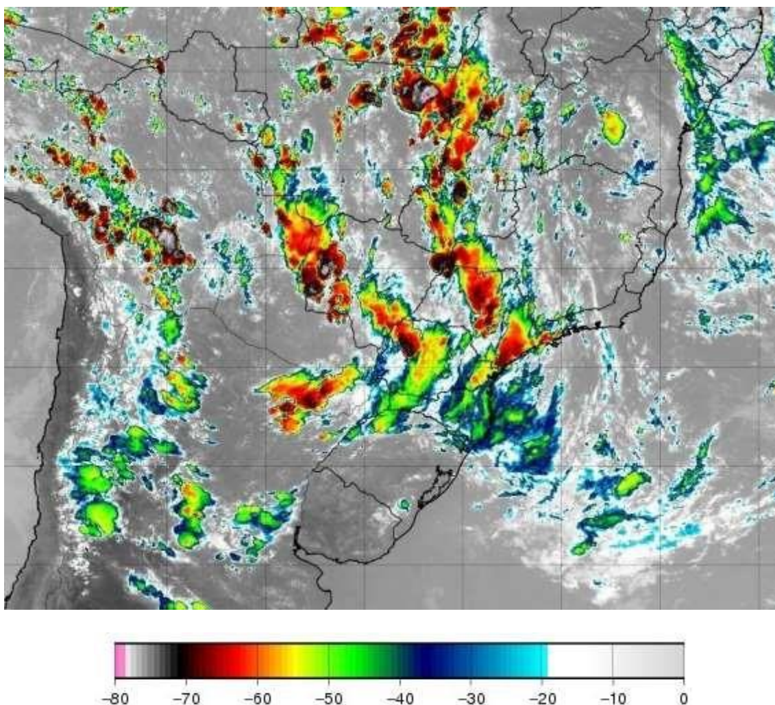
Figura 1 - Imagem de satélite no infravermelho com realce do satélite GOES-16 as 20:00 UT do dia 19/01. As cores indicam diferentes temperaturas dos topos das nuvens.
