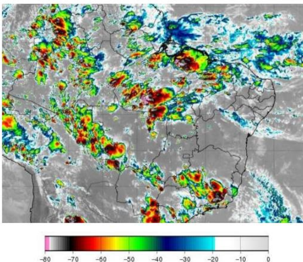
Figura 1 - Imagem de satélite no infravermelho com realce do satélite GOES-16 às 21:00 UT do dia 14/02. As cores indicam diferentes temperaturas dos topos das nuvens.
