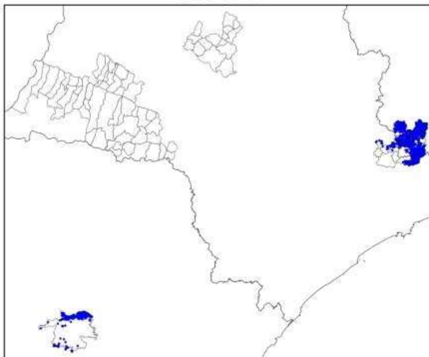
Figura 2 – Mapa de incidência de descargas atmosféricas nuvem-solo e intranuvem para os dias: (a) 01/10; (b) 02/10; (c) 03/10; (d) 04/10; (e) 05/10; e (f) 06/10. Cada ponto corresponde ao local de ocorrência de uma descarga.
