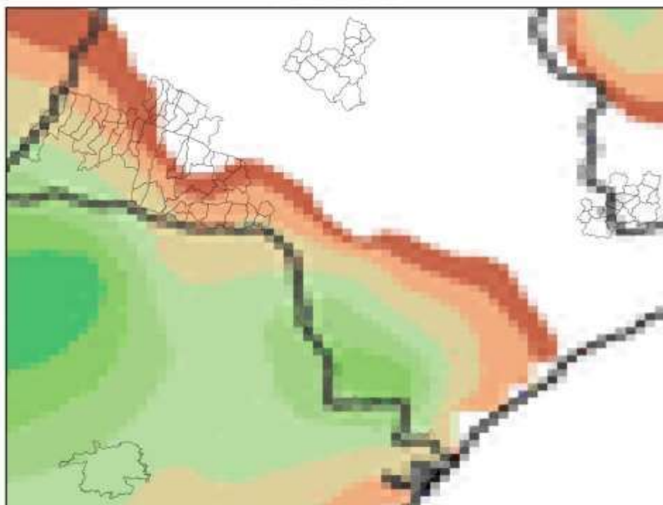
Mapa de Precipitação 2021-10-03
