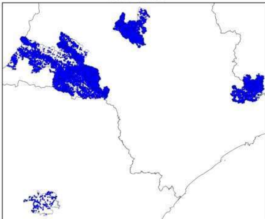
Mapa de Descargas Atmosféricas 2021-10-03
