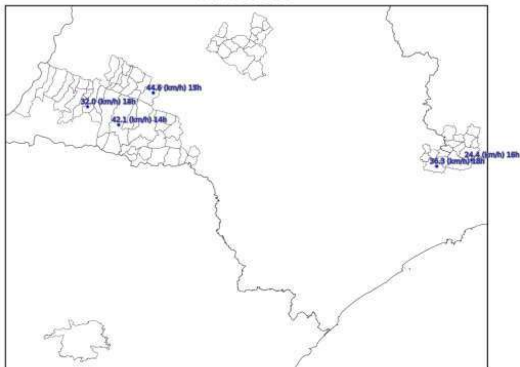
Mapa de Rajada Máxima 2021-10-02
