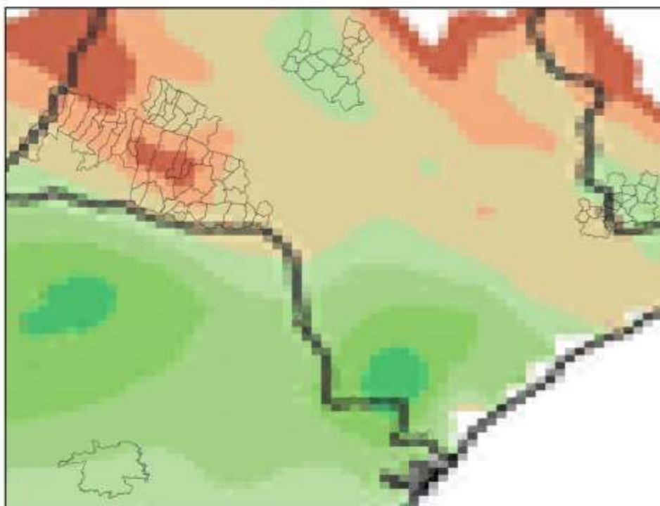
Mapa de Precipitação 2021-10-04
