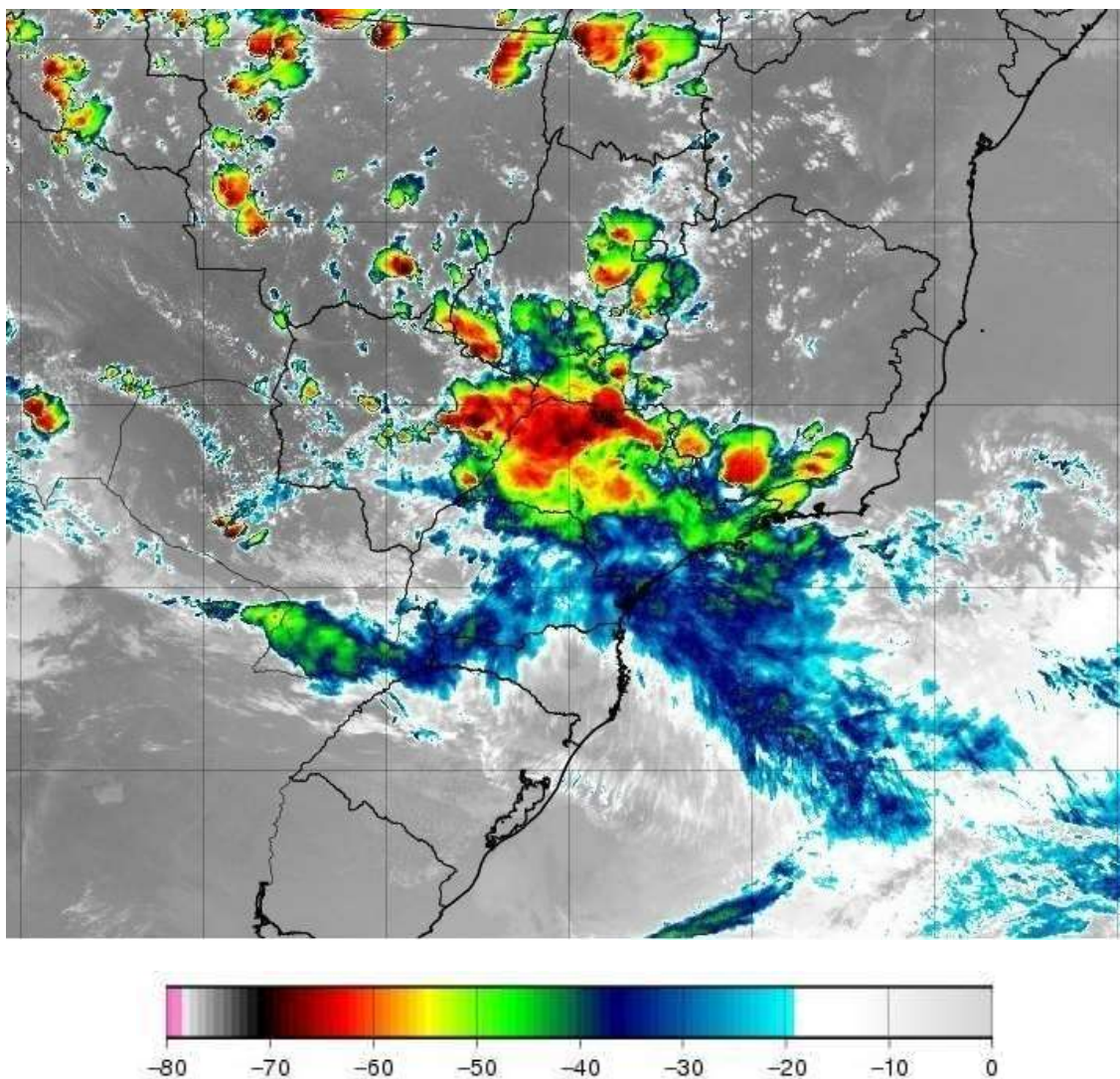
Figura 1 - Imagem de satélite no infravermelho com realce do satélite GOES-16 durante um dos períodos de máxima intensidade do evento às 20:00 UT do dia 01/10. As cores indicam diferentes temperaturas dos topos das nuvens.
