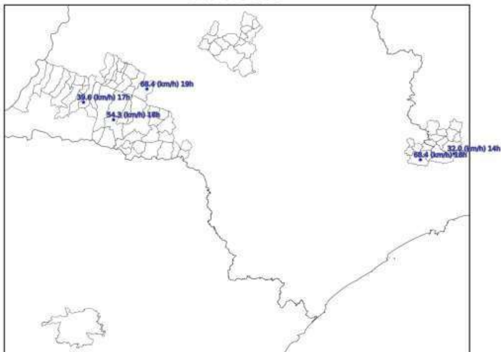
Mapa de Rajada Máxima 2021-10-03
