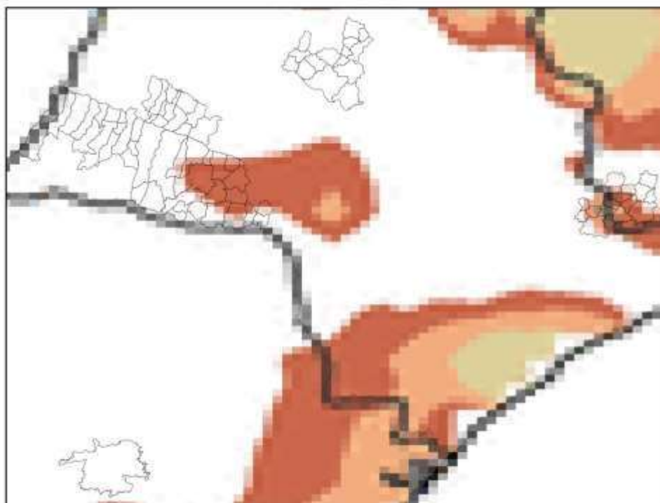
Mapa de Precipitação 2021-10-05
