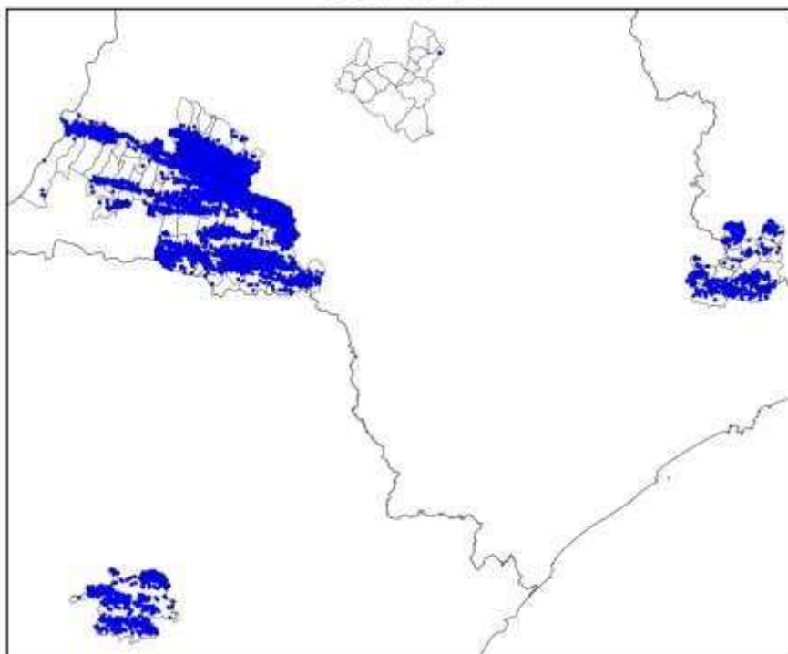
Mapa de Descargas Atmosféricas 2021-10-04
