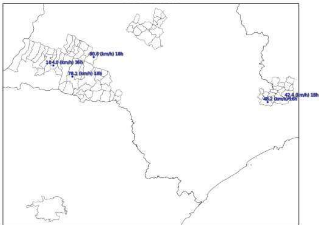
Mapa de Rajada Máxima 2021-10-01
