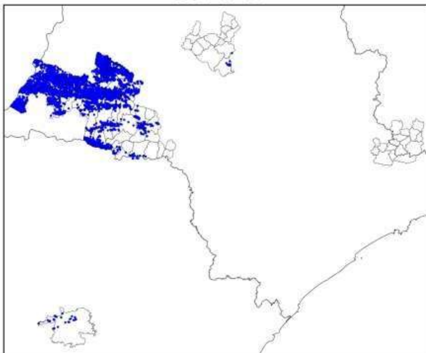
Mapa de Descargas Atmosféricas 2021-10-02
