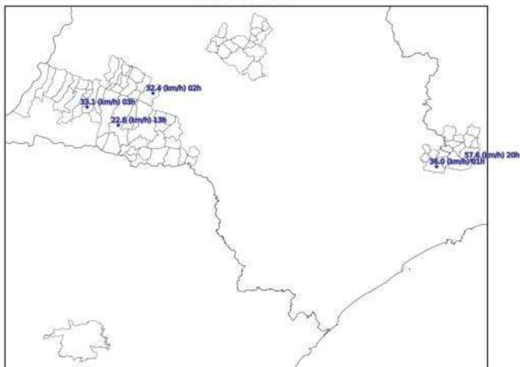
Mapa de Rajada Máxima 2021-10-06
