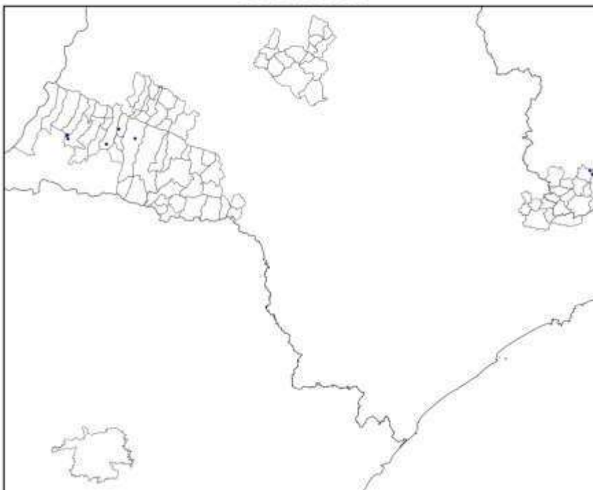
Mapa de Descargas Atmosféricas 2021-10-05
