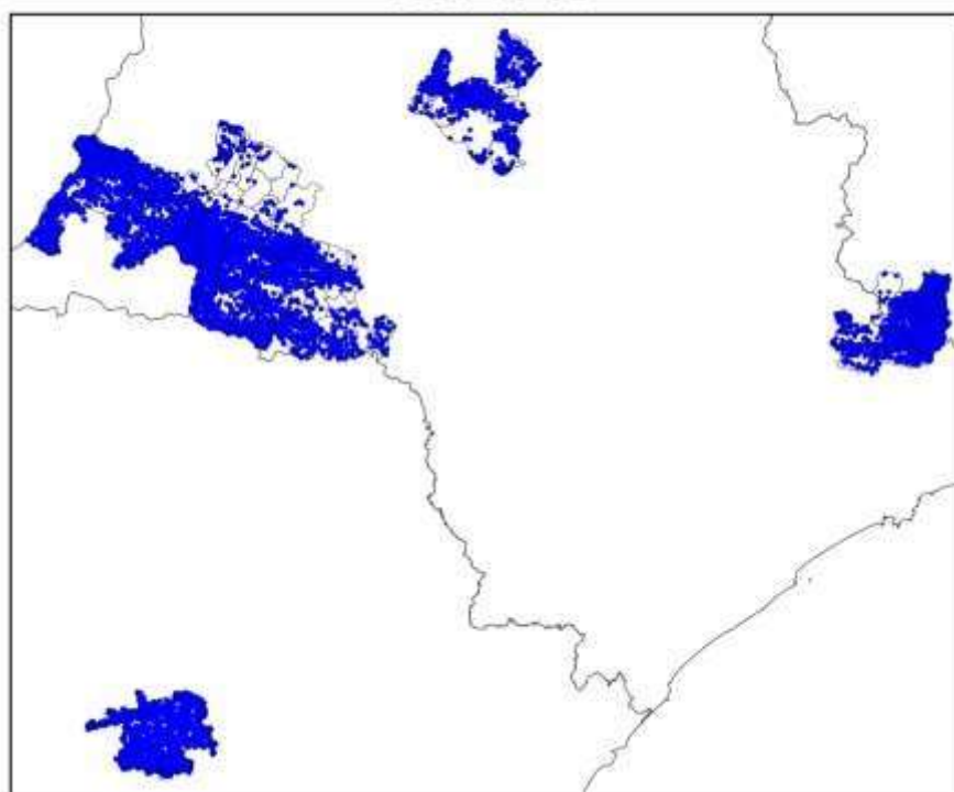
Mapa de Descargas Atmosféricas 2021-10-01
