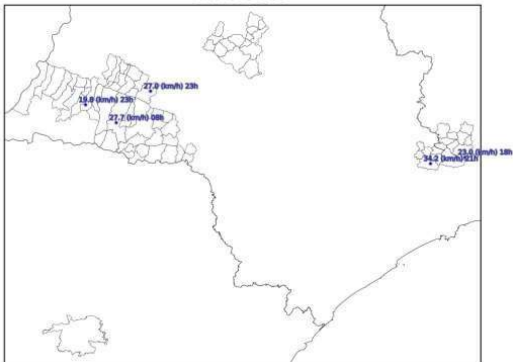
Mapa de Rajada Máxima 2021-10-05
