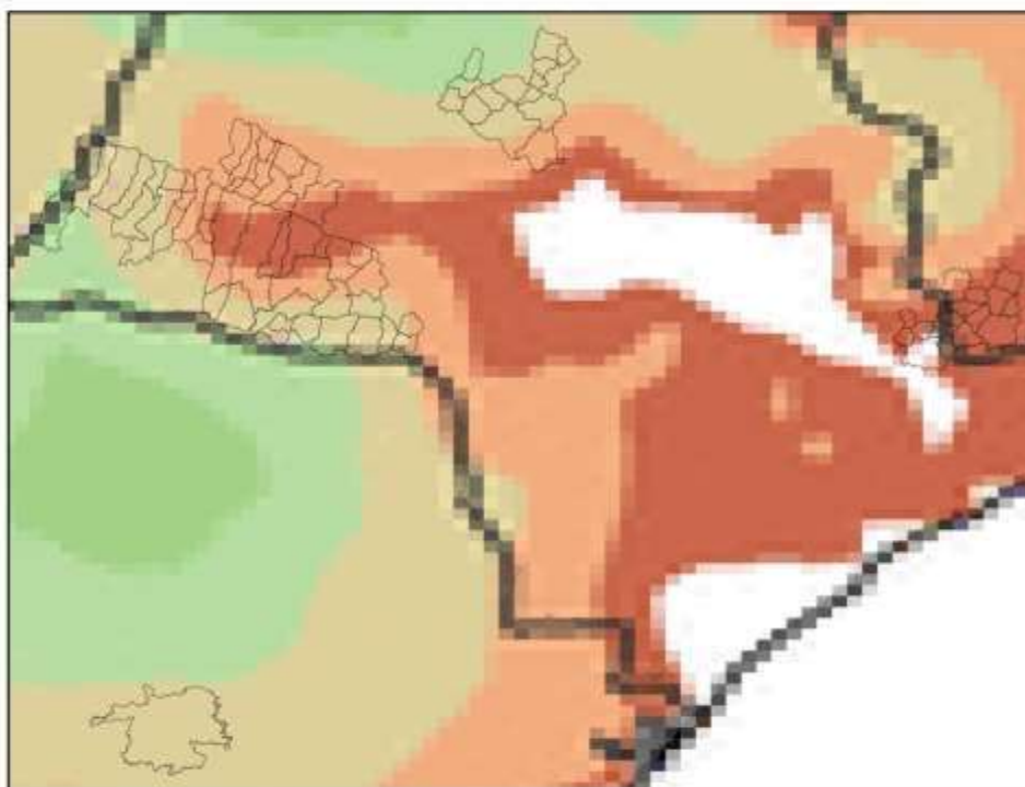
Mapa de Precipitação 2021-10-02
