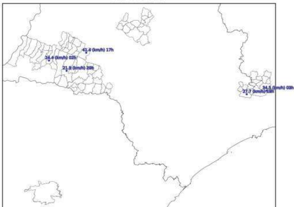
Mapa de Rajada Máxima 2021-10-04
