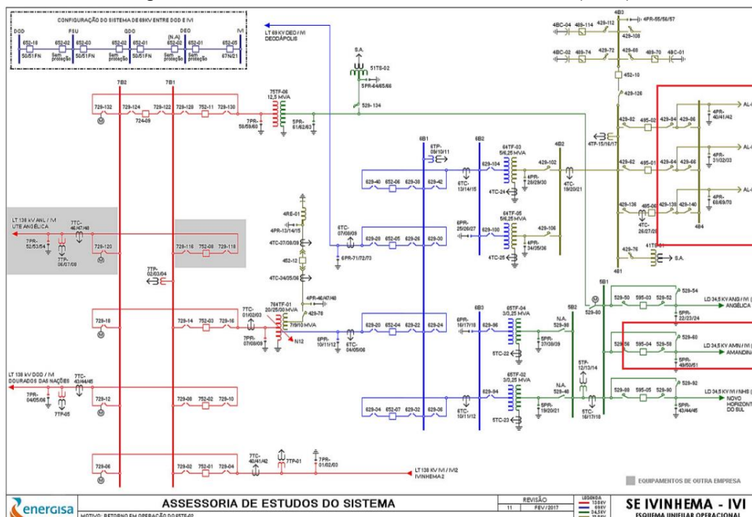
Figura 4 - Alimentadores afetados circulados em vermelho (SE IVI).
