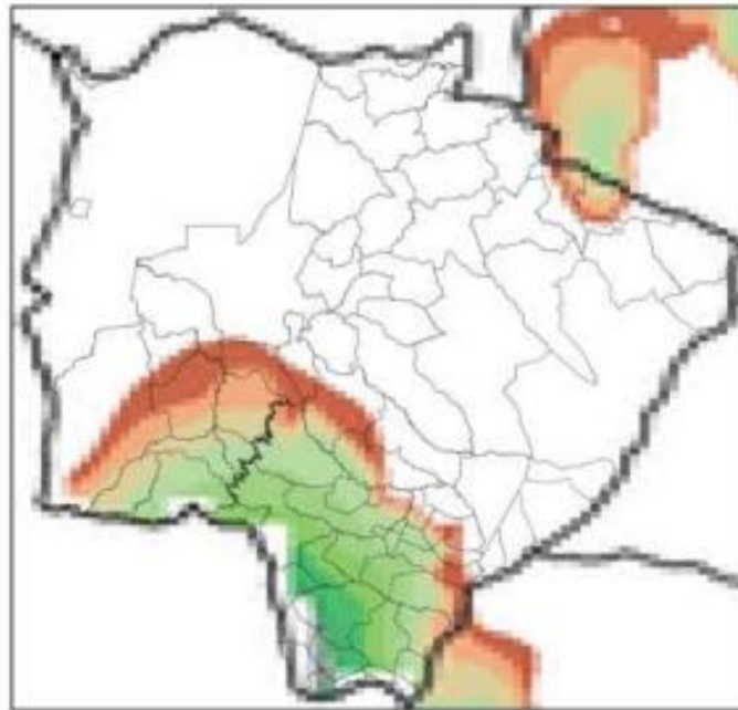
Mapa de Precipitação 2022-11-13
