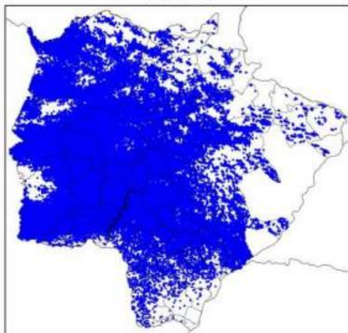
Mapa de Descargas Atmosféricas 2022-11-14
