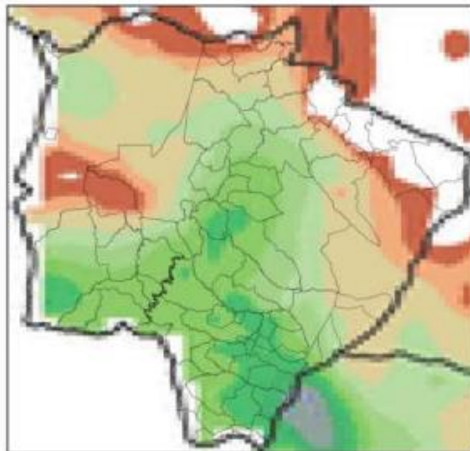
Mapa de Precipitação 2022-11-14
