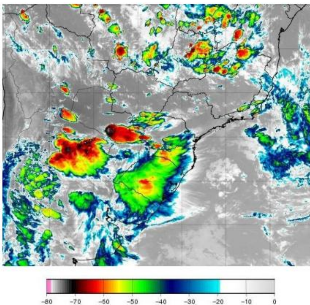
Figura 1 - Imagem de satélite no infravermelho com realce do satélite GOES-16 as 21:00 UT do dia 12/11. As cores indicam diferentes temperaturas dos topos das nuvens.
