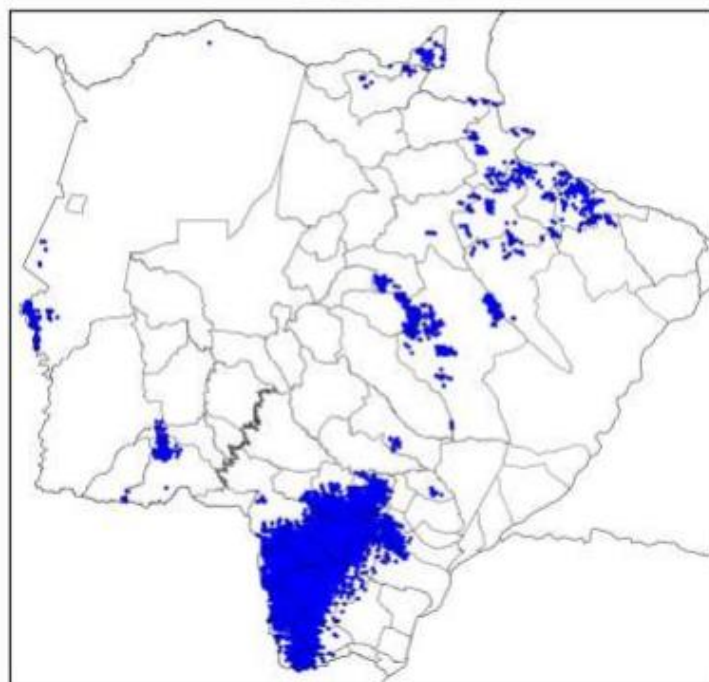
Mapa de Descargas Atmosféricas 2022-11-12
