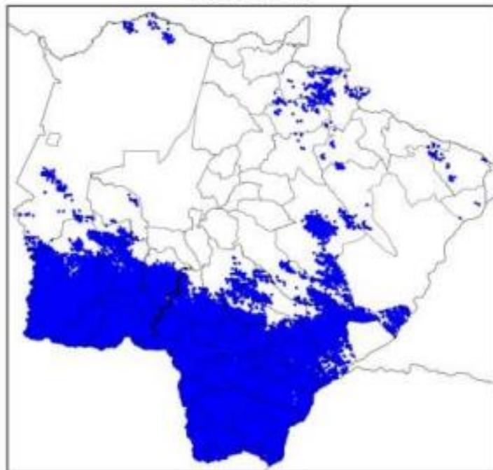
Mapa de Descargas Atmosféricas 2022-11-13
