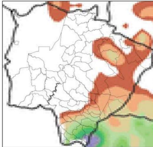
Mapa de Precipitação 2023-11-23
