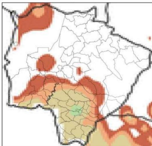
Mapa de Precipitação 2023-11-28
