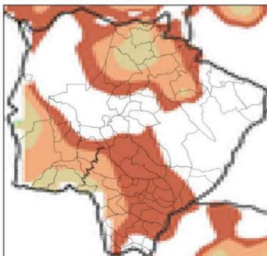
Mapa de Precipitação 2023-11-26
