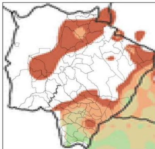
Mapa de Precipitação 2023-11-29
