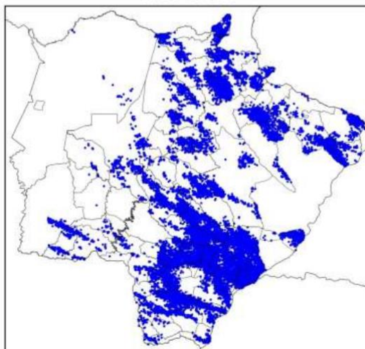
Mapa de Descargas Atmosféricas 2023-11-28
