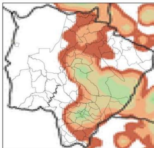
Mapa de Precipitação 2023-11-30
