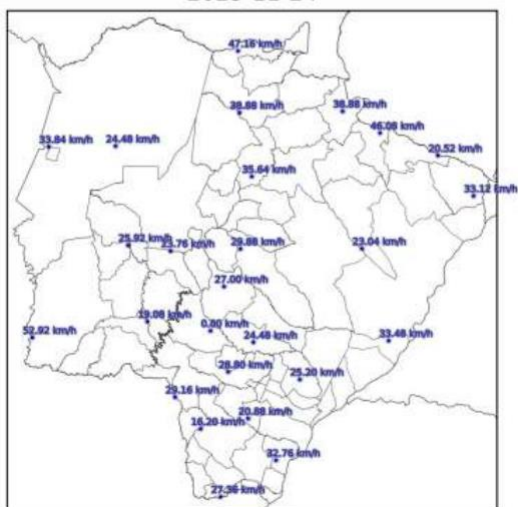
Mapa de Rajada Máxima 2023-11-24
