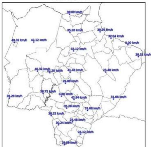
Mapa de Rajada Máxima 2023-11-27
