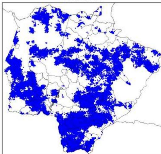
Mapa de Descargas Atmosféricas 2023-11-30
