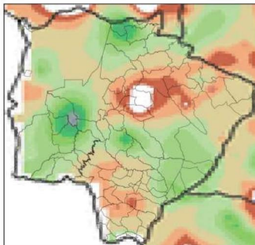
Mapa de Precipitação 2023-11-24
