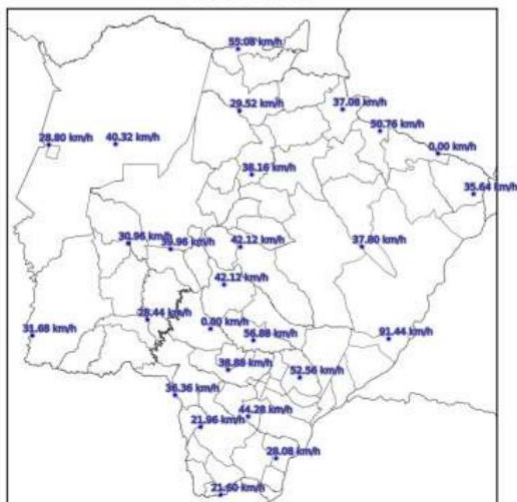
Mapa de Rajada Máxima 2023-11-28
