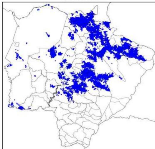
Mapa de Descargas Atmosféricas 2023-11-25
