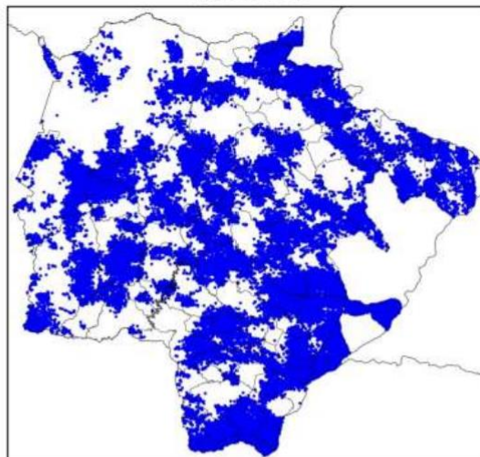
Mapa de Descargas Atmosféricas 2023-11-23
