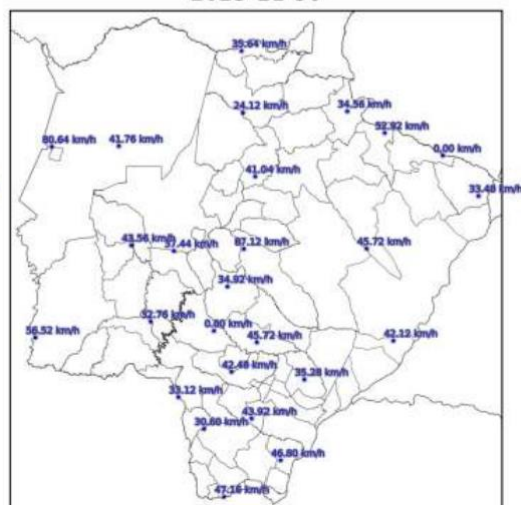
Mapa de Rajada Máxima 2023-11-30
