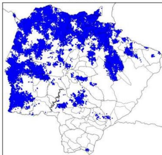
Mapa de Descargas Atmosféricas 2023-11-24
