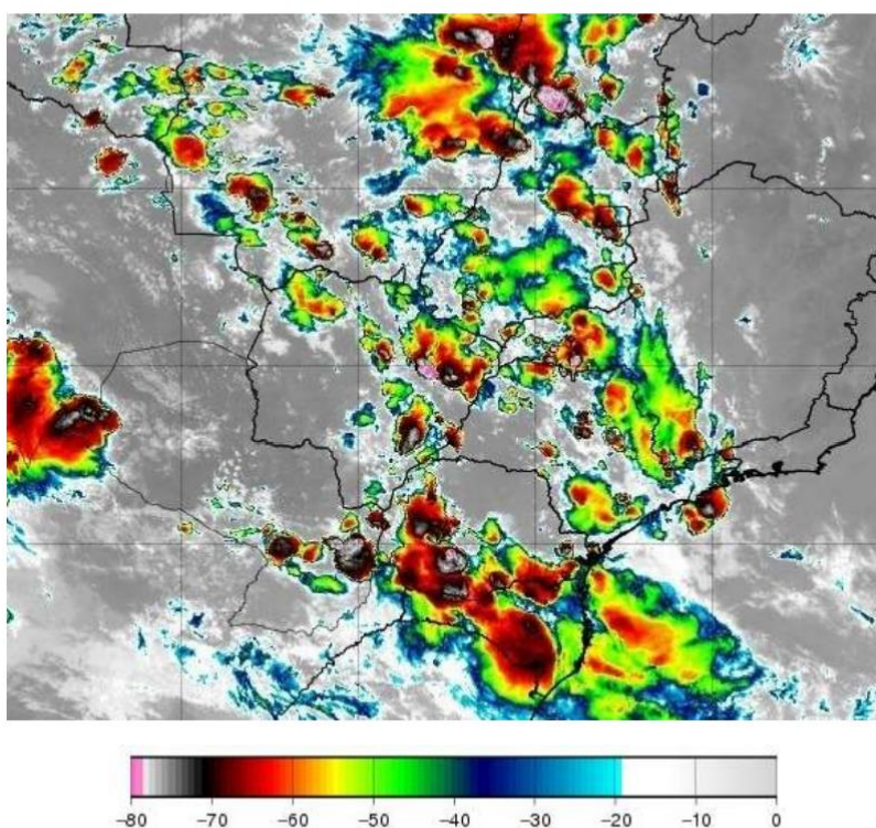
Figura 1 - Imagem de satélite no infravermelho com realce do satélite GOES-16 as 21:00 UT do dia 22/11. As cores indicam diferentes temperaturas dos topos das nuvens.
