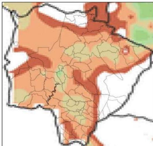
Mapa de Precipitação 2023-11-27
