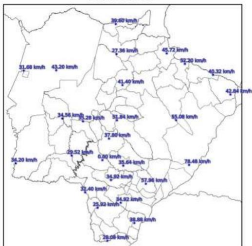
Mapa de Rajada Máxima 2023-11-23
