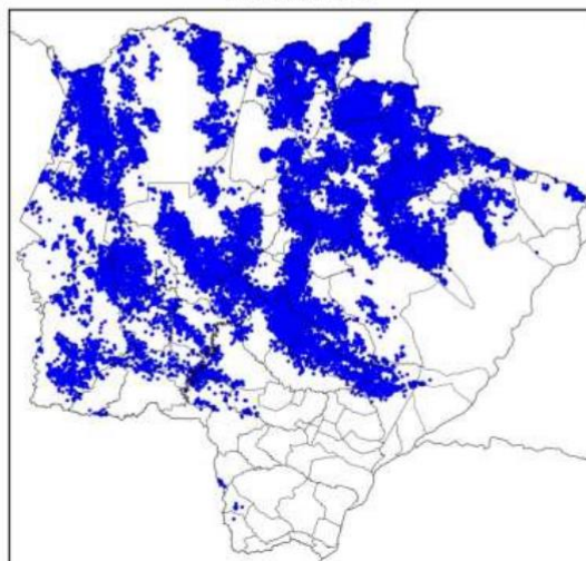
Mapa de Descargas Atmosféricas 2023-11-26
