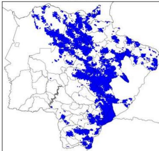
Mapa de Descargas Atmosféricas 2023-11-29
