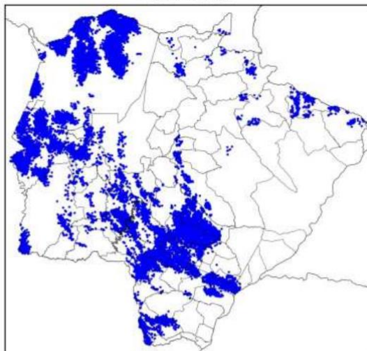
Mapa de Descargas Atmosféricas 2023-11-27
