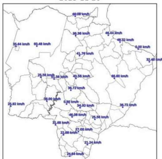
Mapa de Rajada Máxima 2023-11-26
