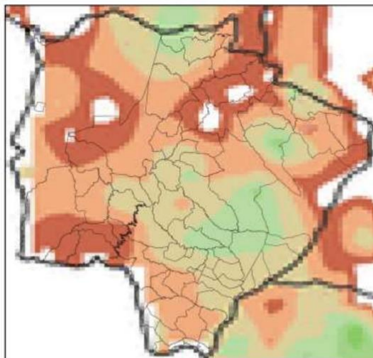
Mapa de Precipitação 2023-11-25
