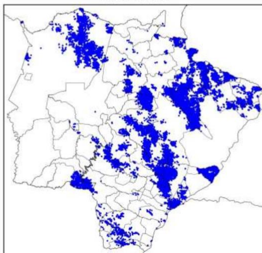
Mapa de Descargas Atmosféricas 2023-11-22
