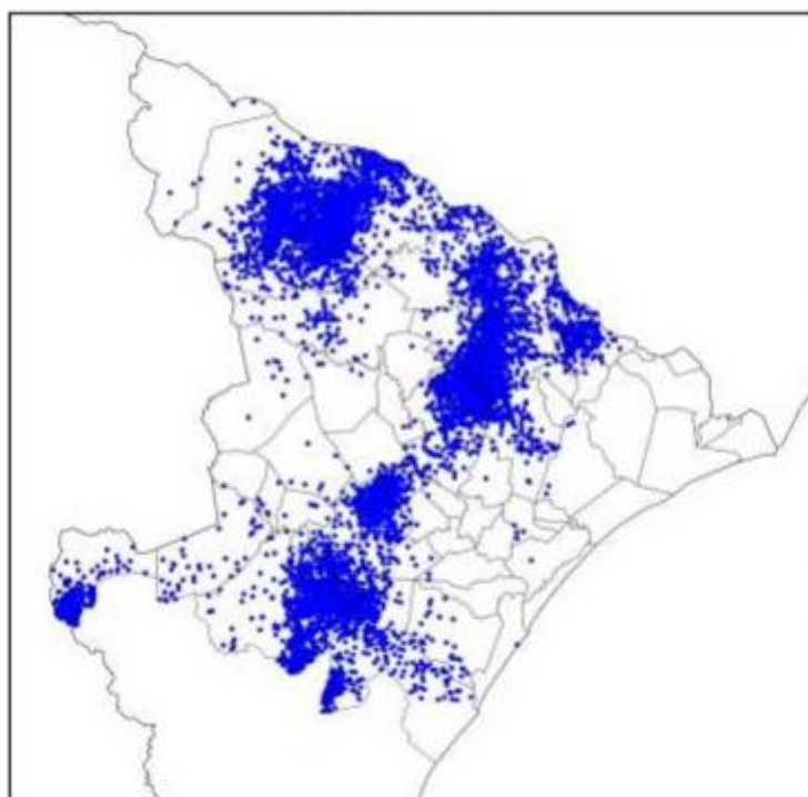
Figura 8 - Registros de descargas atmosféricas no dia 06 de novembro.
