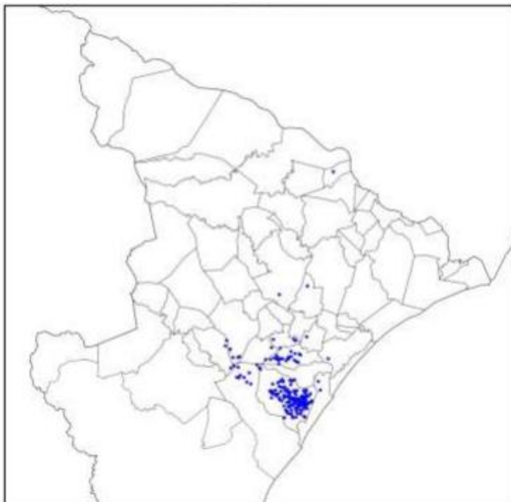
Figura 7 - Registros de descargas atmosféricas no dia 05 de novembro.
