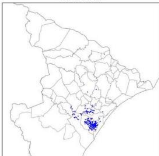
Mapa de Descargas Atmosféricas 2021-11-05
