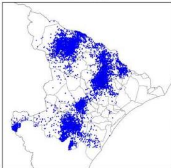
Mapa de Descargas Atmosféricas 2021-11-06
