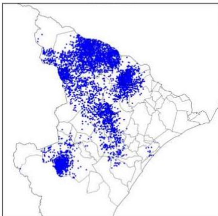
Figura 6 - Registros de descargas atmosféricas no dia 04 de novembro.
