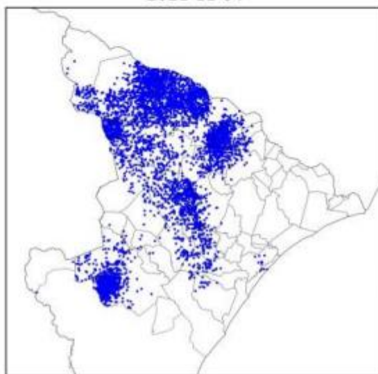
Mapa de Descargas Atmosféricas 2021-11-04
