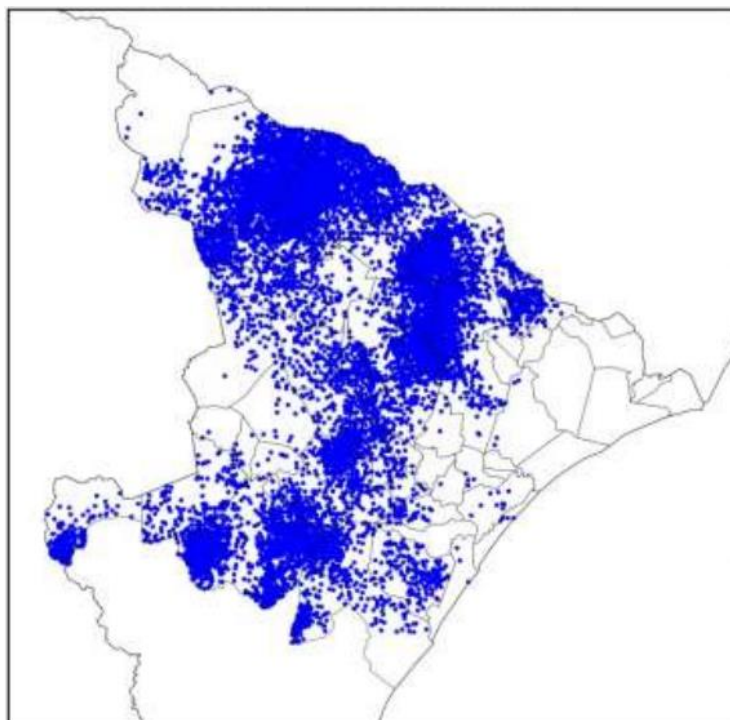
Figura 9 - Registros de descargas atmosféricas todo período (Sobreposição dos dias 4, 5 e 6 de novembro).
