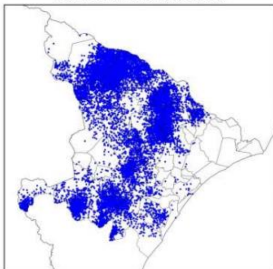
Mapa de Descargas Atmosféricas 2021-11-04 até 2021-11-06
