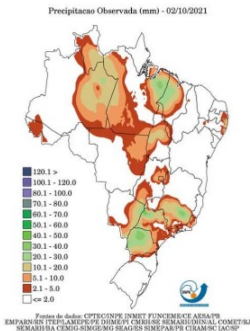
Figura 2 – Mapa de precipitação acumulada para os dias: (a) 22/09; (b) 23/09; (c) 24/09; (d) 25/09; (e) 26/09; (f) 27/09(g); 28/09; (h) 29/09; (i) 30/09; (j) 01/10; e (k) 02/10.
