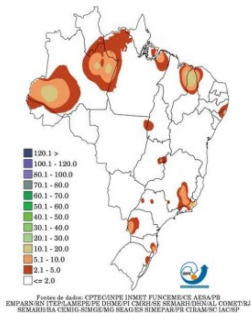
Precipitação Observada (mm) - 30/09/2021
