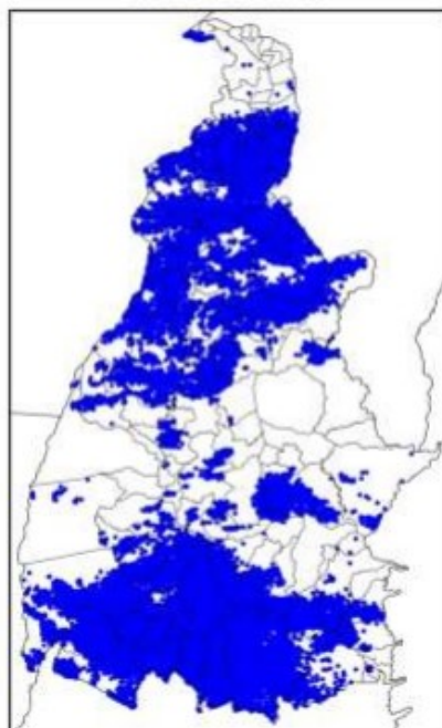
Mapa de Descargas Atmosféricas 2021-09-24
