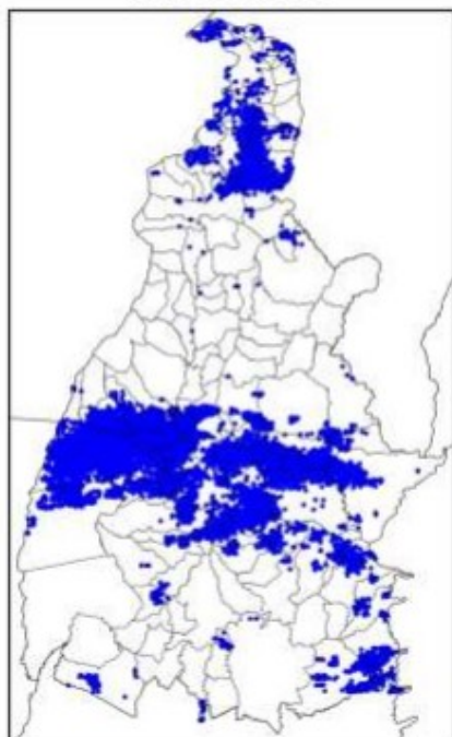
Mapa de Descargas Atmosféricas 2021-10-01
