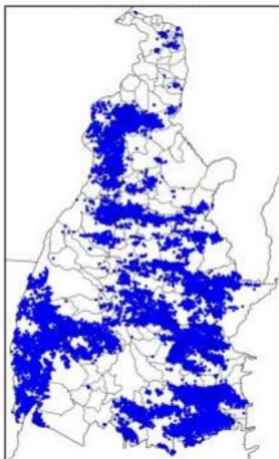
Mapa de Descargas Atmosféricas 2021-09-25
