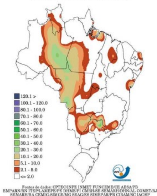
Precipitacao Observada (mm) - 27/09/2021
