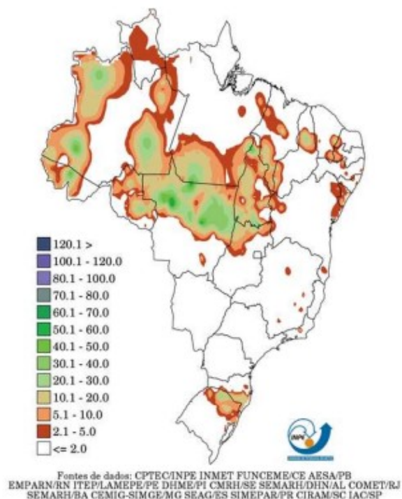
Precipitacao Observada (mm) - 24/09/2021
