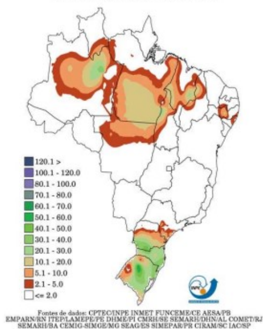
Precipitação Observada (mm) - 01/10/2021
