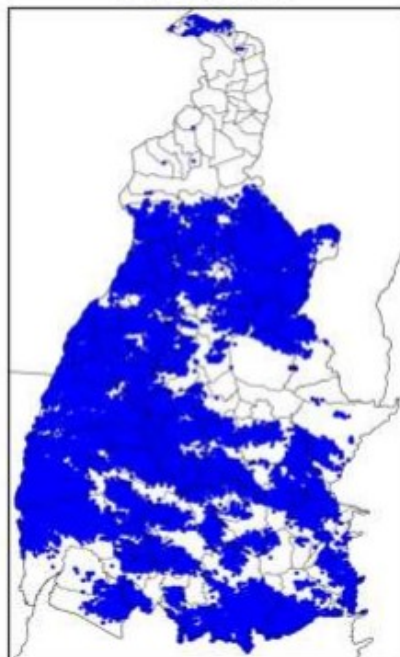
Mapa de Descargas Atmosféricas 2021-09-23
