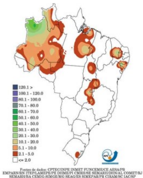
Precipitacao Observada (mm) - 25/09/2021
