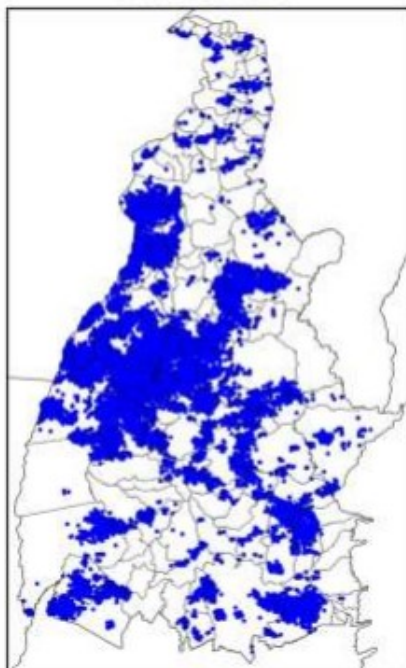
Mapa de Descargas Atmosféricas 2021-09-26
