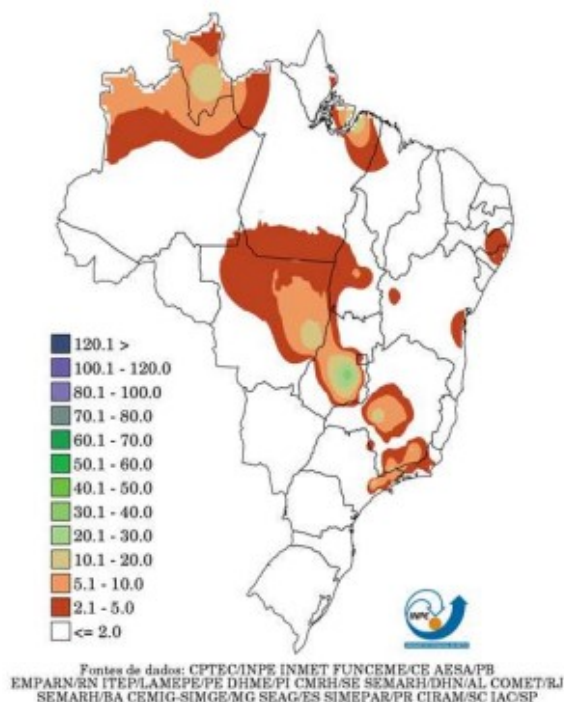
Precipitacao Observada (mm) - 26/09/2021
