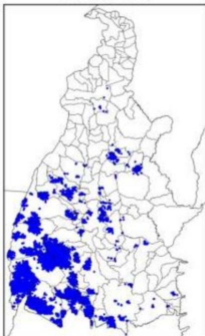
Mapa de Descargas Atmosféricas 2021-09-29
