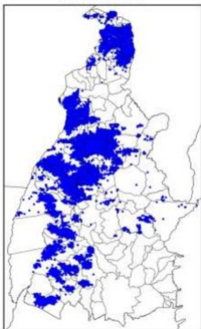
Mapa de Descargas Atmosféricas 2021-09-27
