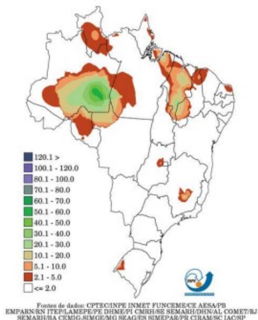
Precipitação Observada (mm) - 28/09/2021
