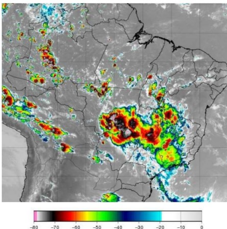
Figura 1 - Imagem de satélite no infravermelho com realce do satélite GOES-16 às 20:00 UT do dia 14/10. As cores indicam diferentes temperaturas dos tops das nuvens.
