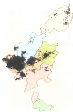
Figura 2 – Descargas Atmosféricas sobre a concessão da EMG
