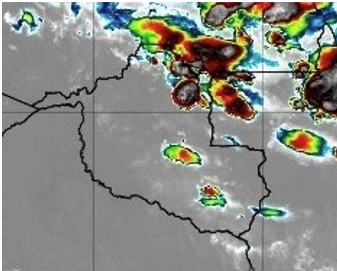
Figura 1 - Imagens de satélite no infravermelho com realce do satélite GOES-16 às 22:00 UT do dia 18/09. As cores indicam diferentes temperaturas nos topos das nuvens.
