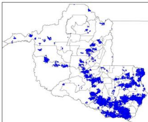
Mapa de Descargas Atmosféricas 2024-09-26
