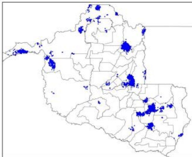
Mapa de Descargas Atmosféricas 2024-09-23
