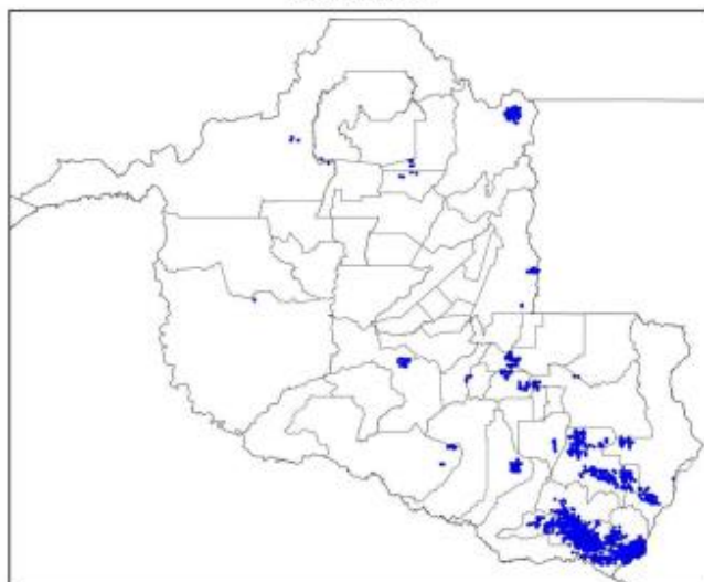
Mapa de Descargas Atmosféricas 2024-09-21
