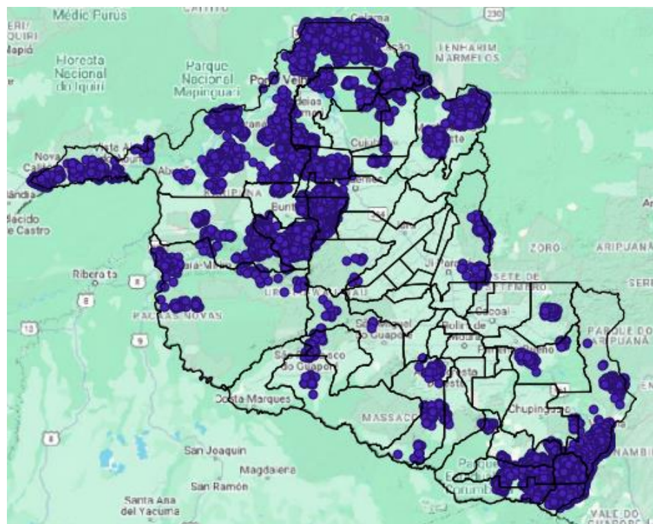
Figura 6 - Descargas Atmosféricas Observadas - 23/09/2024. Fonte: NetClima
