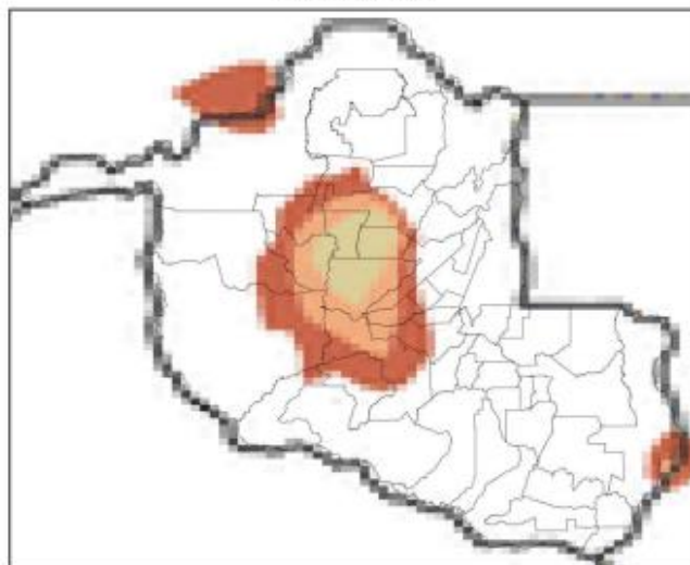
Mapa de Precipitação 2024-09-19
