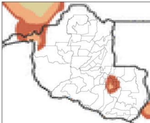
Mapa de Precipitação 2024-09-23
