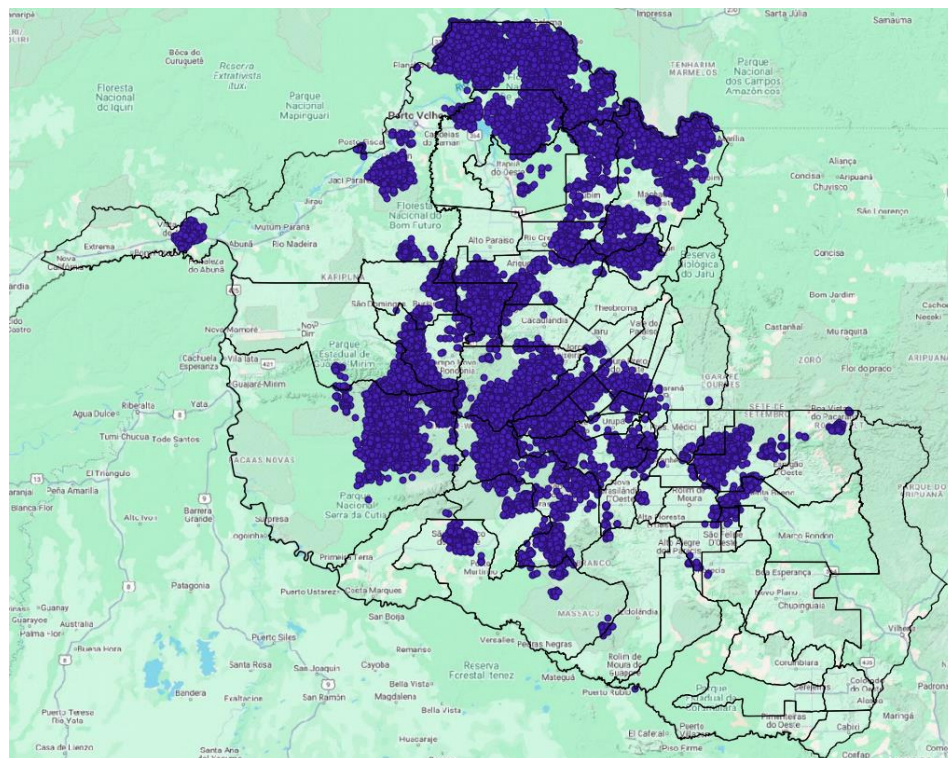
Figura 5 - Descargas Atmosféricas Observadas - 19/09/2024. Fonte: NetClima
