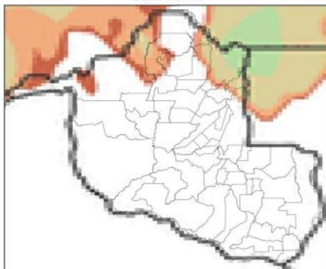
Mapa de Precipitação 2024-09-28
