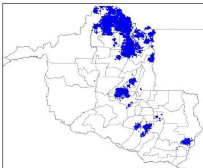
Mapa de Descargas Atmosféricas 2024-09-18
