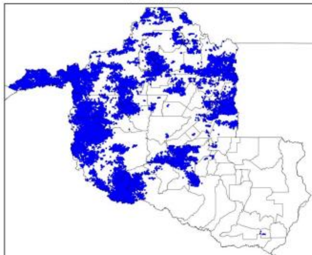
Mapa de Descargas Atmosféricas 2024-09-27
