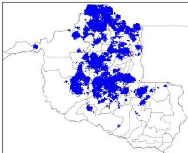
Mapa de Descargas Atmosféricas 2024-09-19
