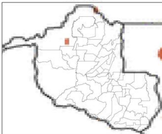
Mapa de Precipitação 2024-09-25
