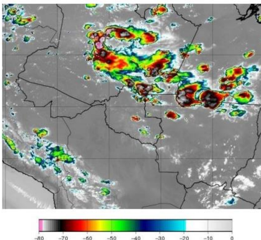
Figura 1 - Imagens de satélite no infravermelho com realce do satélite GOES-16 às 21:00 UT do dia 18/09. As cores indicam diferentes temperaturas dos topos das nuvens.
