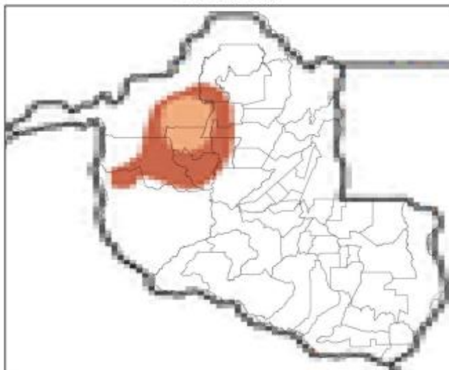
Mapa de Precipitação 2024-09-18
