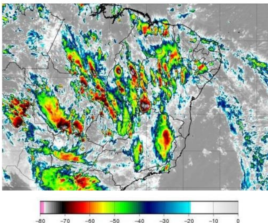
Figura 1 - Imagem de satélite no infravermelho com realce do satélite GOES-16 às 21:00 UT do dia 03/01. As cores indicam diferentes temperaturas dos topos das nuvens.
