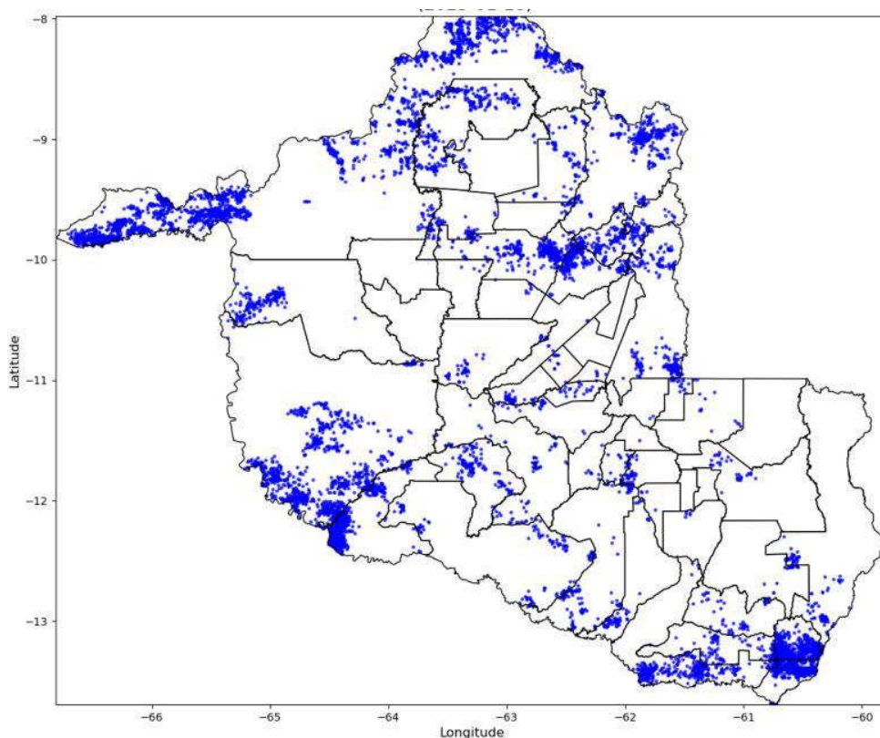
Figura 7 - Descargas Atmosféricas Observadas - 18/01/2025. Fonte: Grupo STORM
