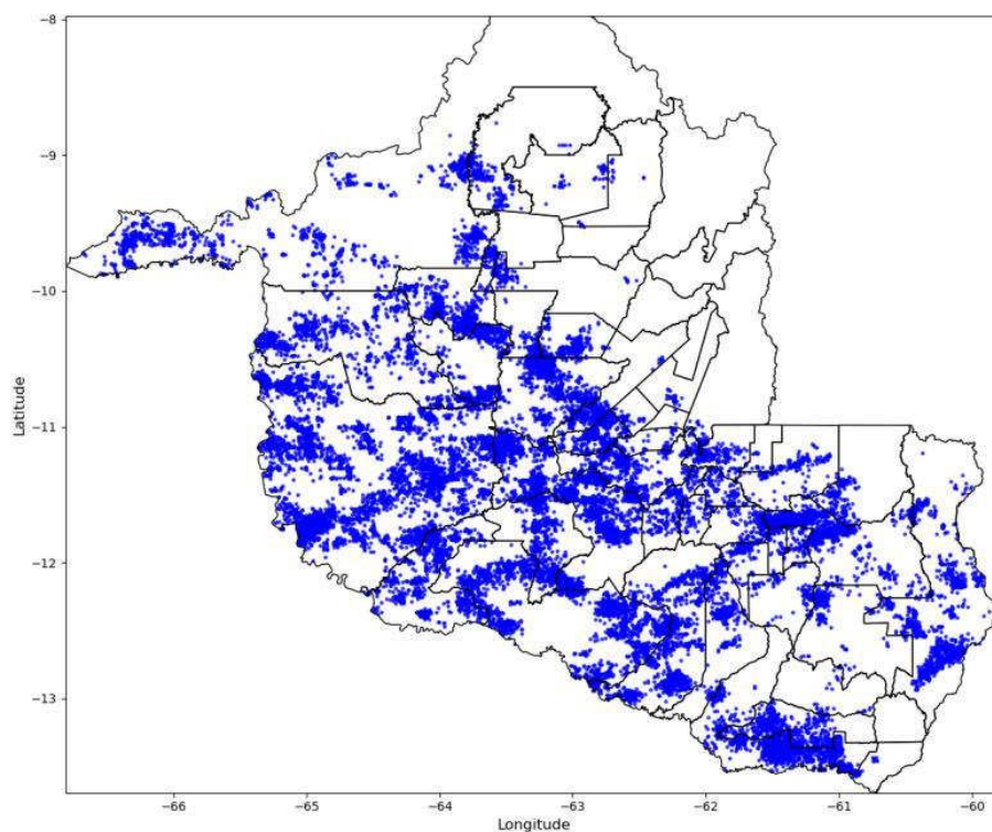
Figura 6 - Descargas Atmosféricas Observadas - 17/01/2025. Fonte: Grupo STORM
