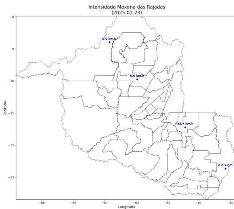
Figura 4 – Mapas de rajadas para os dias entre 15 e 23/01.
