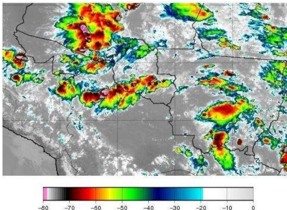
Figura 1 - Imagens de satélite no infravermelho com realce do satélite GOES-16 às 21:00 UT do dia 15/01. As cores indicam diferentes temperaturas dos topos das nuvens.
