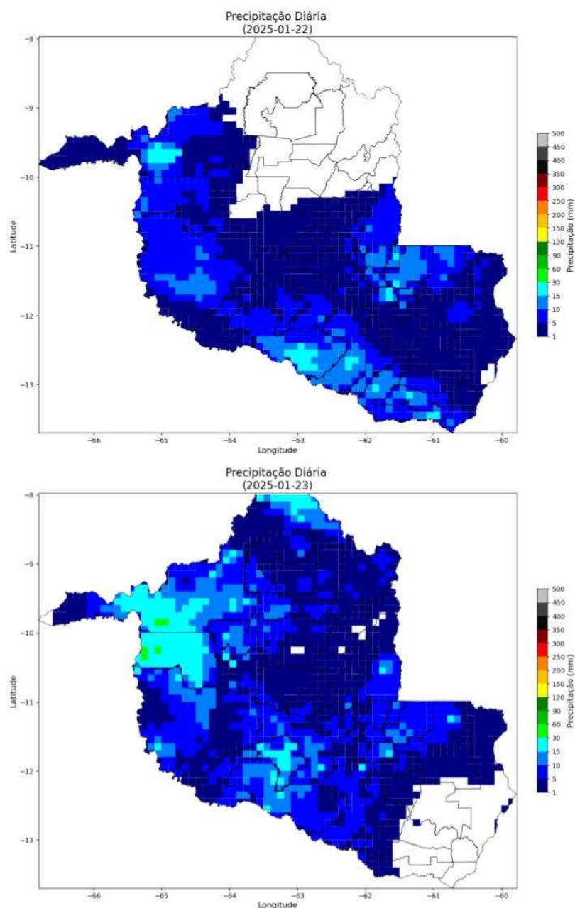
Figura 3 – Mapas de precipitação para os dias entre 15 e 23/01.
