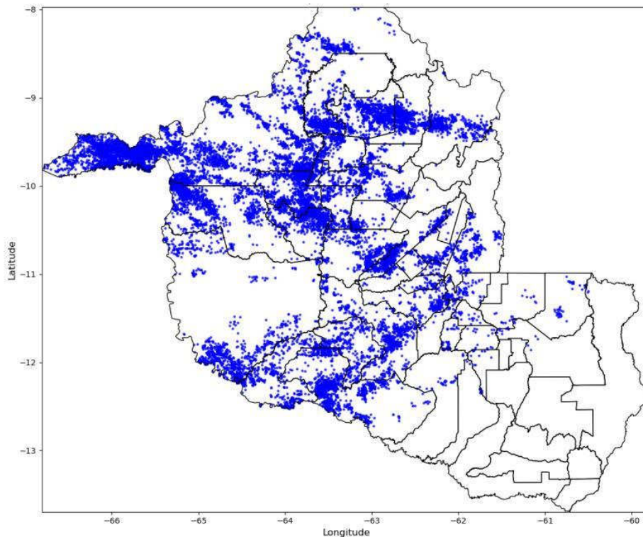
Figura 4 - Descargas Atmosféricas Observadas - 15/01/2025. Fonte: Grupo STORM
