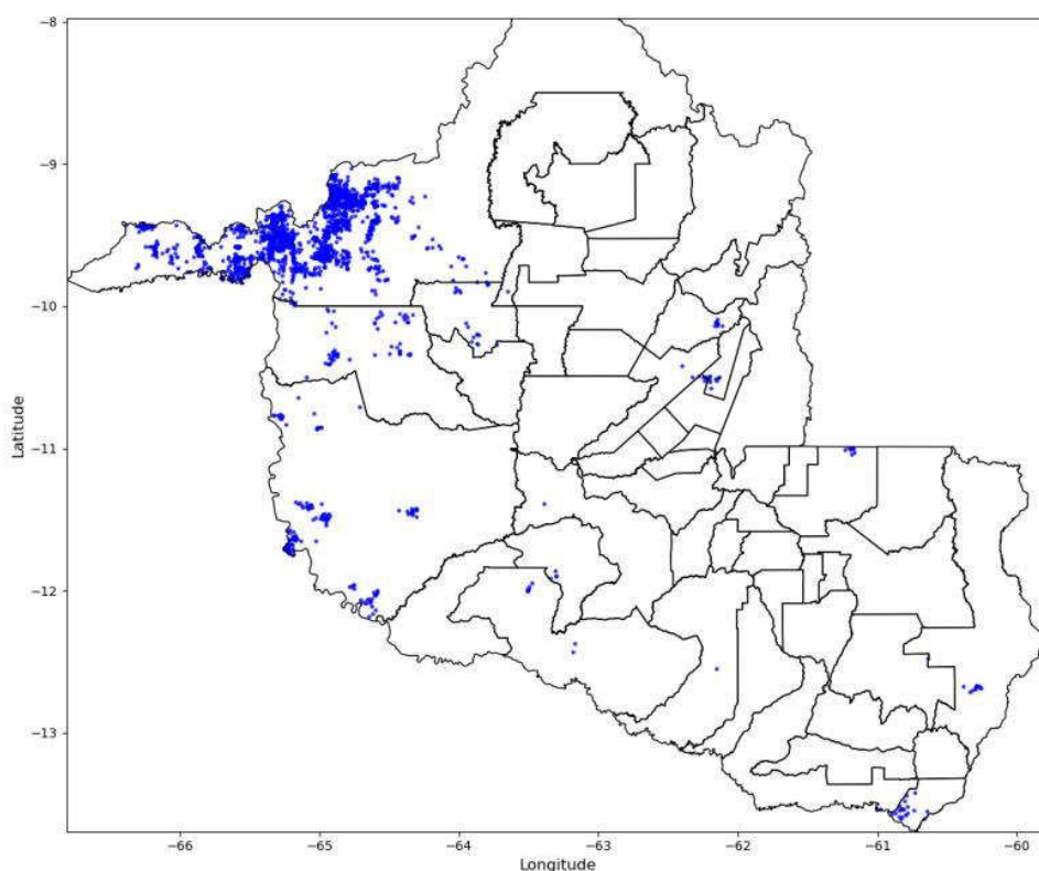
Figura 8 - Descargas Atmosféricas Observadas - 19/01/2025. Fonte: Grupo STORM
