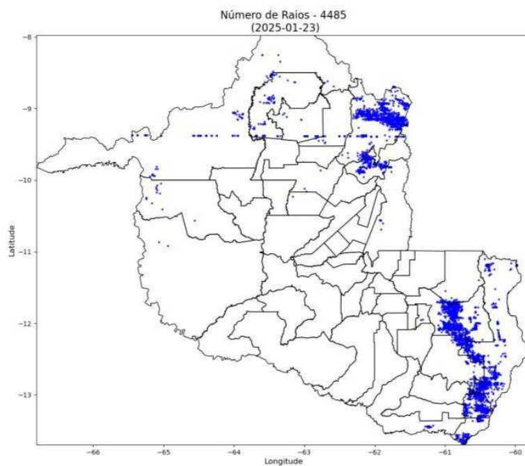
Figura 2 – Mapas de descargas atmosféricas para os dias entre 15 e 23/01.
