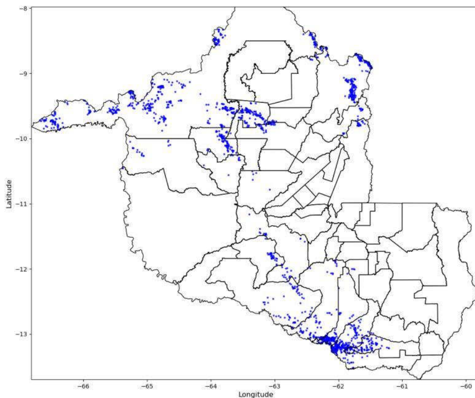
Figura 10 - Descargas Atmosféricas Observadas - 21/01/2025. Fonte: Grupo STORM
