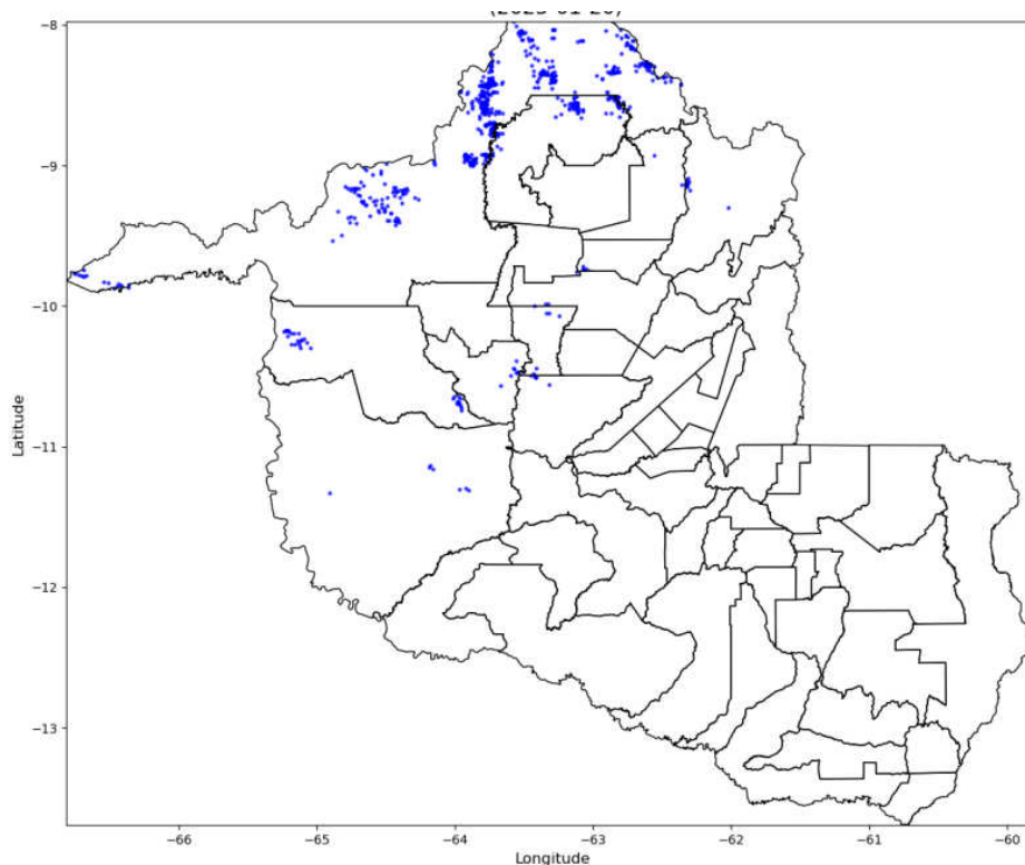
Figura 9 - Descargas Atmosféricas Observadas - 20/01/2025. Fonte: Grupo STORM
