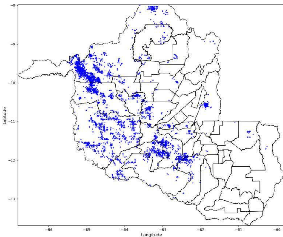
Figura 11 - Descargas Atmosféricas Observadas - 22/01/2025. Fonte: Grupo STORM
