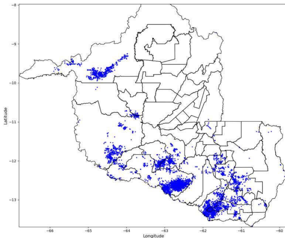
Figura 5 - Descargas Atmosféricas Observadas - 16/01/2025. Fonte: Grupo STORM
