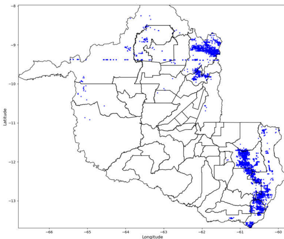
Figura 12 - Descargas Atmosféricas Observadas - 23/01/2025. Fonte: Grupo STORM
