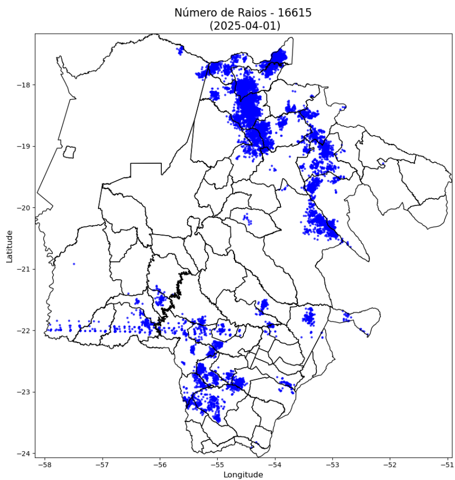
Figura 2 – Mapa de incidência de descargas atmosféricas nuvem-solo e intranuvem para os dias 22/03 a 01/04.
