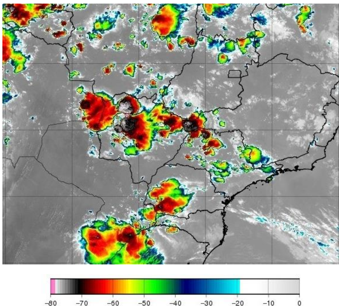
Figura 1 - Imagem de satélite no infravermelho com realce do satélite GOES-16 as 21:00 UT do dia 22/03. As cores indicam diferentes temperaturas dos topos das nuvens.
