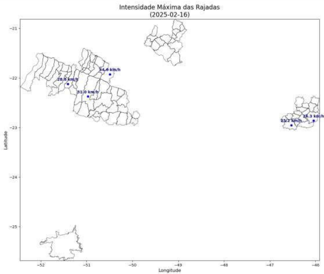
Figura 4 – Mapa de máximas rajadas para os dias de 06 a 16/02.
