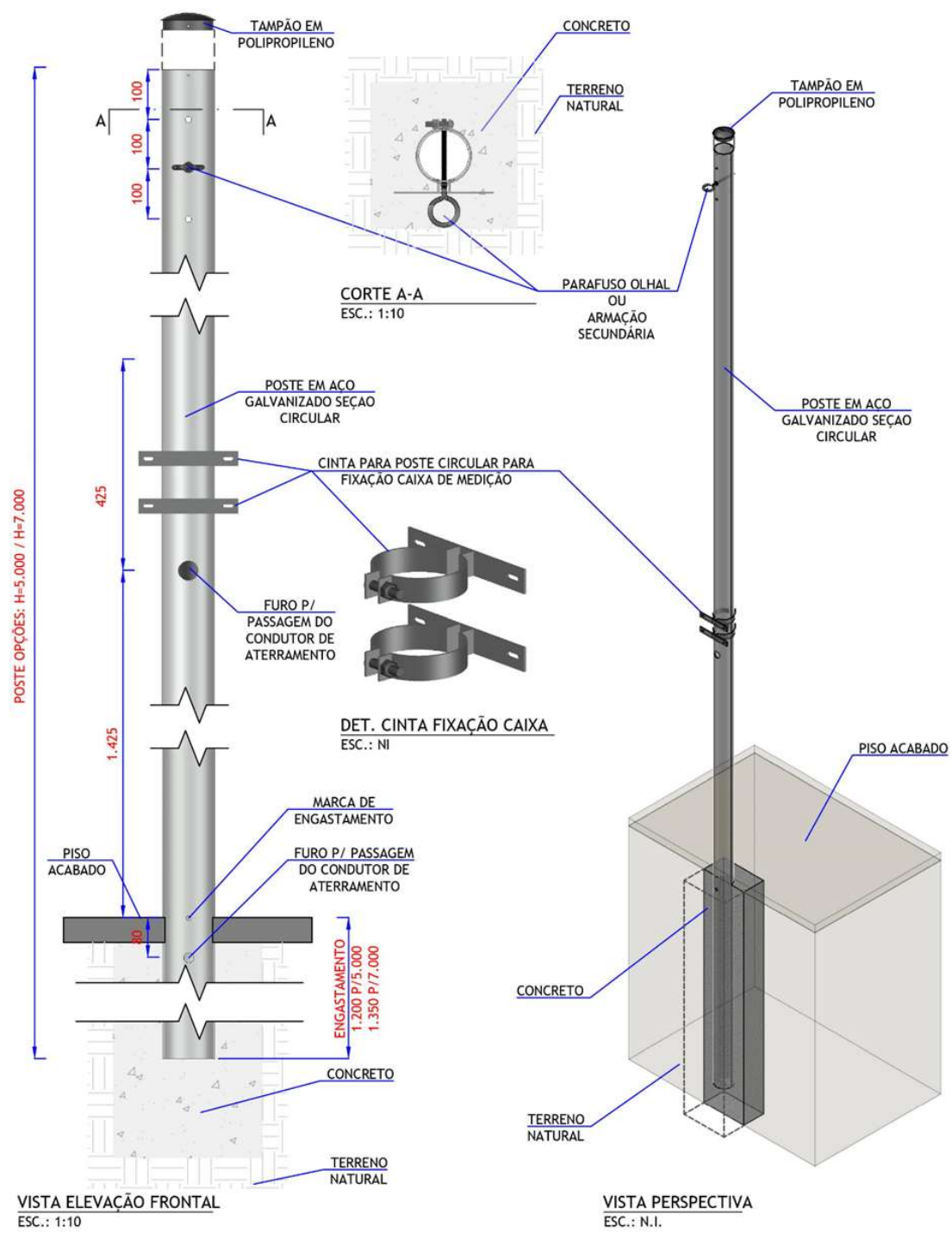
DESENHO 29 - Poste auxiliar em aço galvanizado (seção circular)
