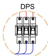
DETALHE A
