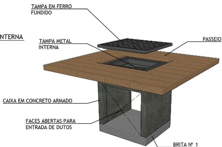
VISTA EM PERSPECTIVA ESC.: N.I.
