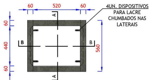
VISTA EM PLANTA - CAIXA EM CONCRETO ESC.: 1/20
