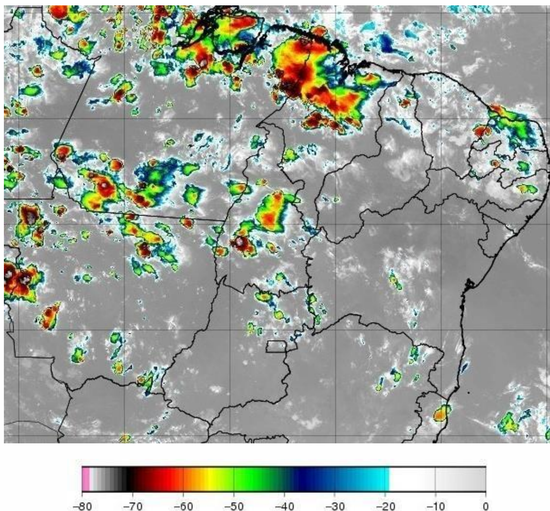
Figura 1 - Imagem de satélite no infravermelho com realce do satélite GOES-19 às 21:00 UT do dia 20/04. As cores indicam diferentes temperaturas dos topos das nuvens.
