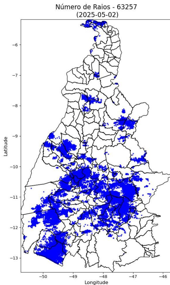
Figura 2 – Mapa de descargas atmosféricas para os dias 20/04 a 02/05.
