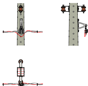
SI1 - FOLHA 03/13
