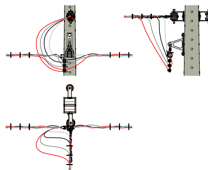
SI1-SI3 - FOLHA 10/21
