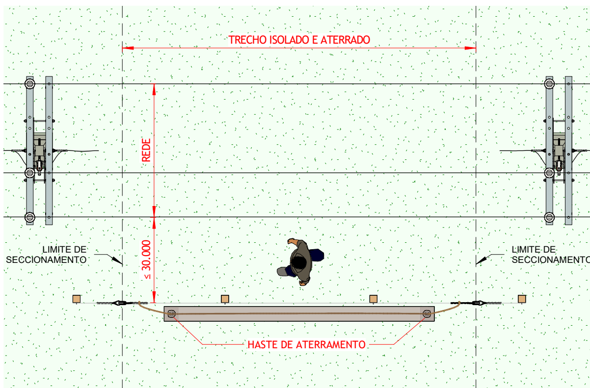
VISTA SUPERIOR
