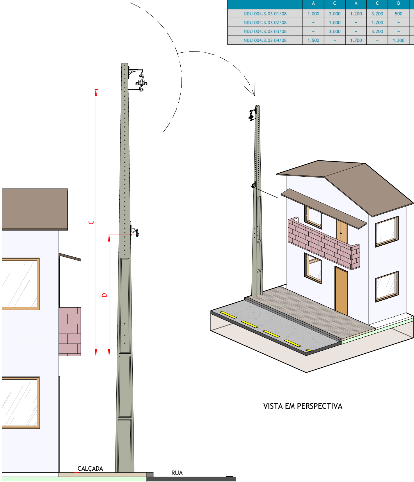
VISTA LATERAL
