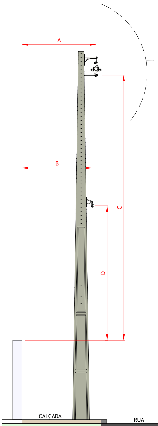
VISTA LATERAL 1 : 50
