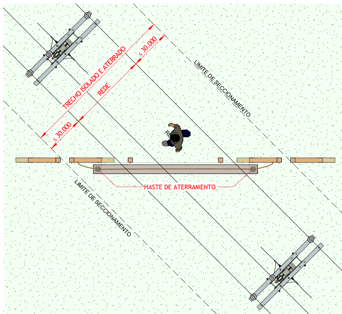
VISTA SUPERIOR
