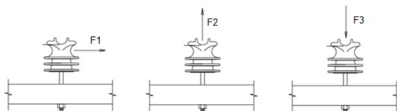
Figura 2 - Detalhe para execução do ensaio
