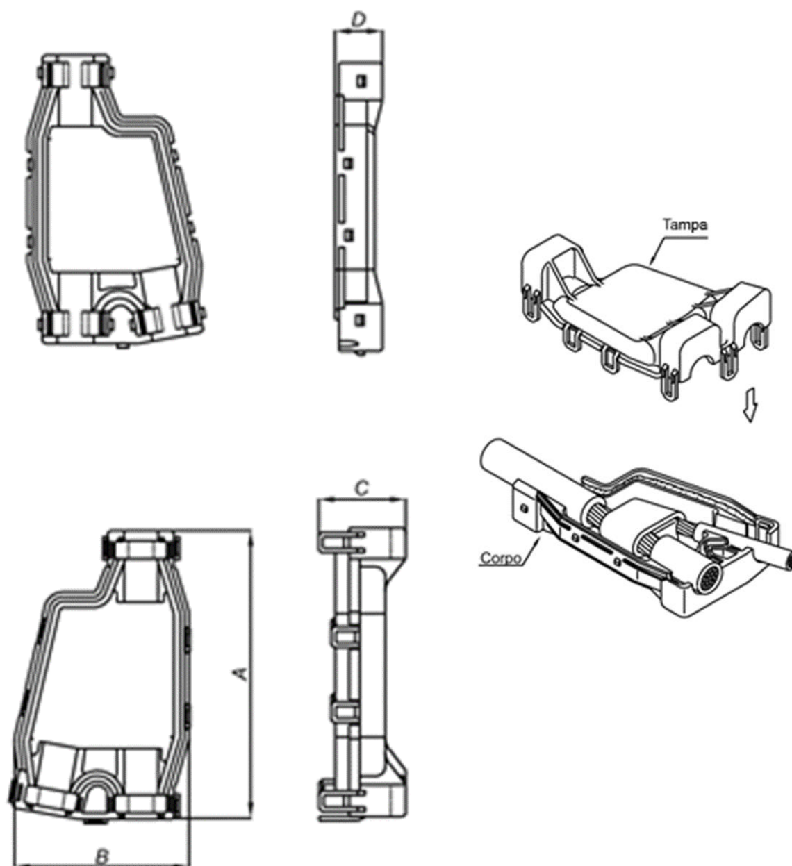
DESENHO 1 - Característica dimensional da capa protetora para conectores de derivação
