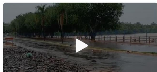
Figura 4 – Evidências de tempestades no período no estado do Mato Grosso do Sul [4].
