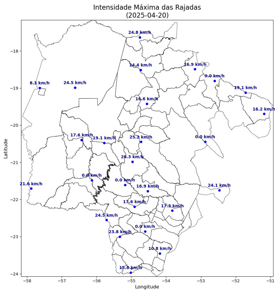
Figura 4 – Mapa de rajadas para os dias 12 a 20/04.
