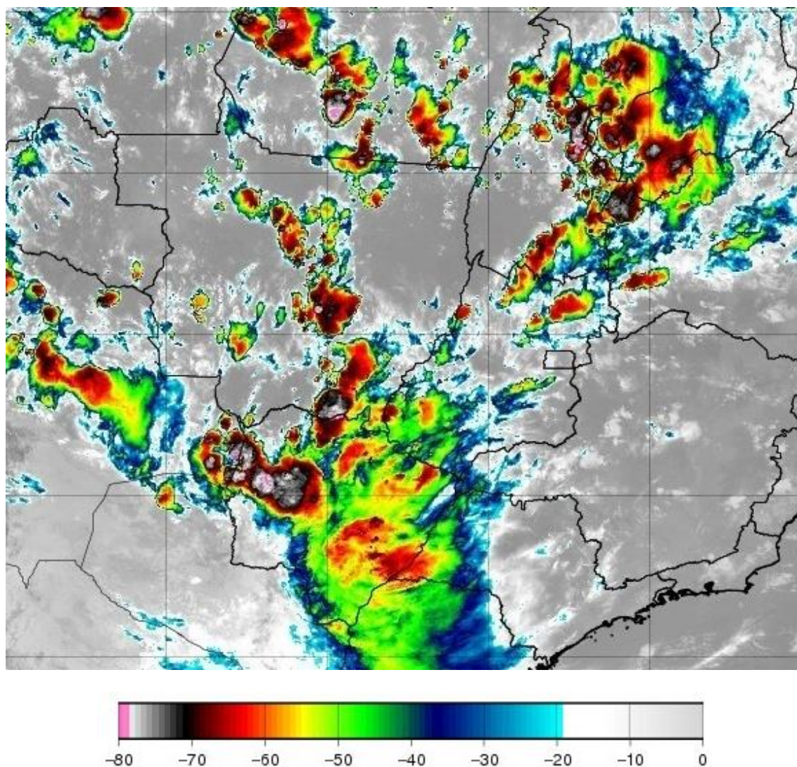
Figura 1 - Imagem de satélite no infravermelho com realce do satélite GOES-19 as 21:00 UT do dia 12/04. As cores indicam diferentes temperaturas dos topos das nuvens.
