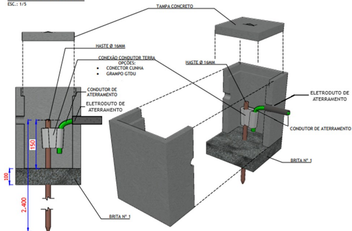
VISTA EM CORTE A-A - SEM TAMPA ESC.: 1/5
