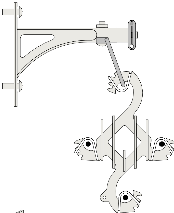
VISTA LATERAL
