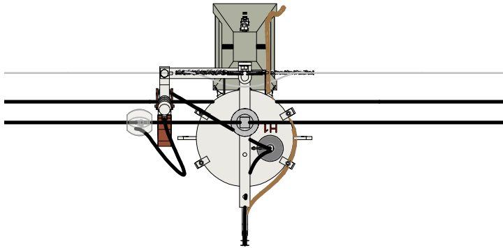
VISTA SUPERIOR 1 : 25
