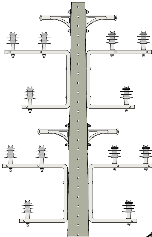
VISTA LATERAL 1 : 20
