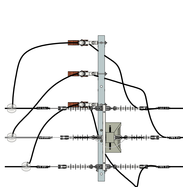
VISTA SUPERIOR
