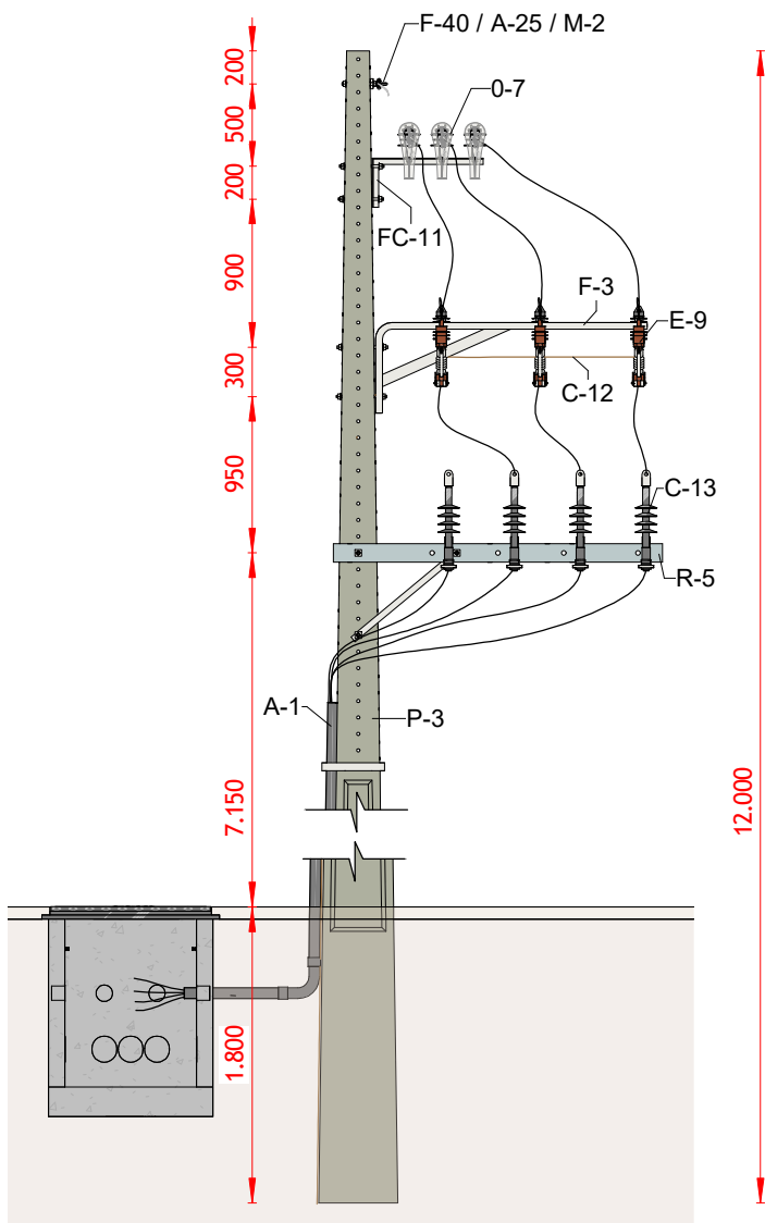
VISTA LATERAL
