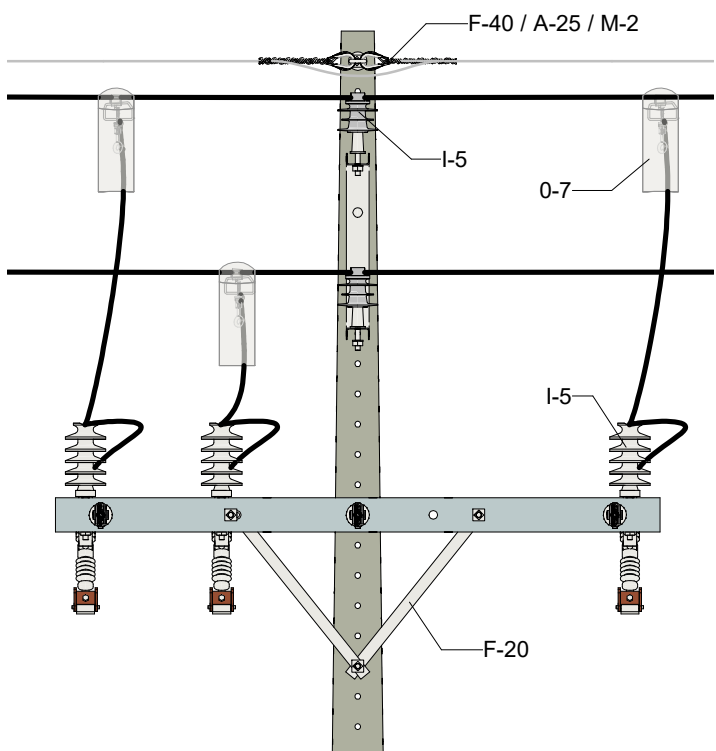
VISTA LATERAL
