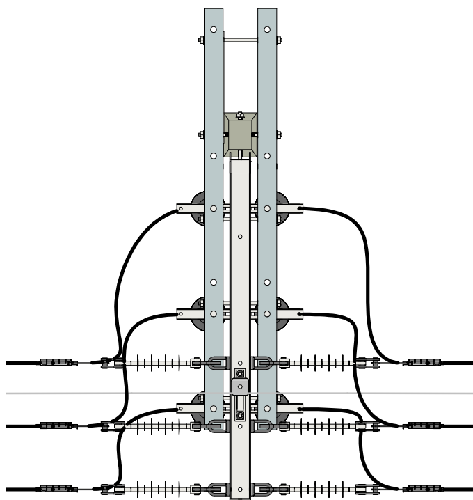
VISTA SUPERIOR
