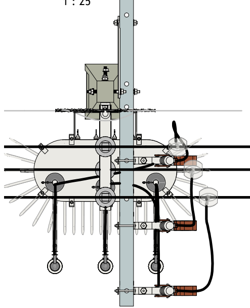
VISTA SUPERIOR 1 : 25
