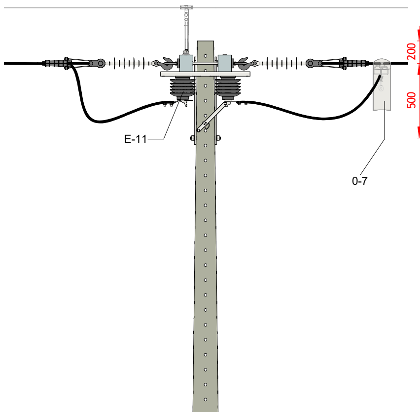
VISTA FRONTAL 1 : 25
