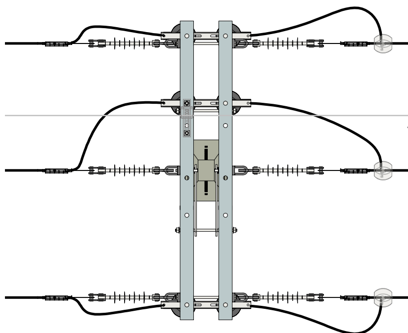
VISTA SUPERIOR 1 : 25
