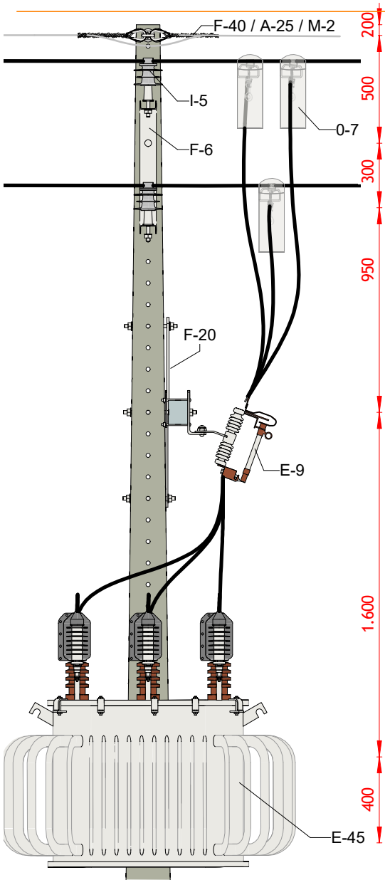
VISTA FRONTAL 1 : 25
