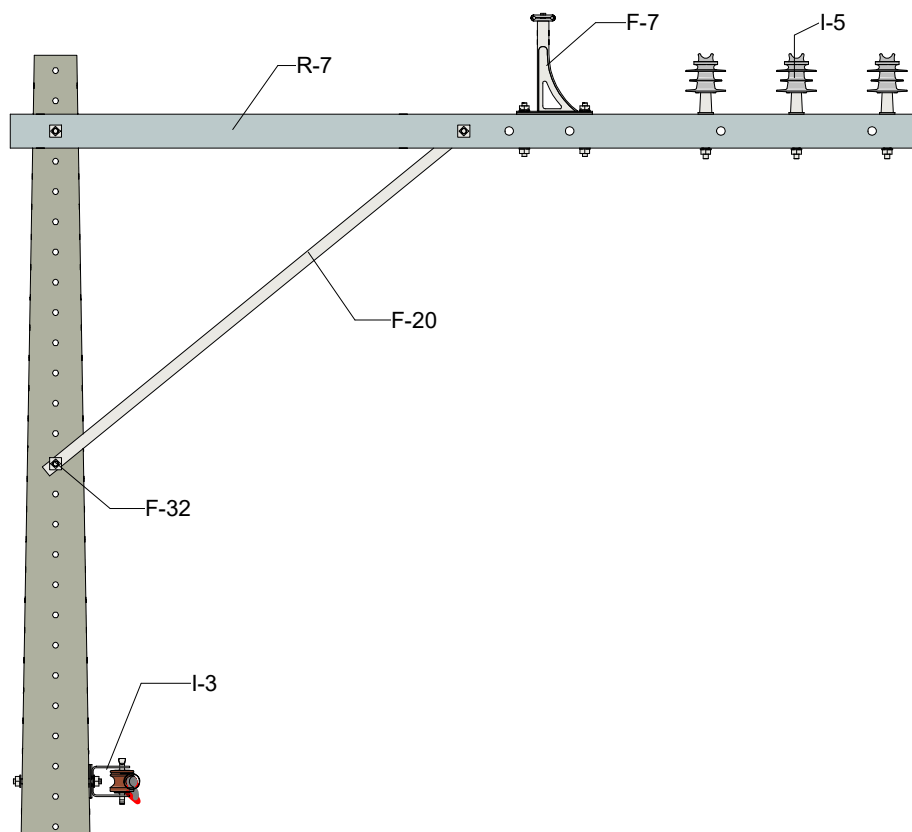
VISTA LATERAL 1 : 25
