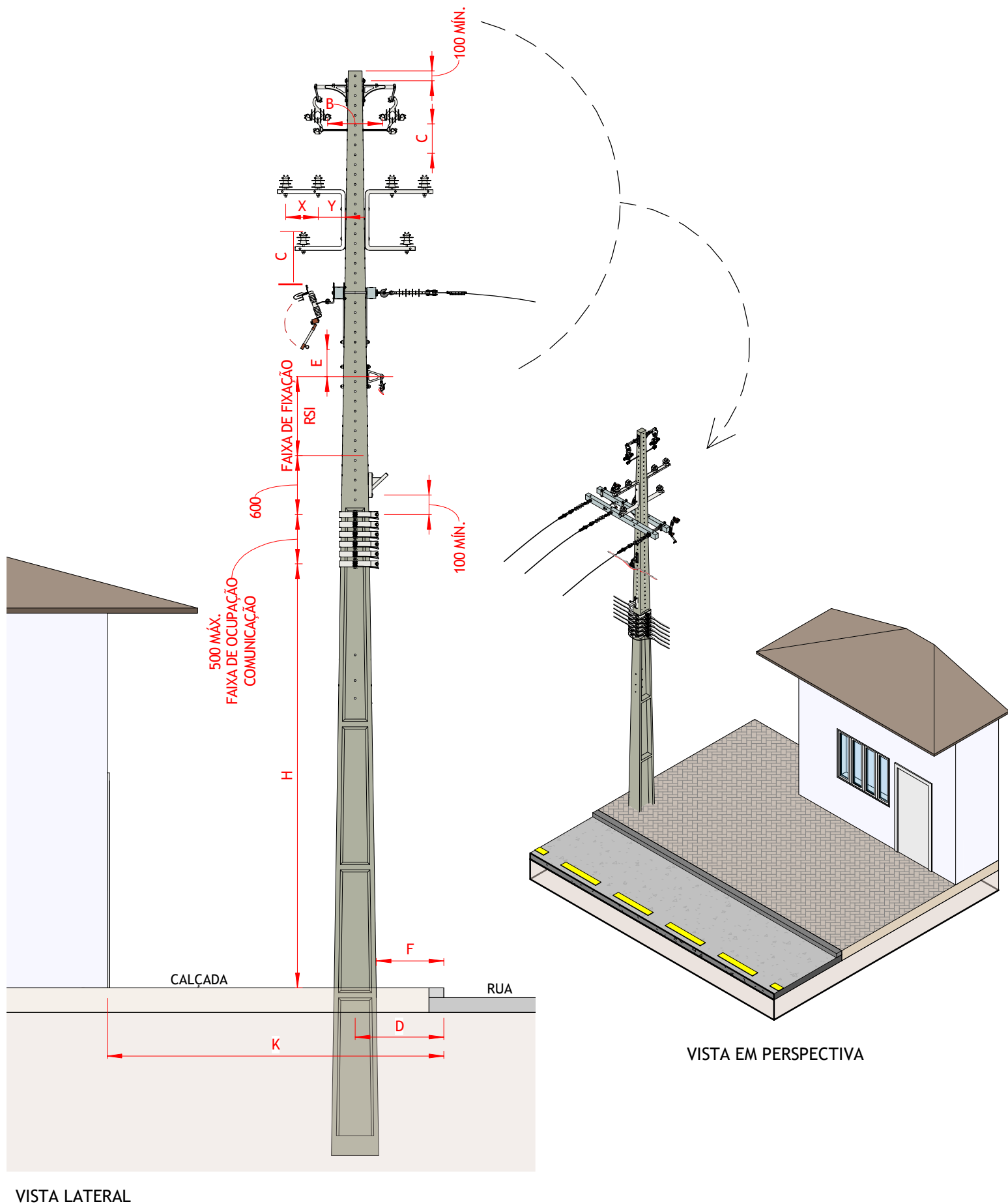
VISTA LATERAL
