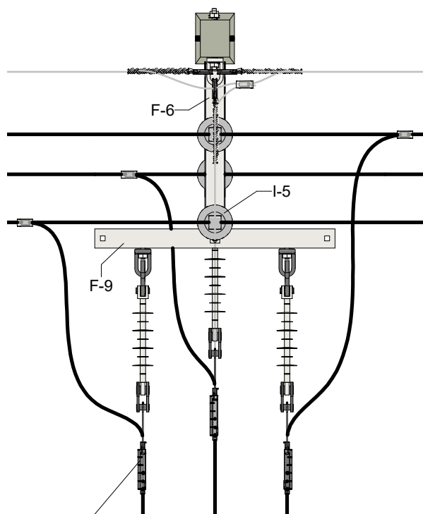
VISTA SUPERIOR
