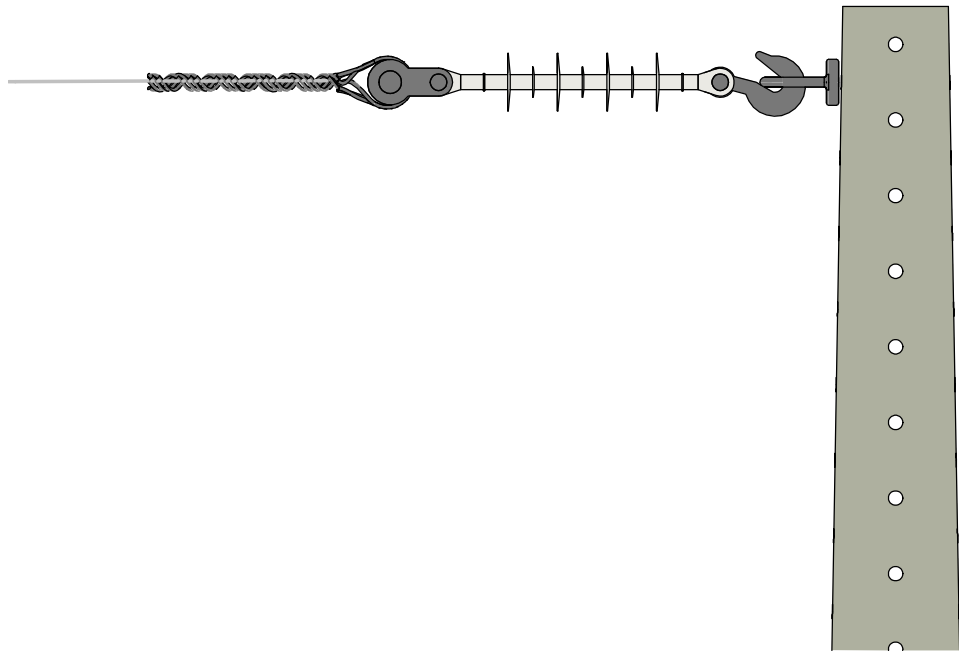
VISTA LATERAL 1 : 10
