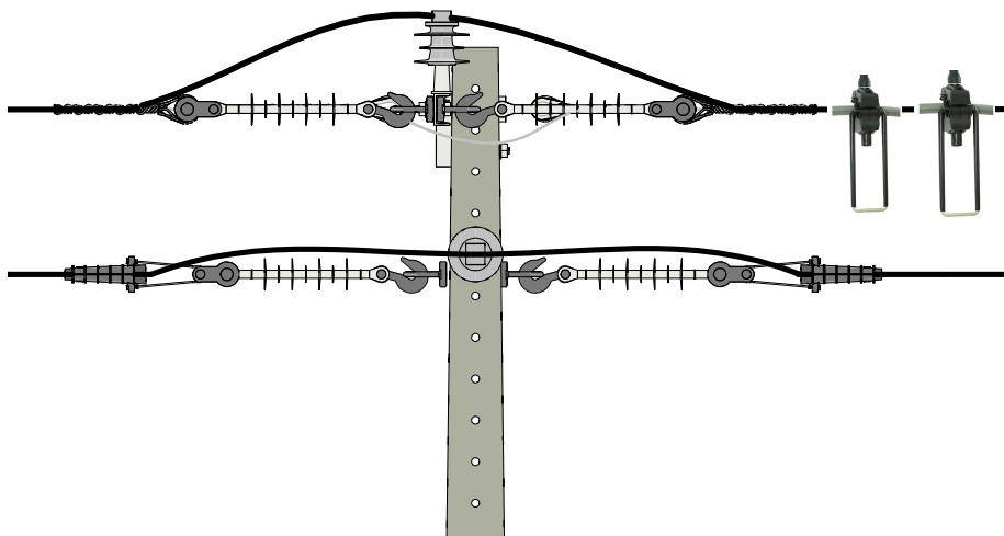
VISTA FRONTAL 1 : 20
