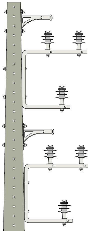
VISTA LATERAL
