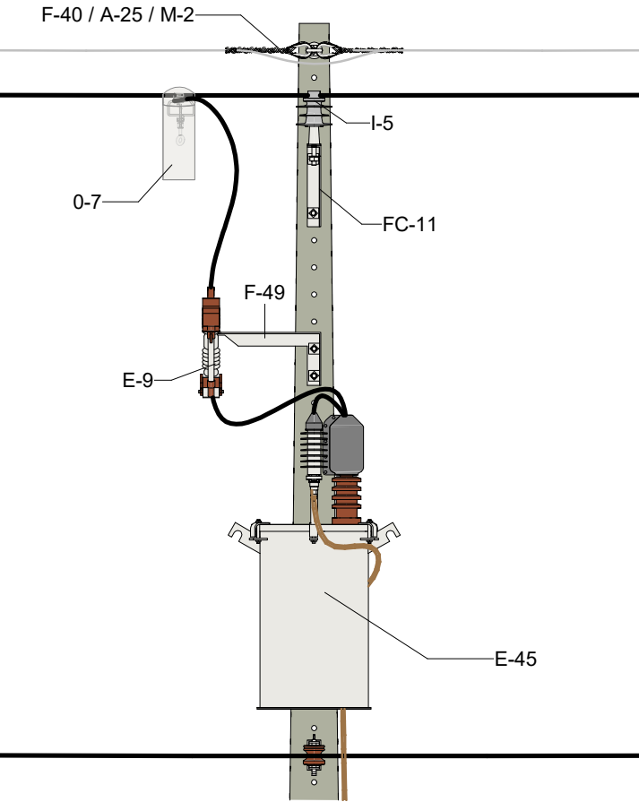
VISTA FRONTAL 1 : 25
