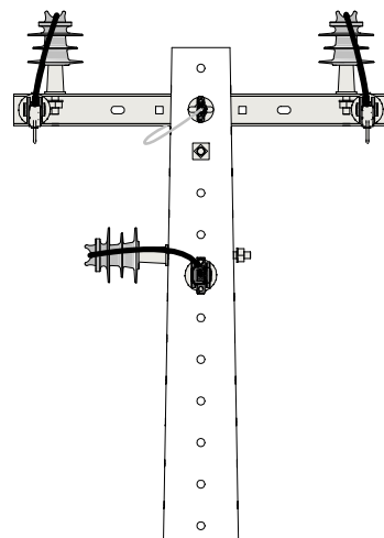
VISTA LATERAL 1 : 20
