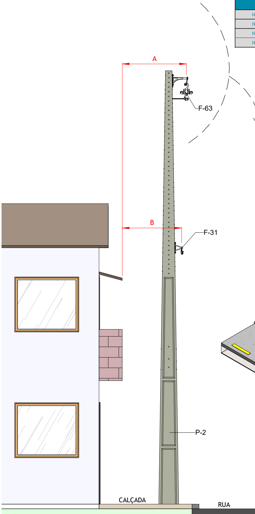
VISTA LATERAL 1 : 50
