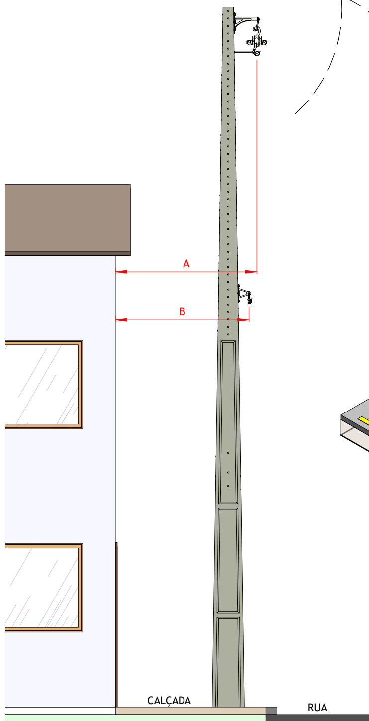
VISTA LATERAL
