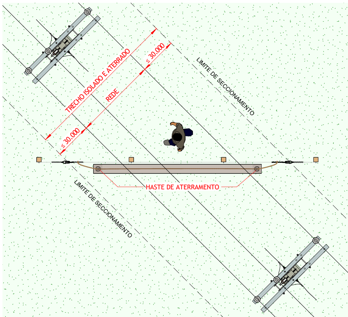
VISTA SUPERIOR
