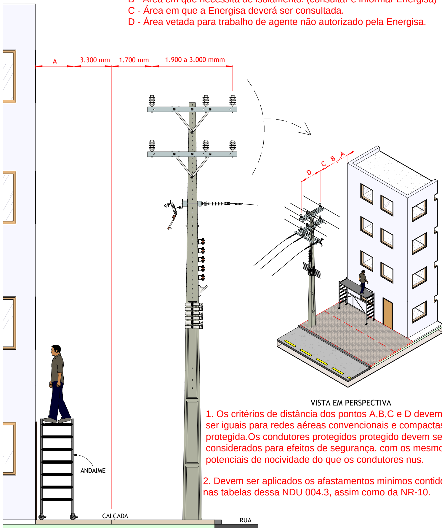
VISTA LATERAL
