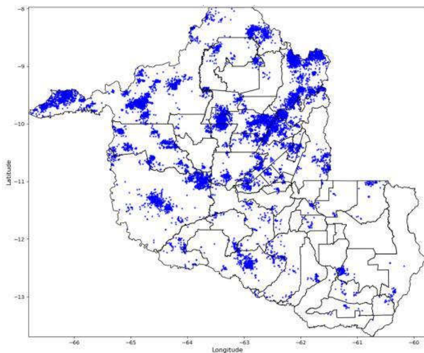
Figura 13 - Descargas Atmosféricas Observadas -18/03/2025. Fonte: Grupo STORM
