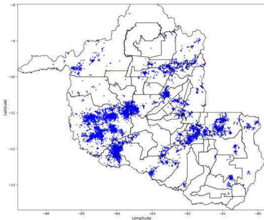
Figura 8 - Descargas Atmosféricas Observadas - 13/03/2025. Fonte: Grupo STORM
