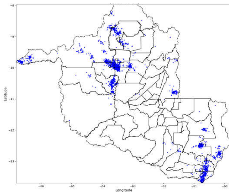
Figura 12 - Descargas Atmosféricas Observadas -29/03/2025. Fonte: Grupo STORM
