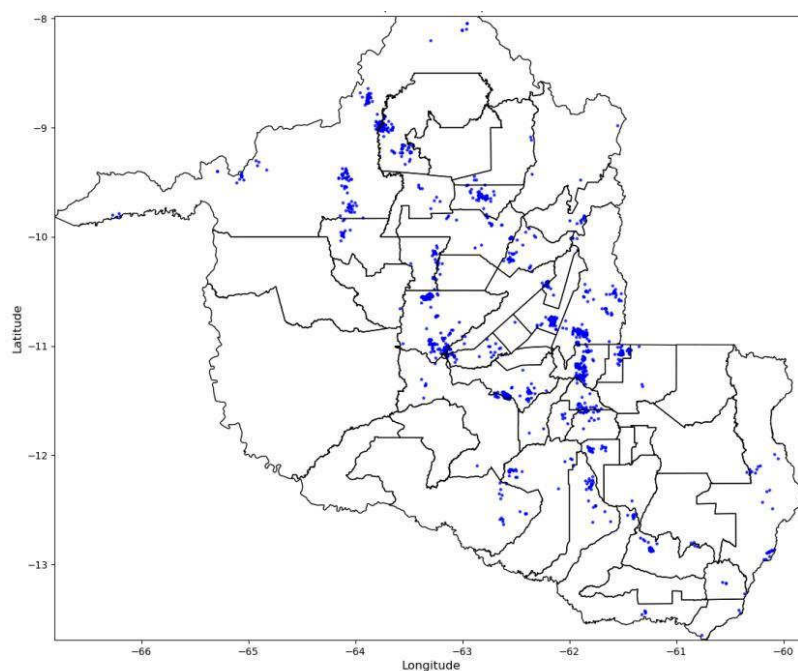
Figura 13 - Descargas Atmosféricas Observadas -30/03/2025. Fonte: Grupo STORM
