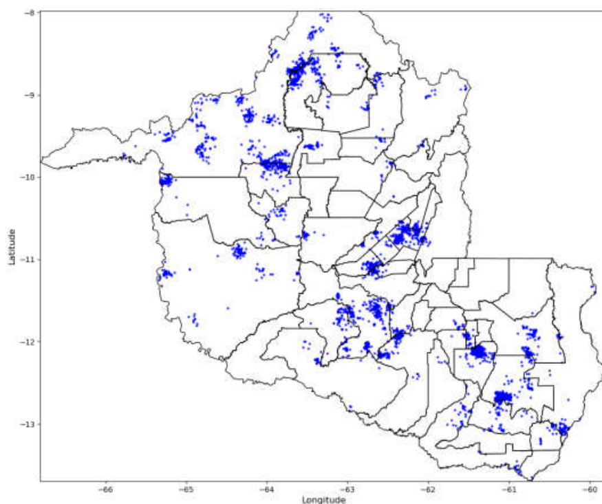
Figura 6 - Descargas Atmosféricas Observadas - 23/03/2025. Fonte: Grupo STORM
