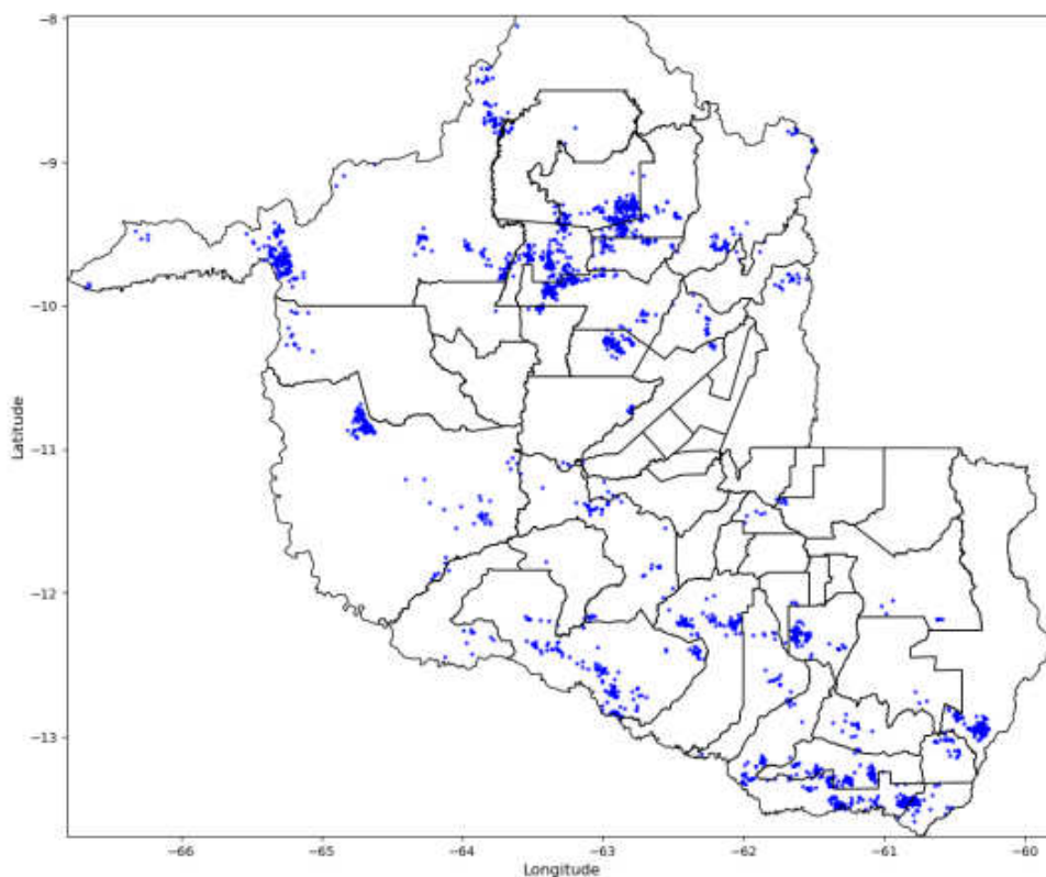
Figura 8 - Descargas Atmosféricas Observadas - 25/03/2025. Fonte: Grupo STORM
