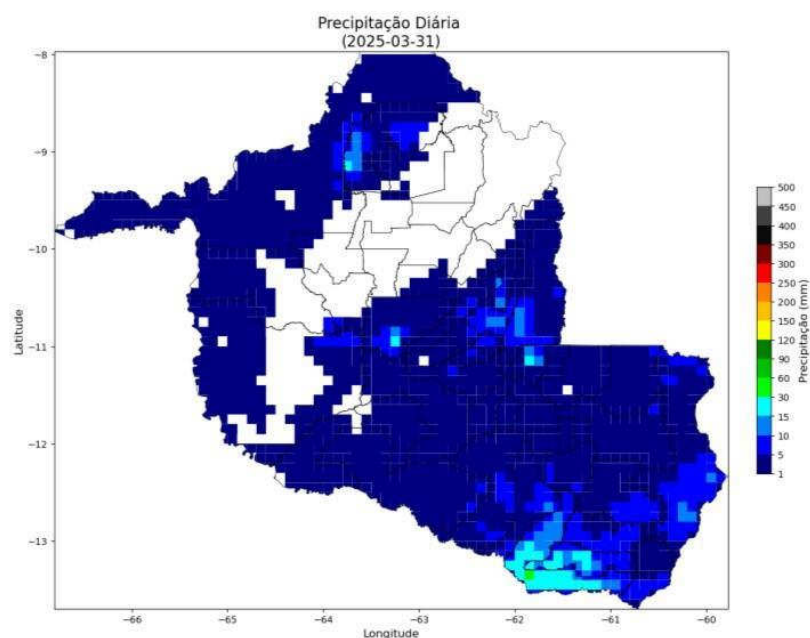
Figura 3 – Mapas de precipitação para os dias entre 21 e 31/03.
