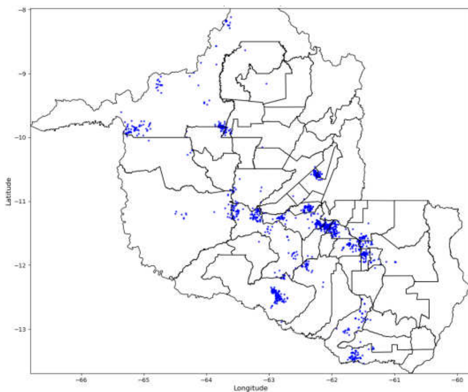
Figura 5 - Descargas Atmosféricas Observadas - 22/03/2025. Fonte: Grupo STORM
