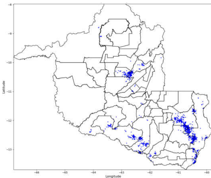
Figura 9 - Descargas Atmosféricas Observadas - 26/03/2025. Fonte: Grupo STORM
