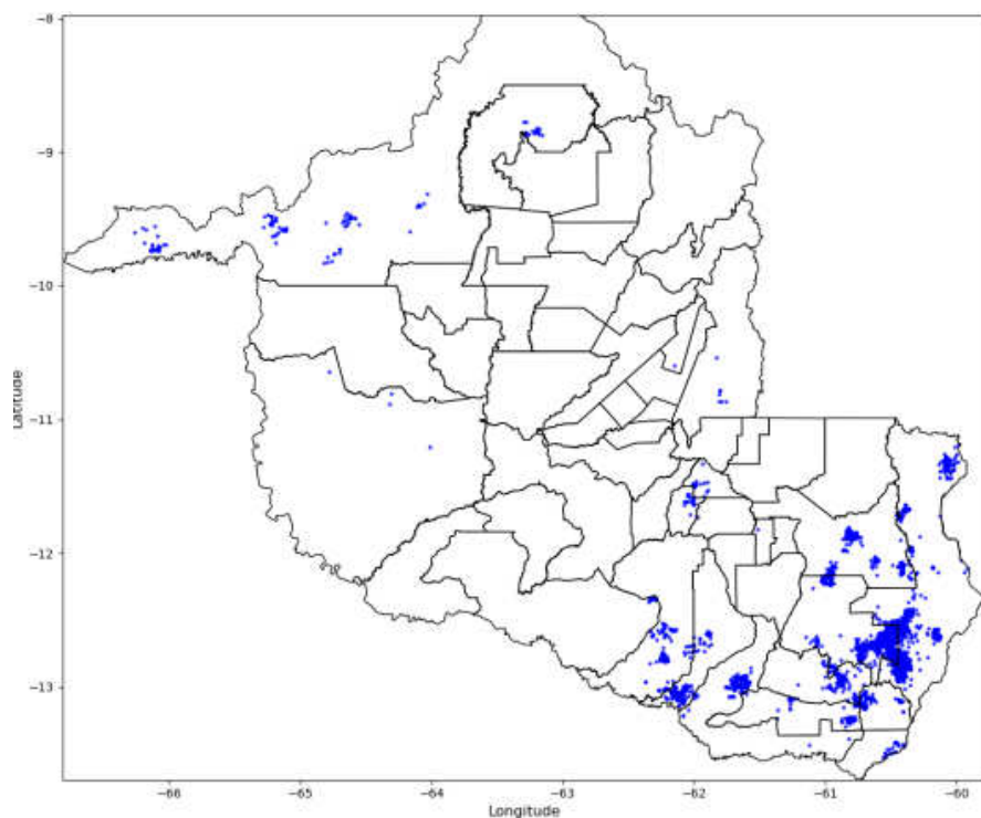
Figura 4 - Descargas Atmosféricas Observadas - 21/03/2025. Fonte: Grupo STORM
