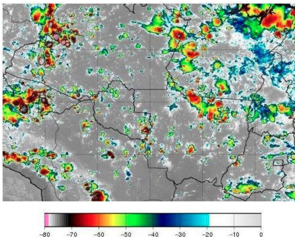
Figura 1 - Imagens de satélite no infravermelho com realce do satélite GOES-16 às 21:00 UT do dia 21/03. As cores indicam diferentes temperaturas dos topos das nuvens.
