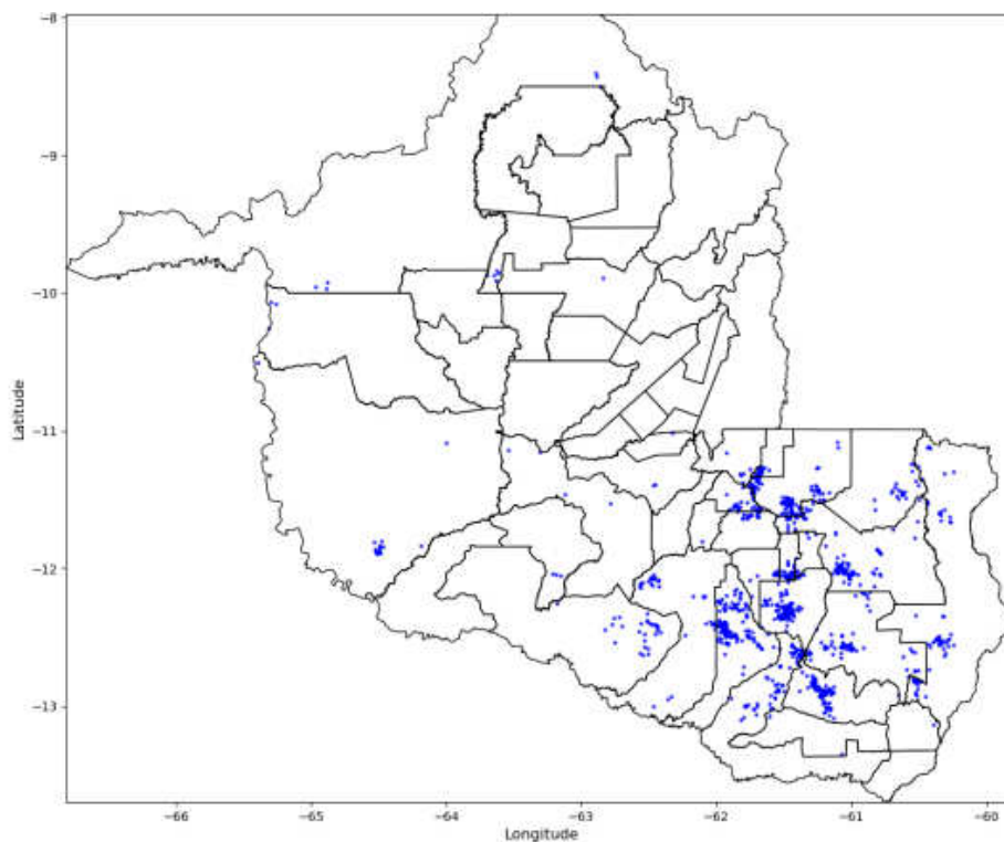
Figura 11 - Descargas Atmosféricas Observadas -28/03/2025. Fonte: Grupo STORM
