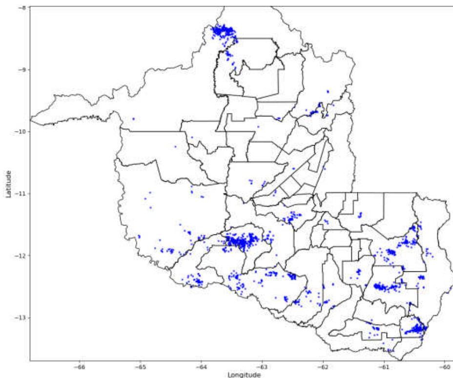
Figura 10 - Descargas Atmosféricas Observadas -27/03/2025. Fonte: Grupo STORM
