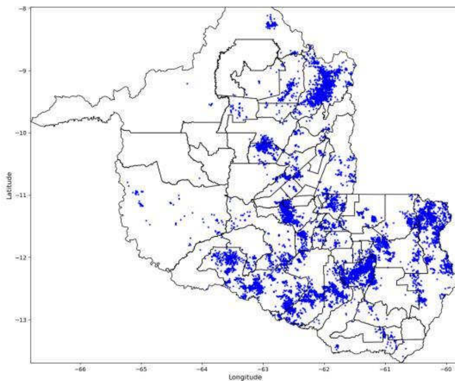
Figura 7 - Descargas Atmosféricas Observadas - 24/03/2025. Fonte: Grupo STORM
