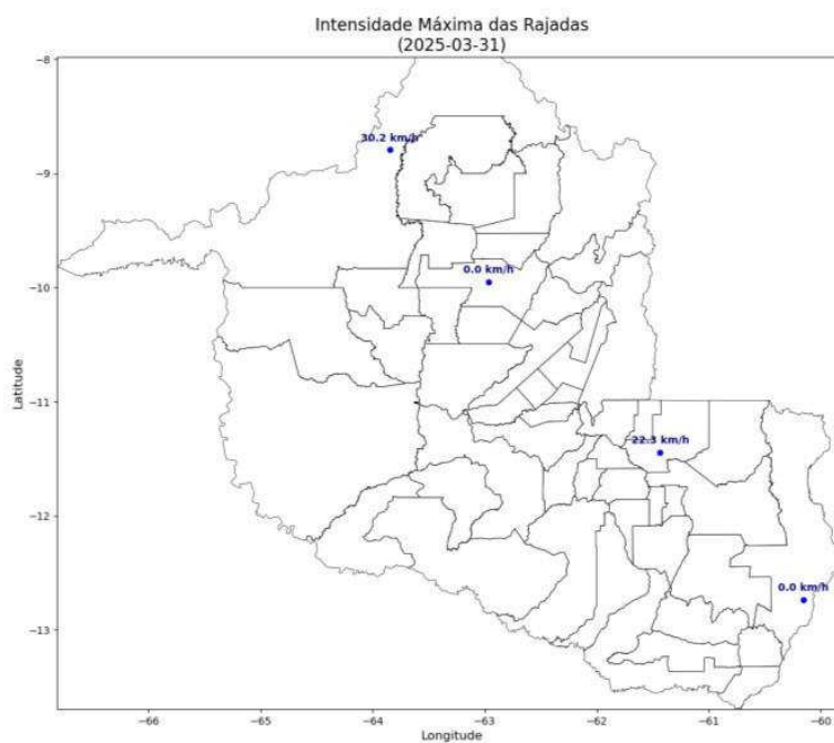
Figura 4 – Mapas de rajadas para os dias entre 21 e 31/03.
