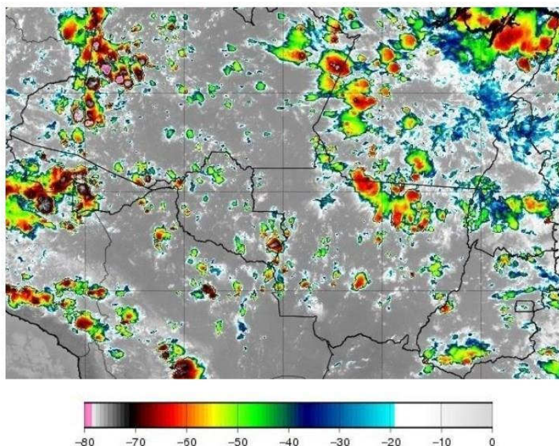
Figura 1 - Imagens de satélite no infravermelho com realce do satélite GOES-16 às 21:00 UT do dia 21/03. As cores indicam diferentes temperaturas dos topos das nuvens.
