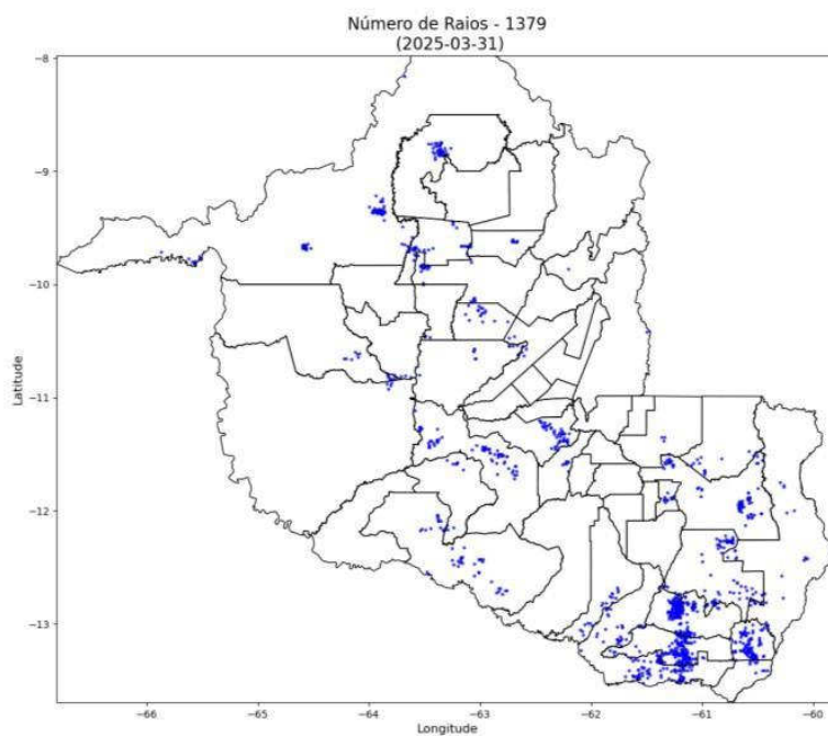
Figura 2 – Mapas de descargas atmosféricas para os dias entre 21 e 31/03.
