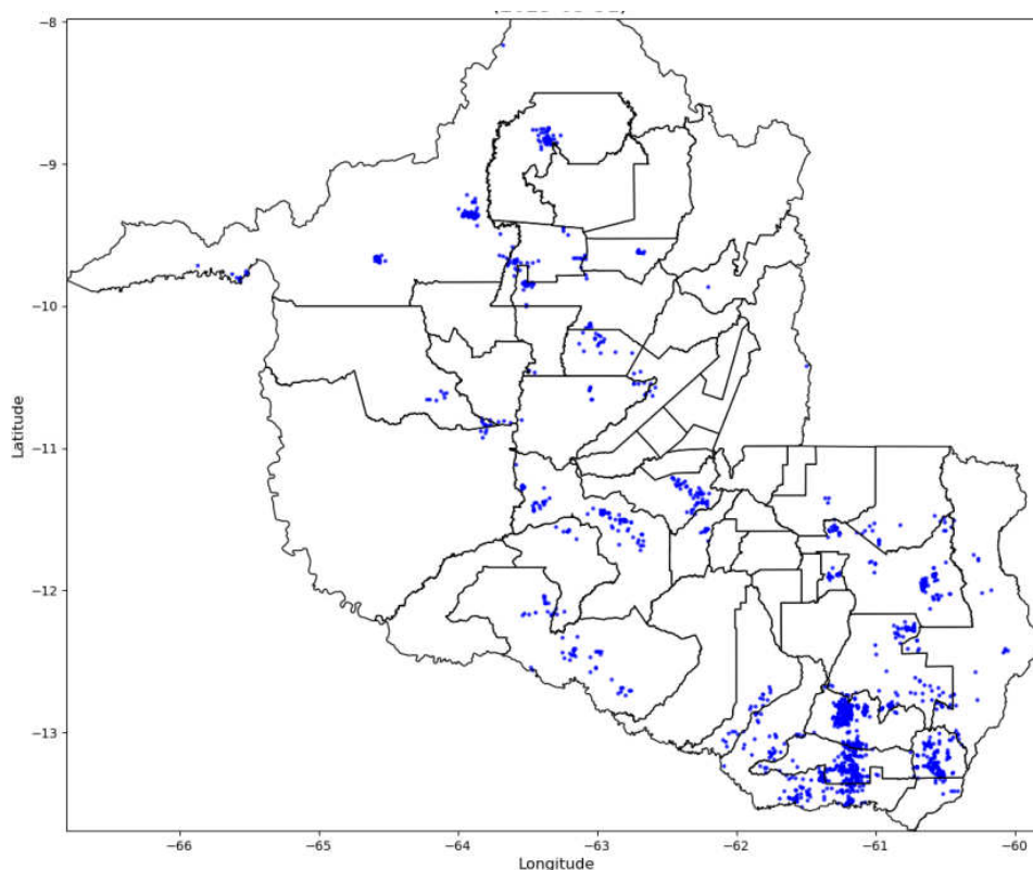
Figura 14 - Descargas Atmosféricas Observadas -31/03/2025. Fonte: Grupo STORM
