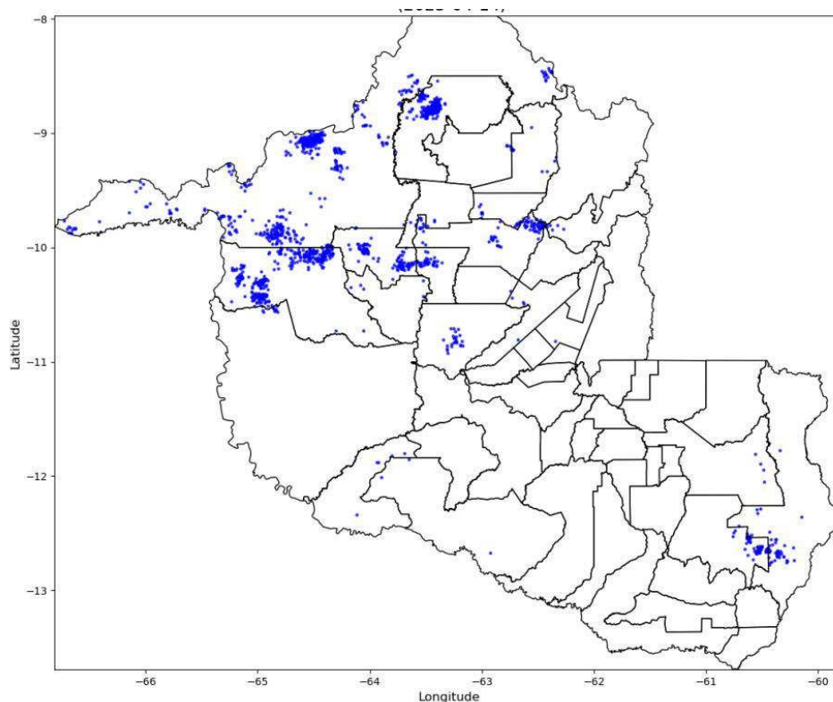
Figura 5 - Descargas Atmosféricas Observadas - 14/04/2025. Fonte: Grupo STORM
