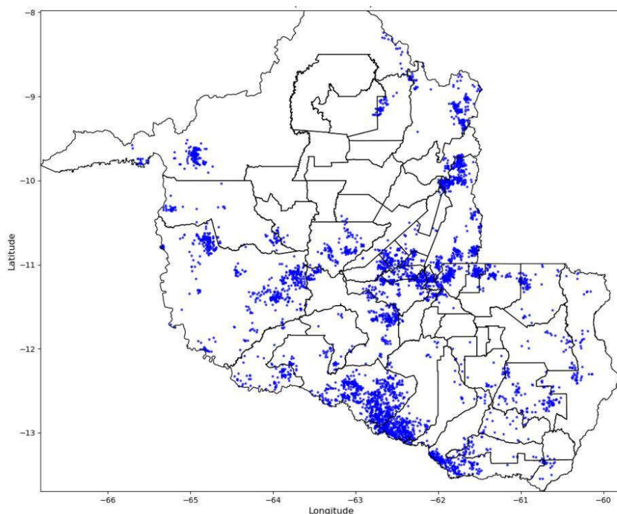
Figura 4 - Descargas Atmosféricas Observadas - 13/04/2025. Fonte: Grupo STORM
