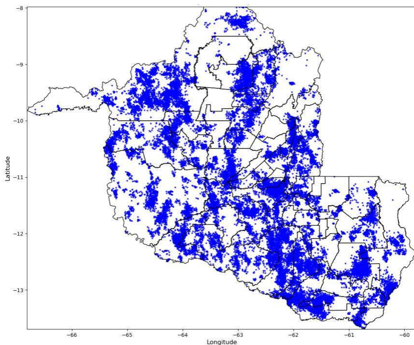
Figura 12 - Descargas Atmosféricas Observadas -21/04/2025. Fonte: Grupo STORM
