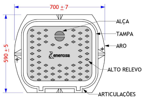
TAMPA E ARO ARTICULADOS PARA CAIXA TIPO CP1 - GARAGEM
