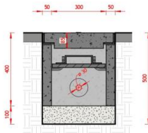
VISTA EM CORTE B 1 : 10
