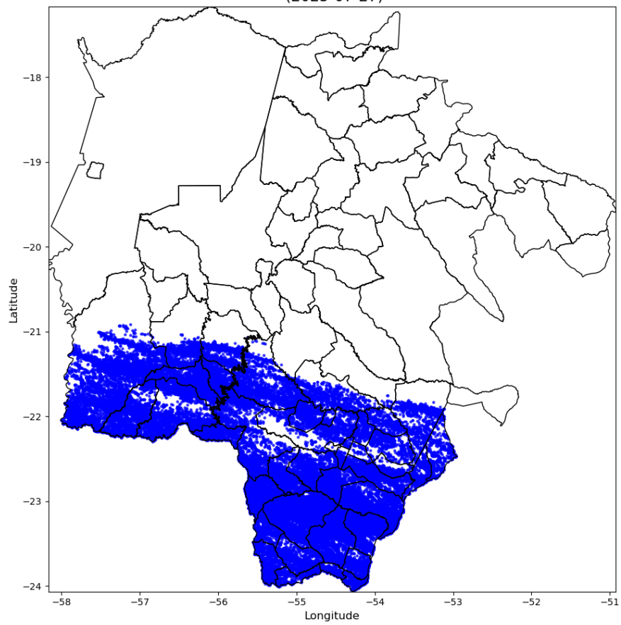
Número de Raios - 73564 (2025-07-27)
