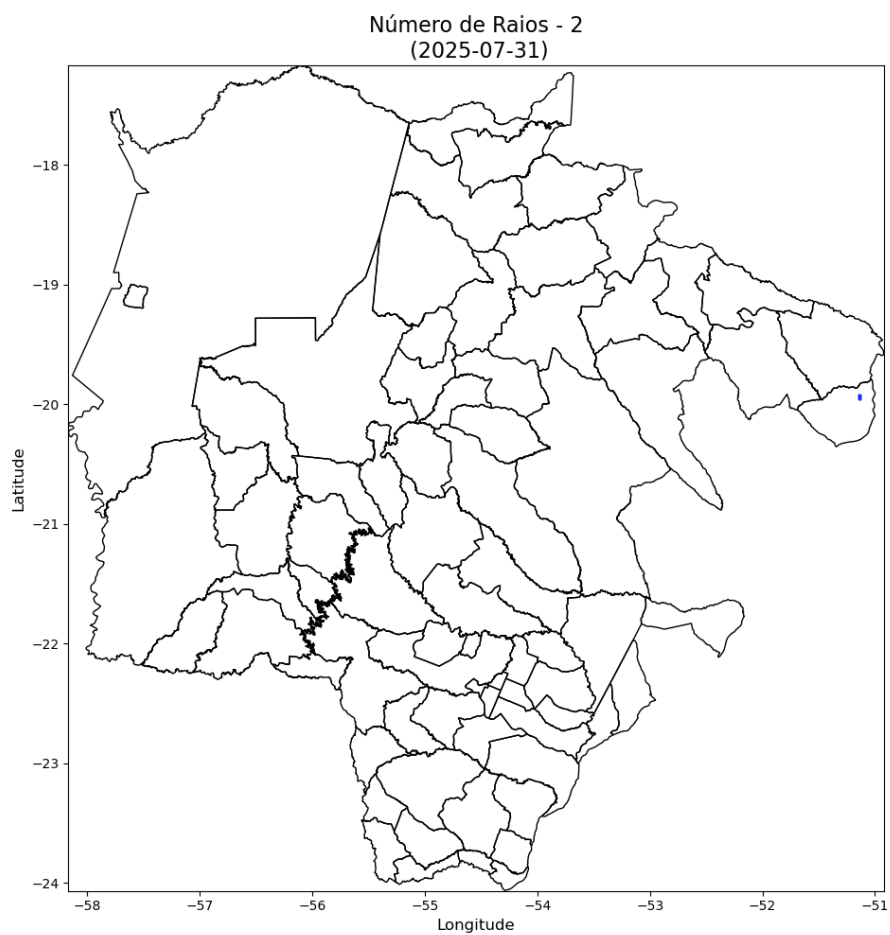
Figura 2 – Mapa de incidência de descargas atmosféricas nuvem-solo e intranuvem para os dias 24 a 31/07.
