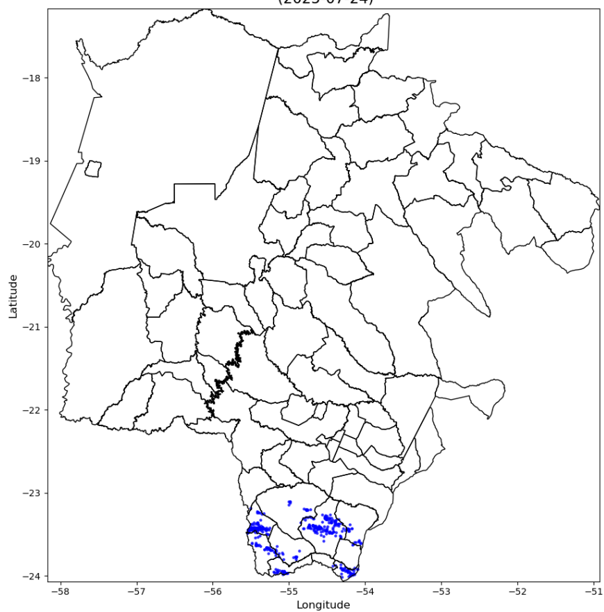
Número de Raios - 446 (2025-07-24)
