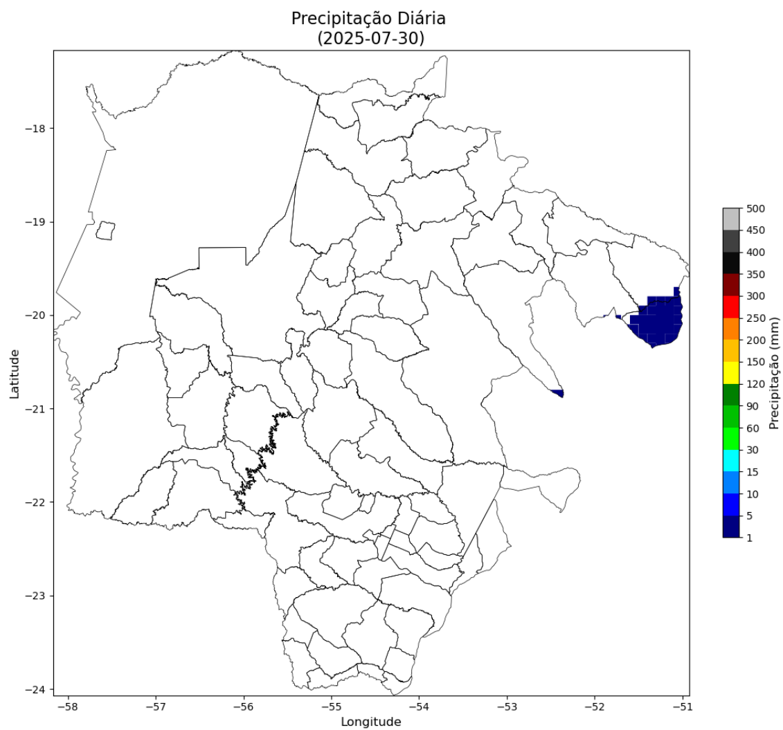
Figura 3 – Mapa de precipitação para os dias 24 a 30/07. Dia 31/07 não houve precipitação.
