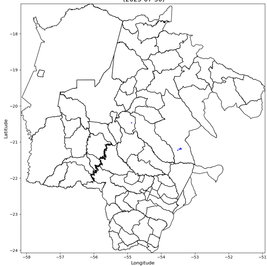
Número de Raios - 6 (2025-07-30)
