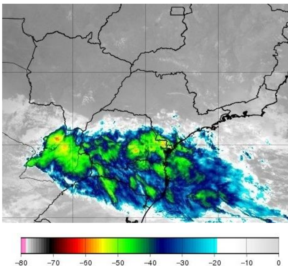
Figura 1 - Imagem de satélite no infravermelho com realce do satélite GOES-19 as 21:00 UT do dia 24/07. As cores indicam diferentes temperaturas dos topos das nuvens.
