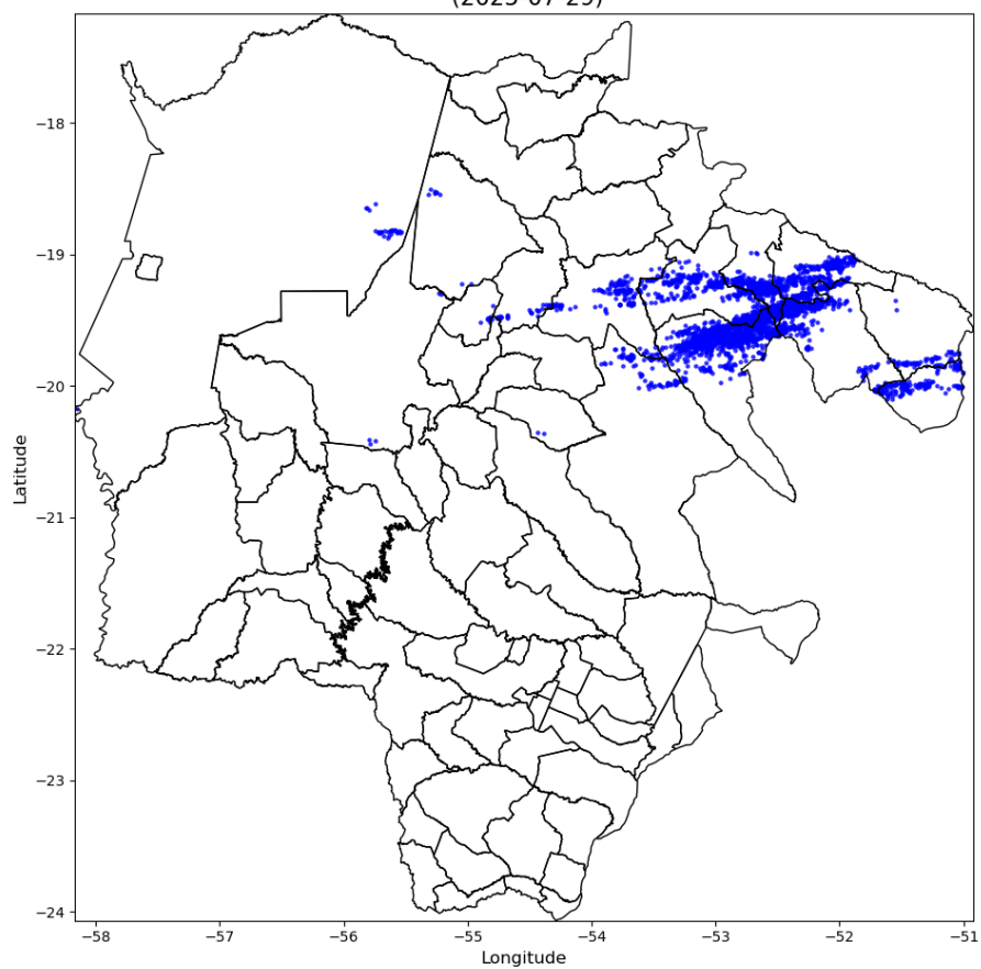
Número de Raios - 3976 (2025-07-29)
