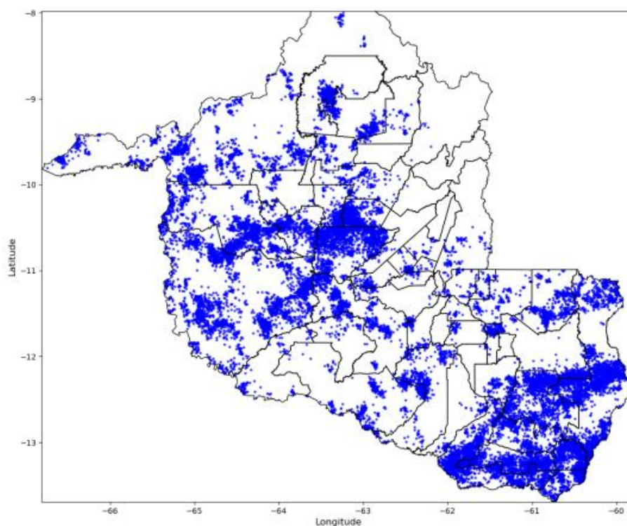
Figura 14 - Descargas Atmosféricas Observadas -19/03/2025. Fonte: Grupo STORM
