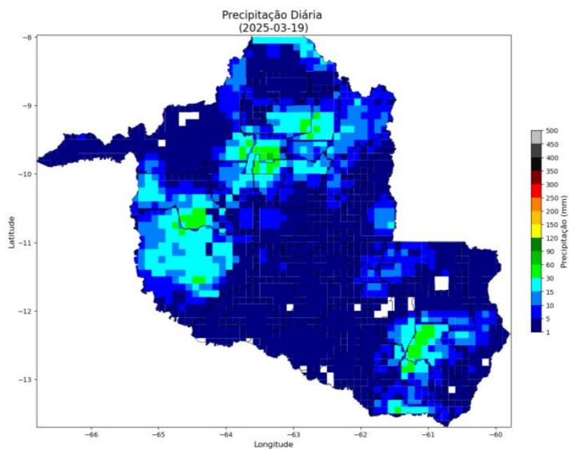
Figura 3 – Mapas de precipitação para os dias entre 09 e 19/03.
