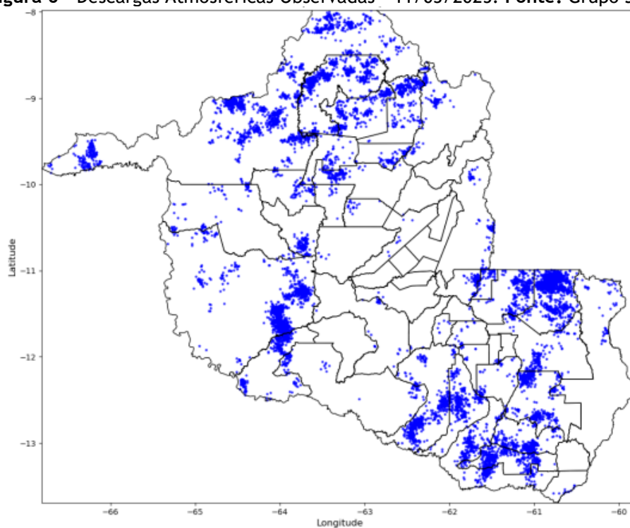
Figura 7 - Descargas Atmosféricas Observadas - 12/03/2025. Fonte: Grupo STORM
