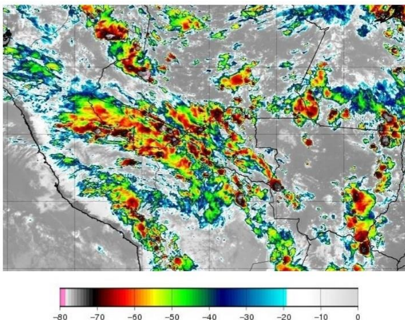
Figura 1 - Imagens de satélite no infravermelho com realce do satélite GOES-16 às 21:00 UT do dia 09/03. As cores indicam diferentes temperaturas dos topos das nuvens.
