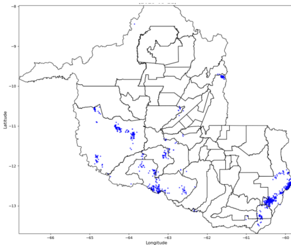
Figura 6 - Descargas Atmosféricas Observadas - 11/03/2025. Fonte: Grupo STORM
