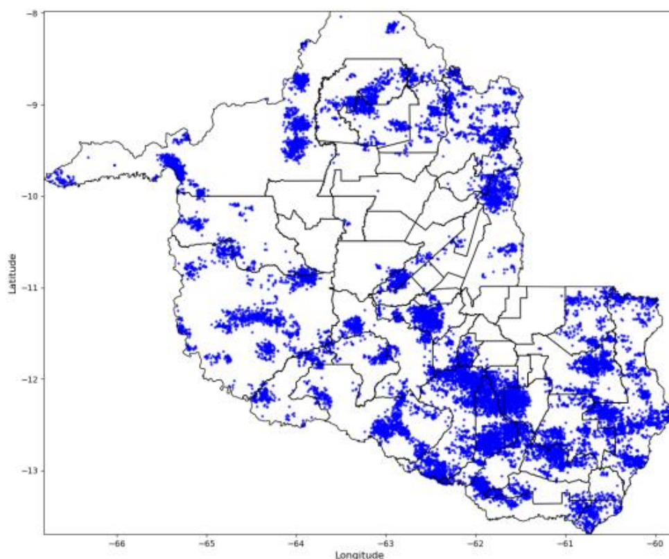
Figura 11 - Descargas Atmosféricas Observadas -16/03/2025. Fonte: Grupo STORM
