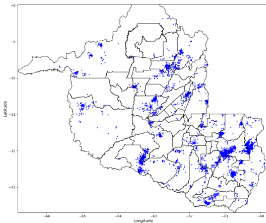
Figura 5 - Descargas Atmosféricas Observadas - 10/03/2025. Fonte: Grupo STORM
