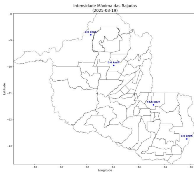
Figura 4 – Mapas de rajadas para os dias entre 09 e 19/03.
