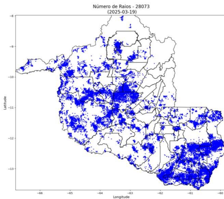
Figura 2 – Mapas de descargas atmosféricas para os dias entre 09 e 19/03.
