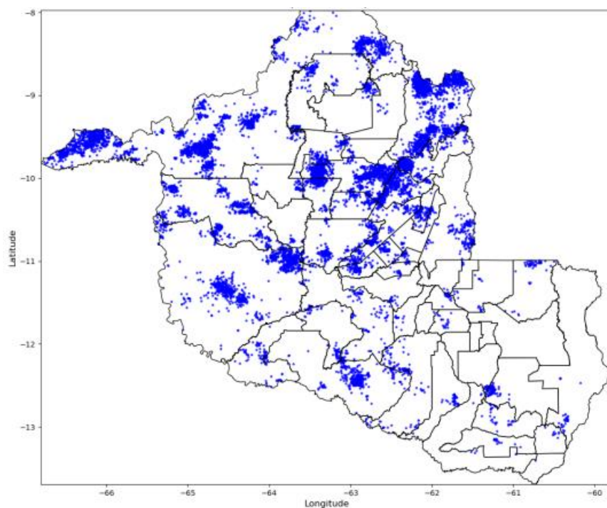
Figura 13 - Descargas Atmosféricas Observadas -18/03/2025. Fonte: Grupo STORM
