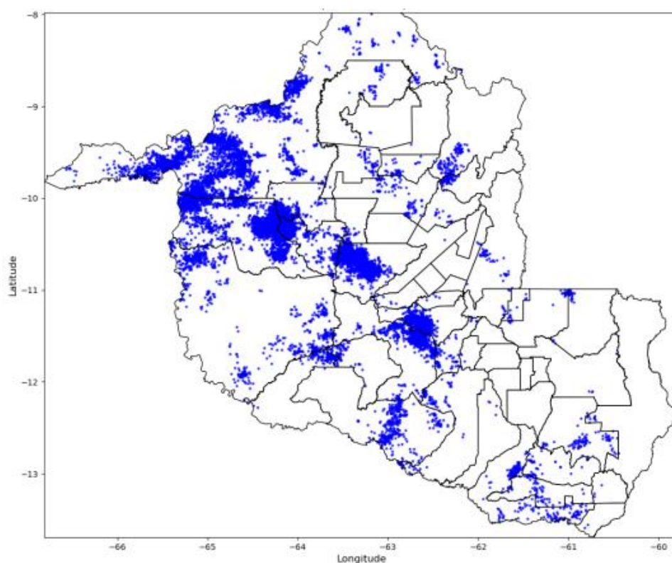
Figura 12 - Descargas Atmosféricas Observadas -17/03/2025. Fonte: Grupo STORM
