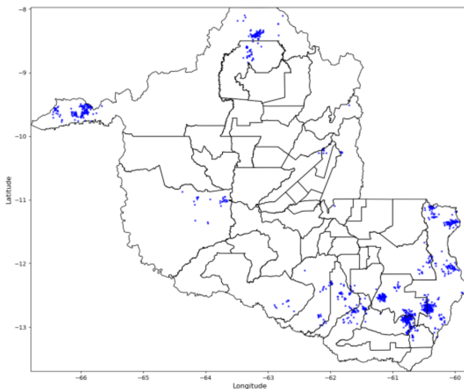
Figura 10 - Descargas Atmosféricas Observadas -15/03/2025. Fonte: Grupo STORM
