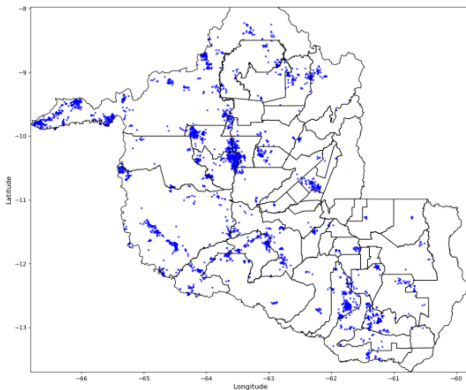
Figura 4 - Descargas Atmosféricas Observadas - 09/03/2025. Fonte: Grupo STORM
