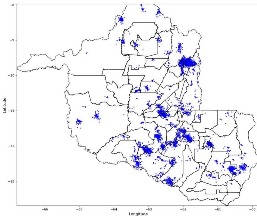
Figura 7 - Descargas Atmosféricas Observadas - 16/04/2025. Fonte: Grupo STORM
