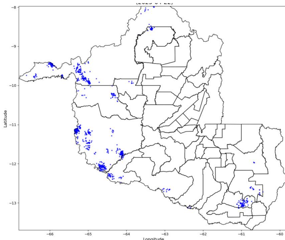
Figura 13 - Descargas Atmosféricas Observadas -22/04/2025. Fonte: Grupo STORM
