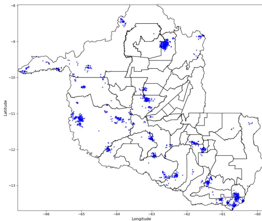
Figura 8 - Descargas Atmosféricas Observadas - 17/04/2025. Fonte: Grupo STORM
