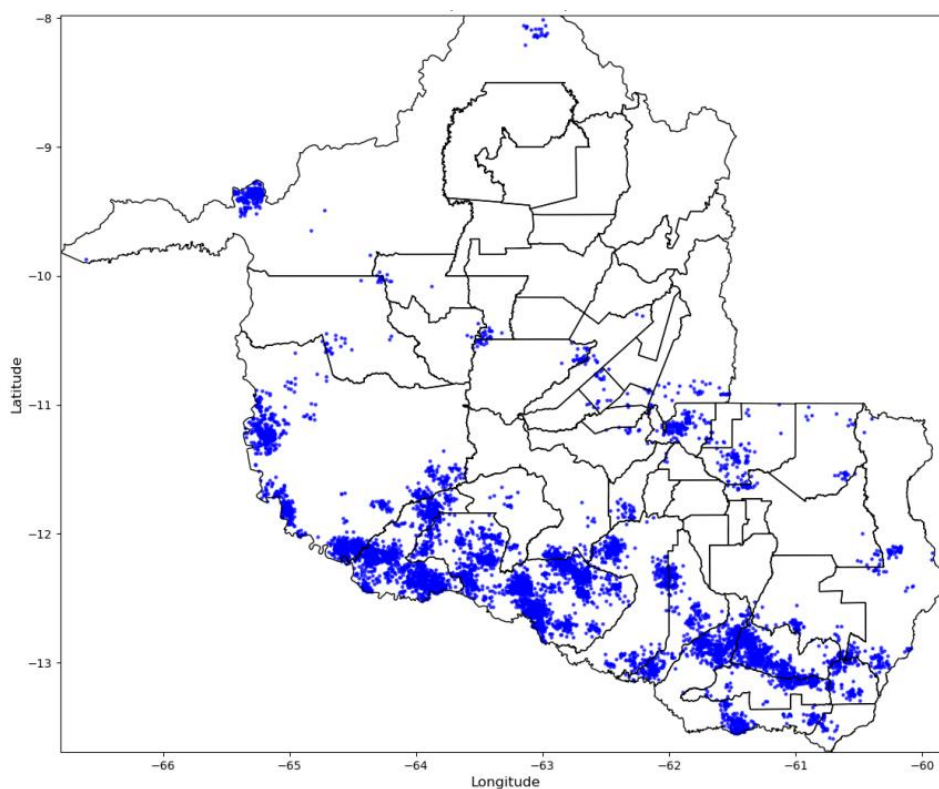
Figura 10 - Descargas Atmosféricas Observadas -19/04/2025. Fonte: Grupo STORM
