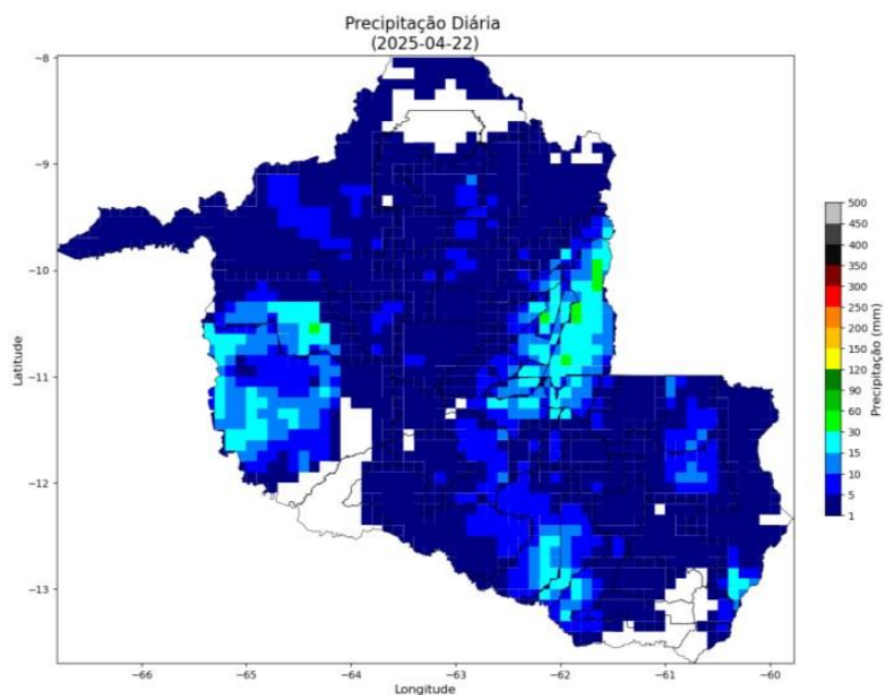
Figura 3 – Mapas de precipitação para os dias entre 13 e 22/04.
