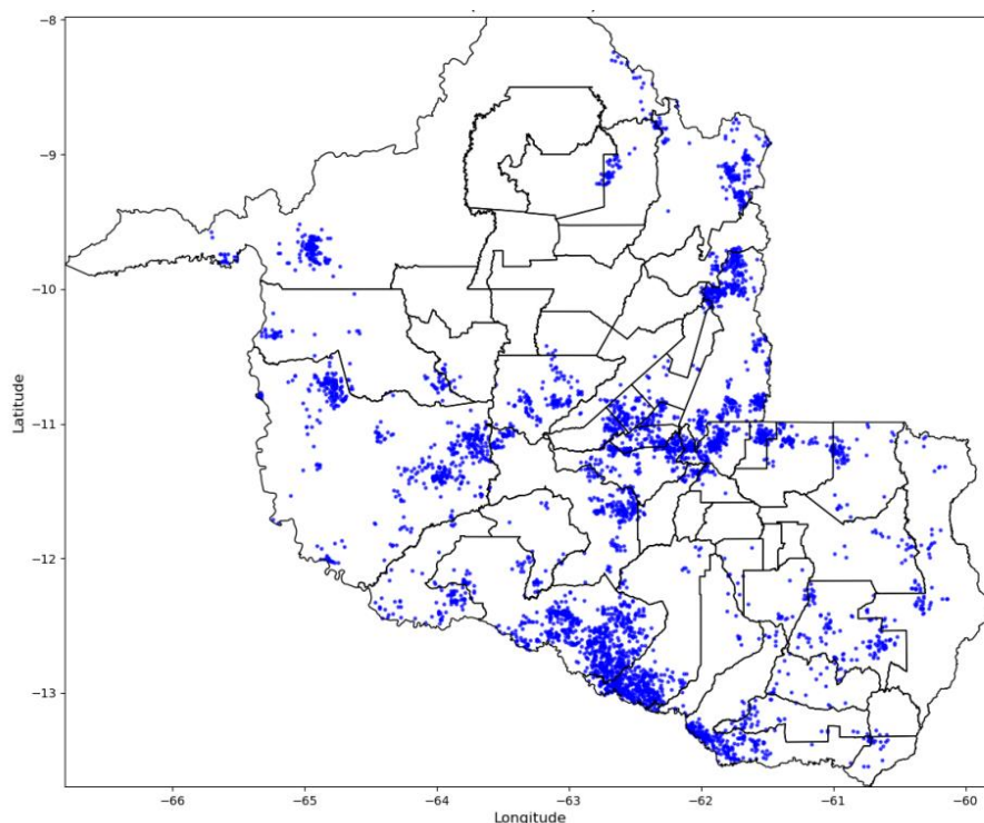
Figura 4 - Descargas Atmosféricas Observadas - 13/04/2025. Fonte: Grupo STORM
