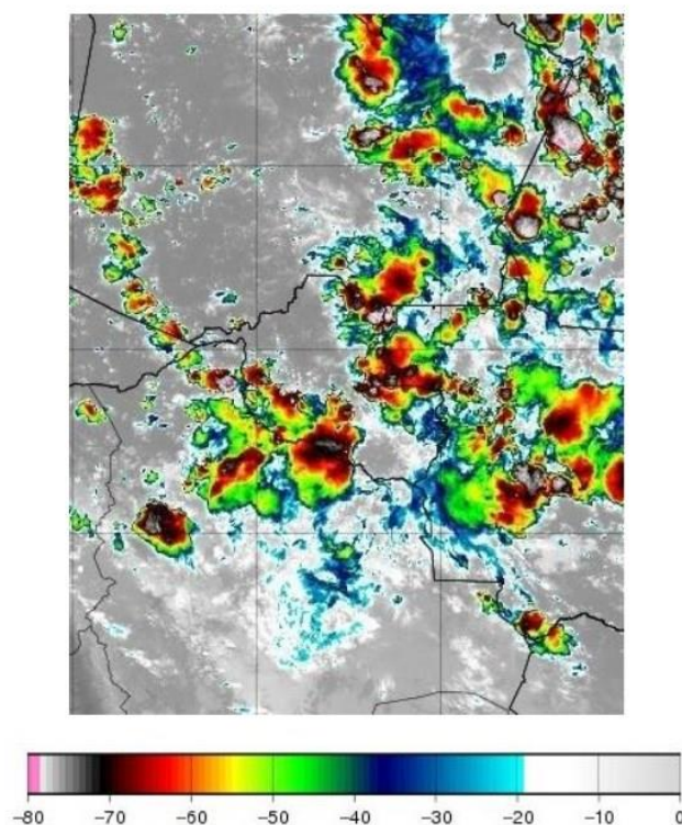
Figura 1 - Imagens de satélite no infravermelho com realce do satélite GOES-16 às 21:00 UT do dia 13/04. As cores indicam diferentes temperaturas dos topos das nuvens.
