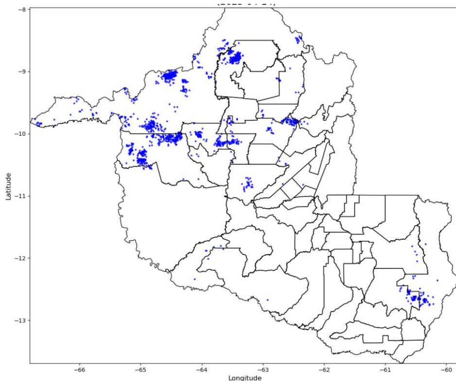
Figura 5 - Descargas Atmosféricas Observadas - 14/04/2025. Fonte: Grupo STORM
