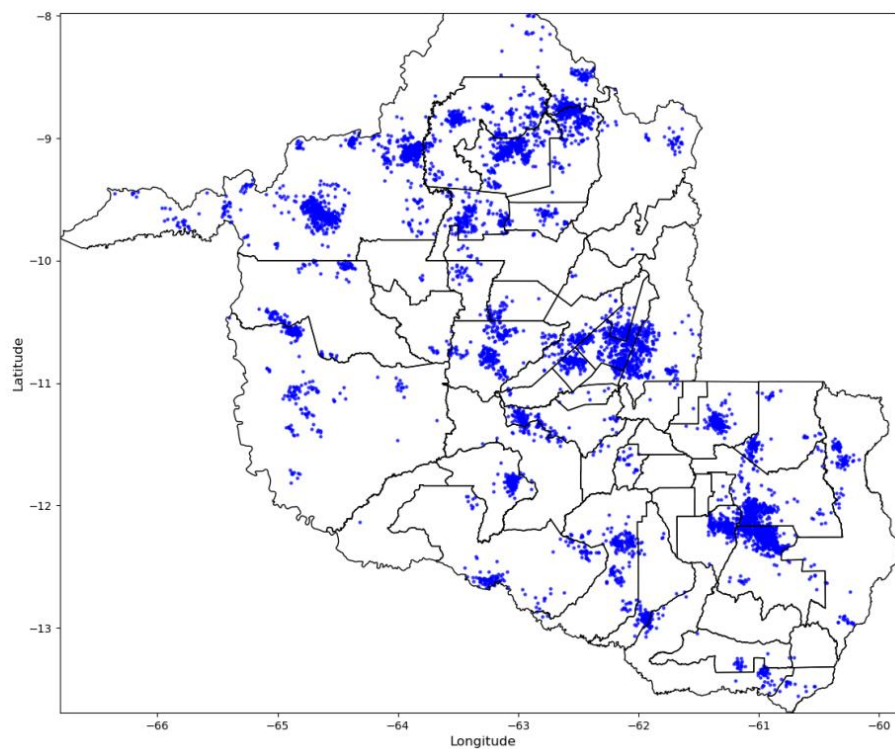
Figura 6 - Descargas Atmosféricas Observadas - 15/04/2025. Fonte: Grupo STORM
