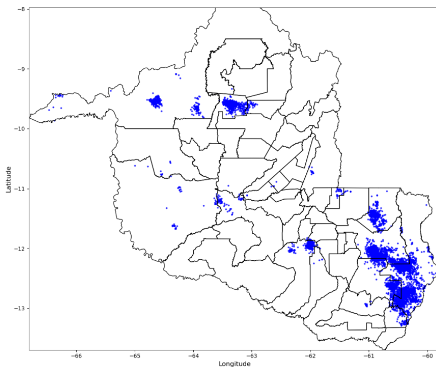
Figura 11 - Descargas Atmosféricas Observadas -20/04/2025. Fonte: Grupo STORM
