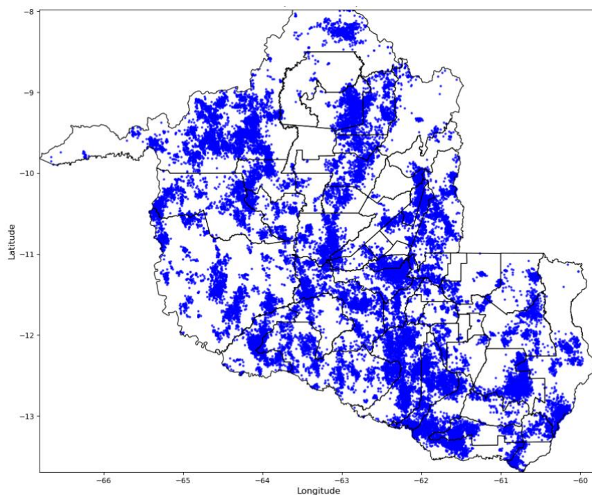
Figura 12 - Descargas Atmosféricas Observadas -21/04/2025. Fonte: Grupo STORM
