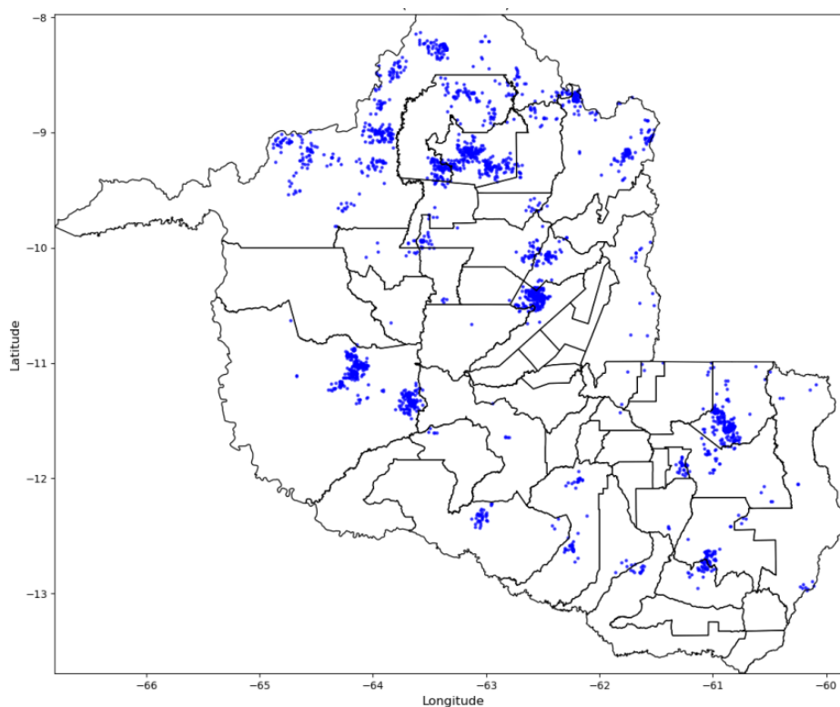
Figura 9 - Descargas Atmosféricas Observadas - 18/04/2025. Fonte: Grupo STORM
