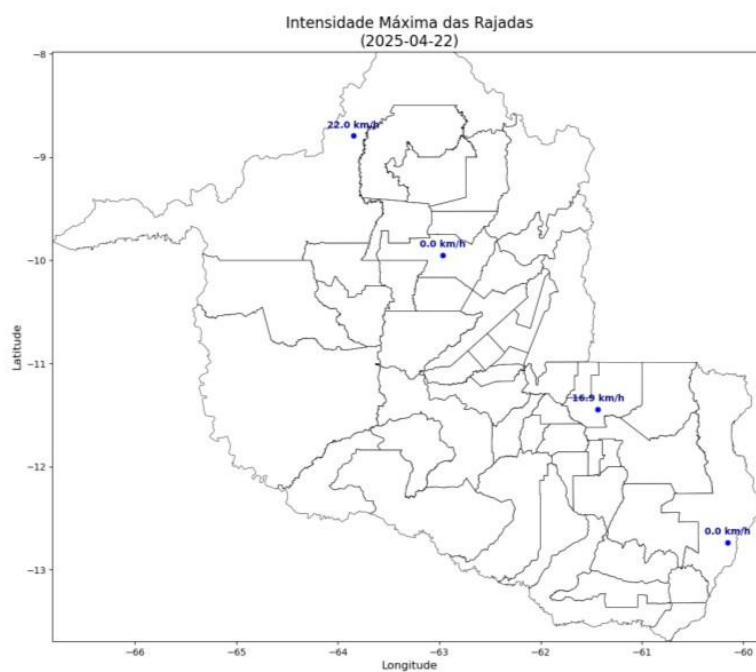
Figura 4 – Mapas de rajadas para os dias entre 13 e 22/04.
