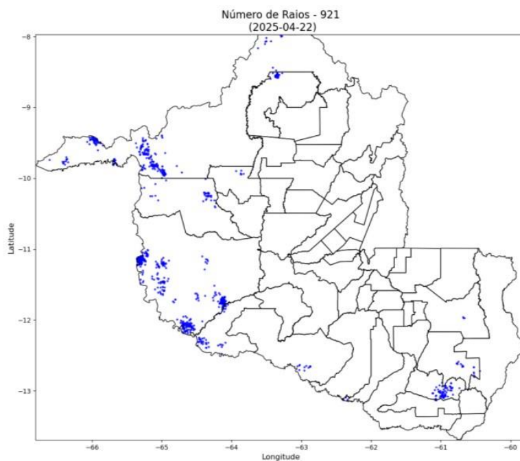
Figura 2 – Mapas de descargas atmosféricas para os dias entre 13 e 22/04.
