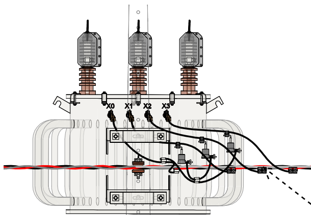
DIAGRAMA ELÉTRICO DE LIGAÇÃO DOS PRBT'S
