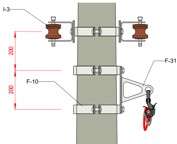
VISTA LATERAL
