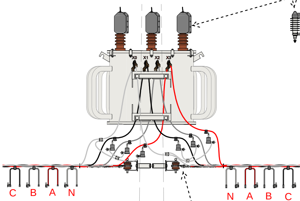
VISTA FRONTAL 1 : 25
