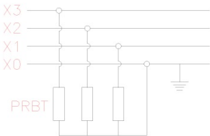
DIAGRAMA ELÉTRICO DE LIGAÇÃO DOS PRBT'S
