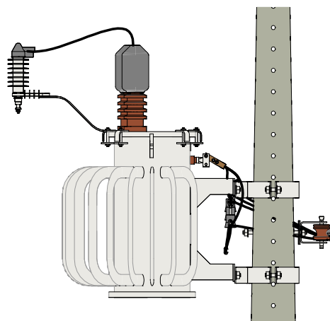
VISTA LATERAL 1 : 25
