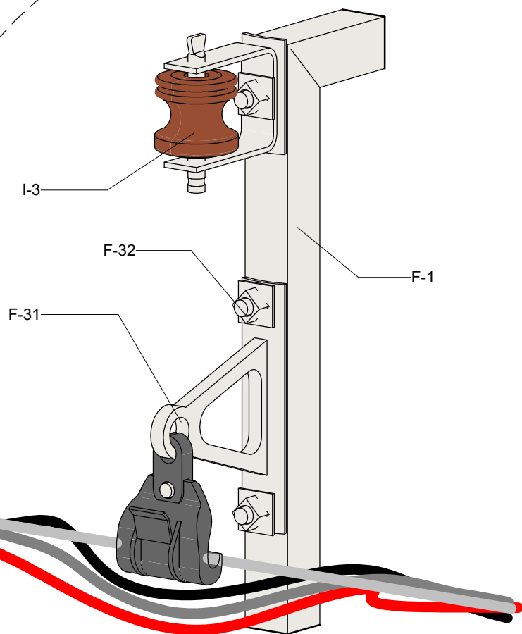
VISTA EM PERSPECTIVA - DETALHE
