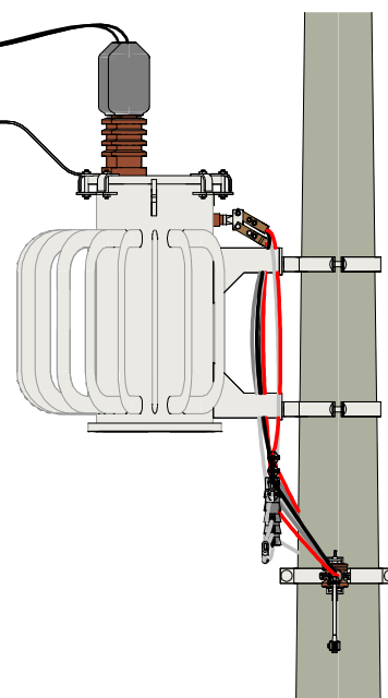
VISTA LATERAL 1 : 25
