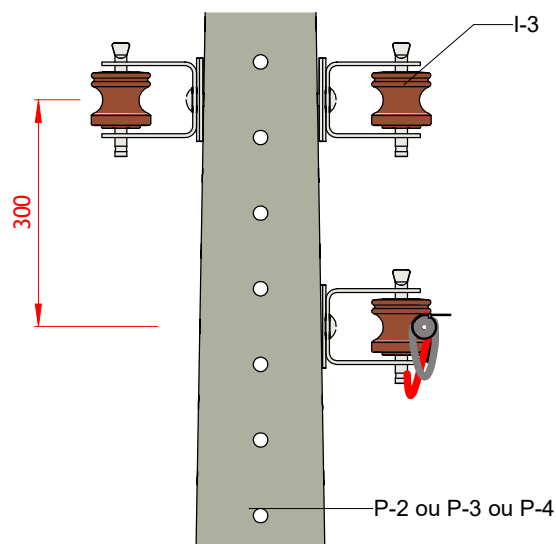
VISTA LATERAL 1 : 10
