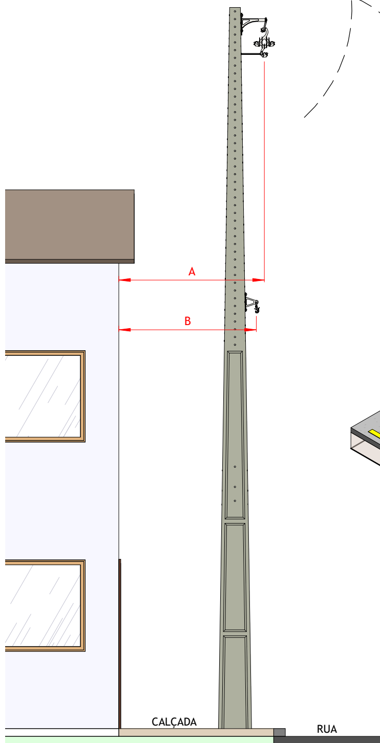
VISTA LATERAL 1 : 50
