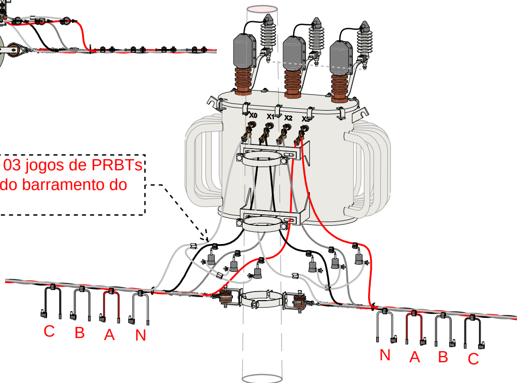
EM PERSPECTIVA
