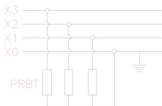
DIAGRAMA ELÉTRICO DE LIGAÇÃO DOS PRBT'S
