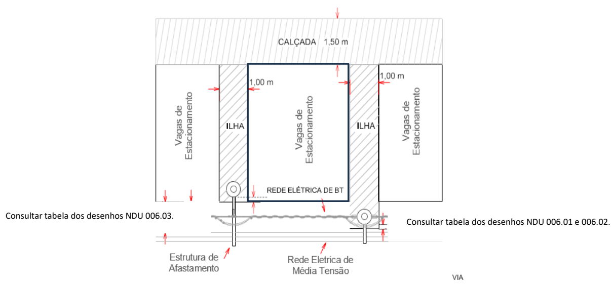
Figura 07. Localização de postes ao lado de vagas de estacionamento.
