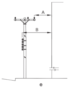
Afastamento horizontal entre os condutores e a parede de edificações
