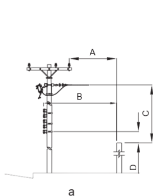
Afastamentos horizontal e vertical entre os condutores e o muro
