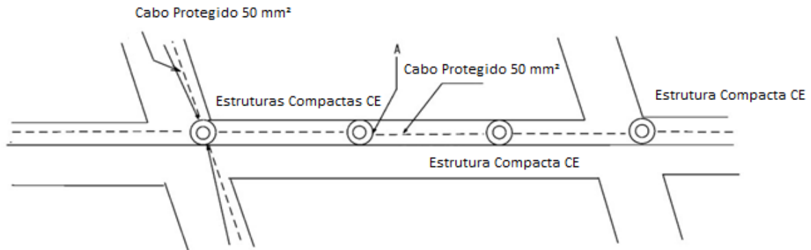
Disposição unilateral
