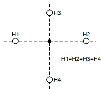
Figura 06. Cruzamento Aéreo - Rede aérea protegida.
