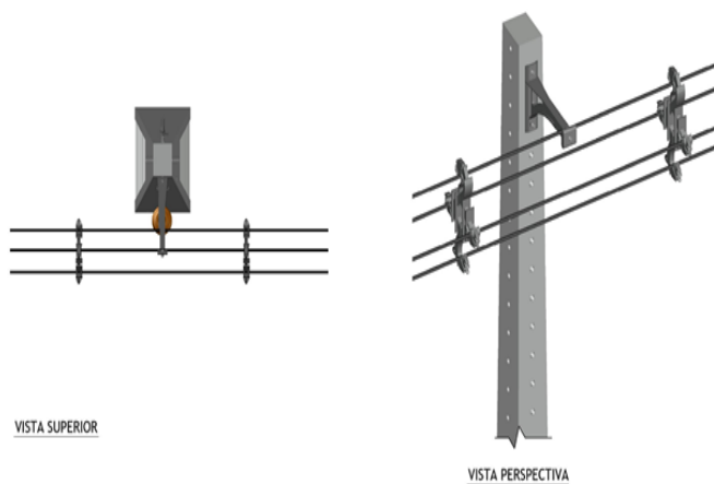
Estrutura CE 1
