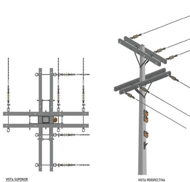
Estrutura N3
