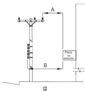
Afastamentos horizontal entre os condutores e as placas de publicidade
