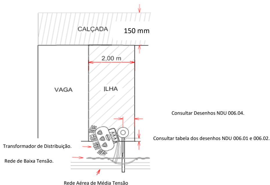
Figura 08. Dimensionamento da ilha para instalação de transformador ao lado de
