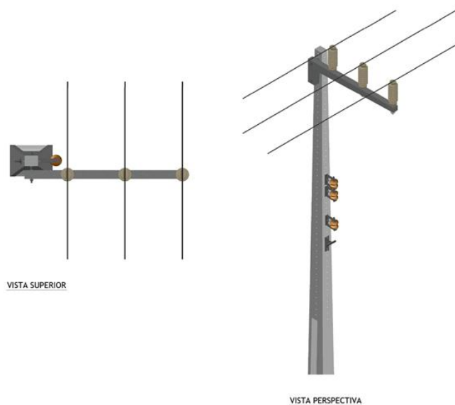
Estrutura B1
