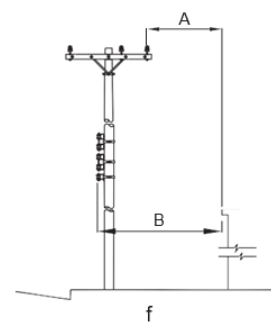
Afastamentos horizontal entre os condutores e a cimalha e o telhado de edificações
