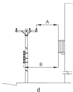
Afastamento horizontal entre os condutores e o piso da sacada, terraço e janela das edificações
