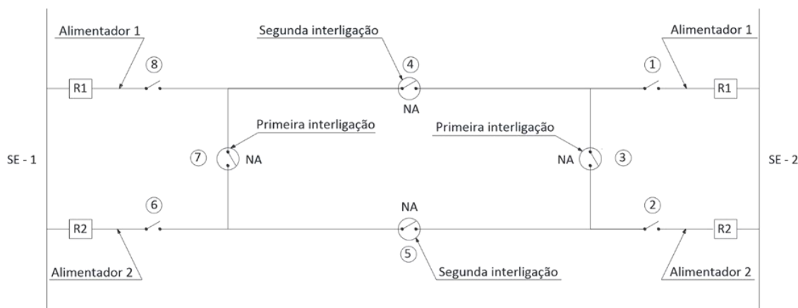
Legenda: Figura 15 - Interligação de alimentadores.
