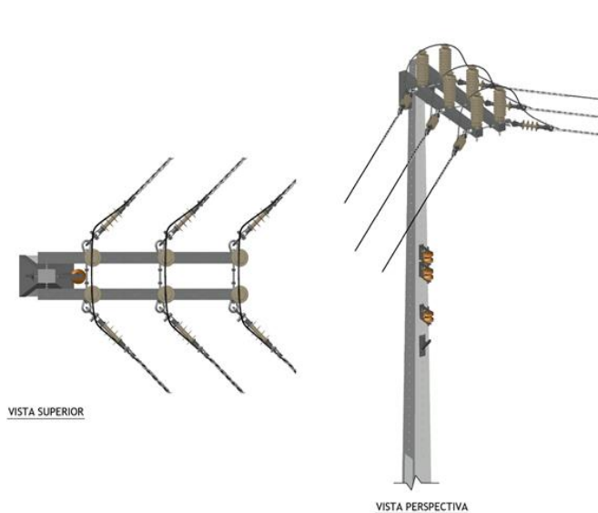
Estrutura B4
