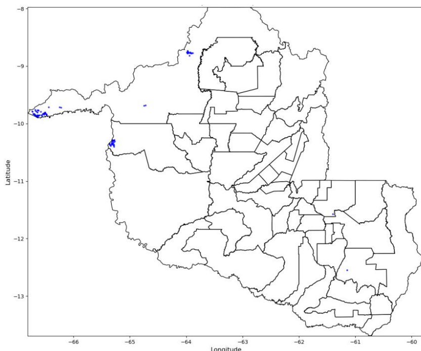
Figura 18 - Descargas Atmosféricas Observadas -15/05/2025. Fonte: Grupo STORM
