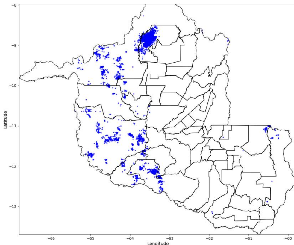
Figura 12 - Descargas Atmosféricas Observadas -09/05/2025. Fonte: Grupo STORM
