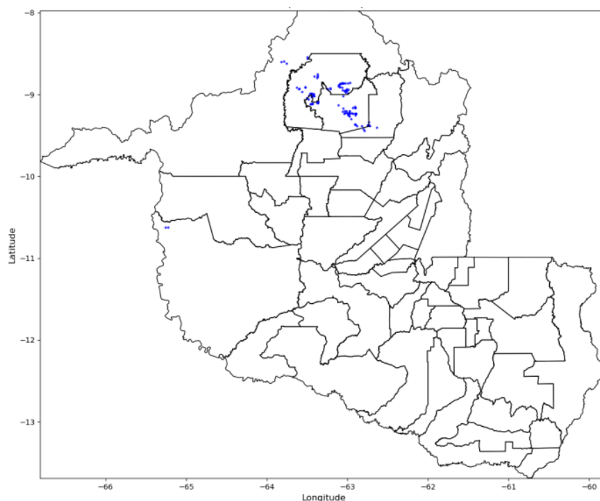
Figura 15 - Descargas Atmosféricas Observadas -12/05/2025. Fonte: Grupo STORM
