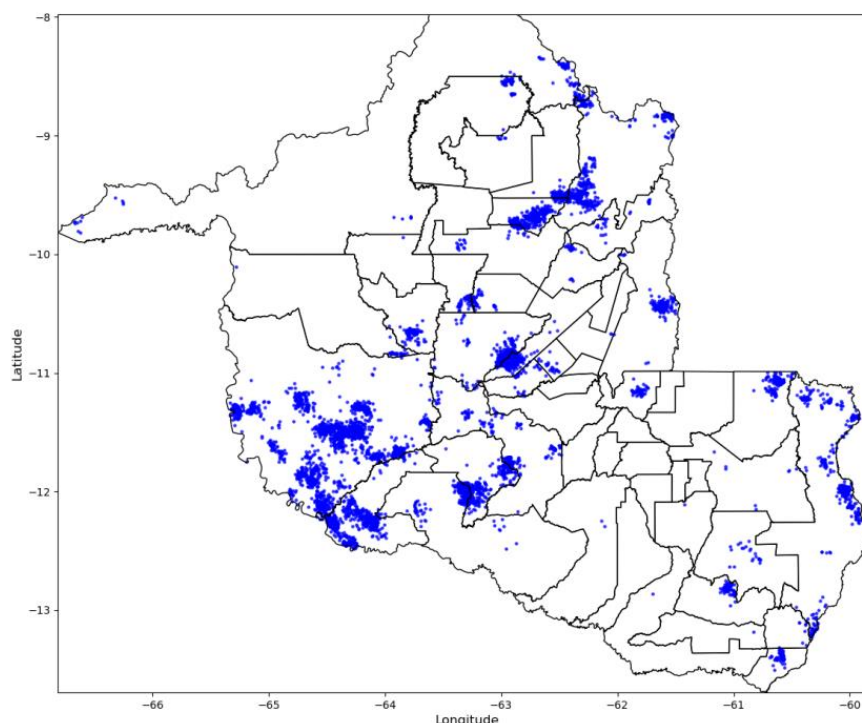
Figura 9 - Descargas Atmosféricas Observadas - 06/05/2025. Fonte: Grupo STORM
