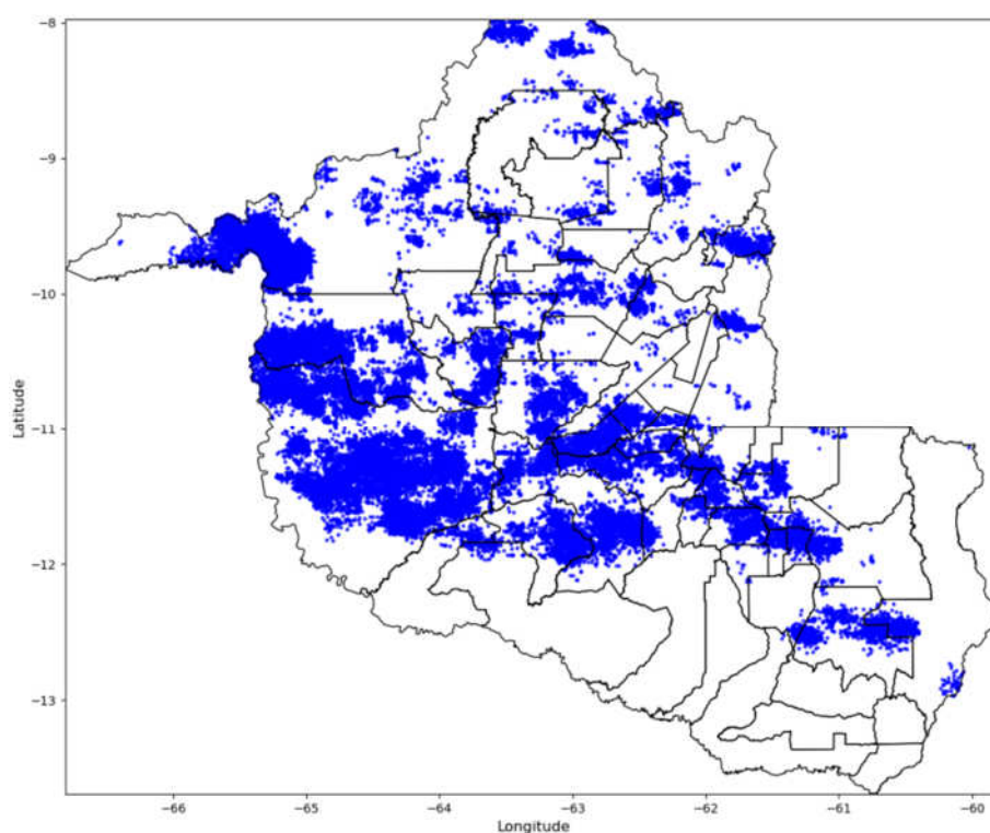
Figura 10 - Descargas Atmosféricas Observadas 05/09/2025. Fonte: Grupo STORM
