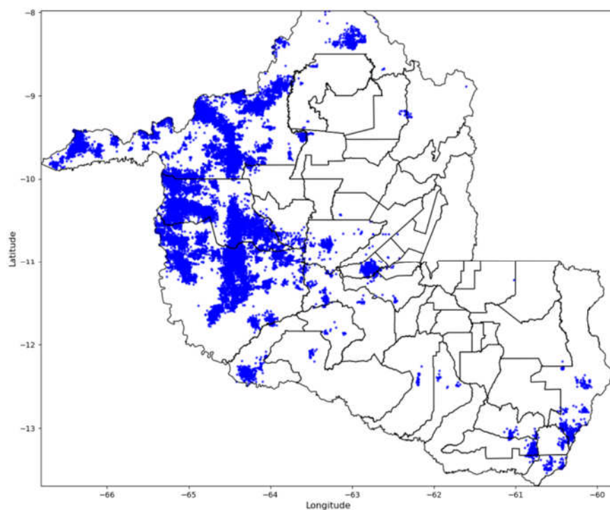
Figura 9 - Descargas Atmosféricas Observadas - 04/09/2025. Fonte: Grupo STORM
