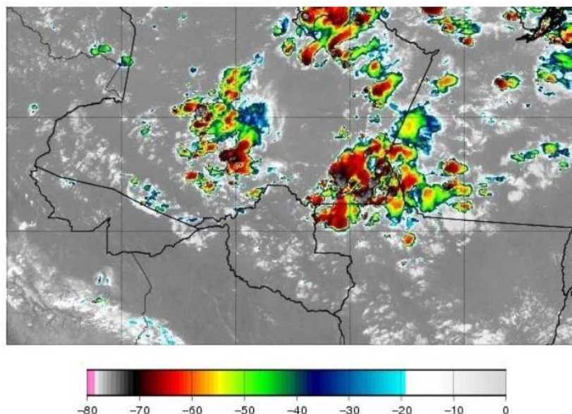
Figura 1 - Imagens de satélite no infravermelho com realce do satélite GOES-19 às 21:00 UT do dia 30/08. As cores indicam diferentes temperaturas dos topos das nuvens.
