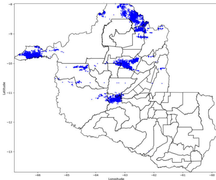
Figura 11 - Descargas Atmosféricas Observadas 06/09/2025. Fonte: Grupo STORM
