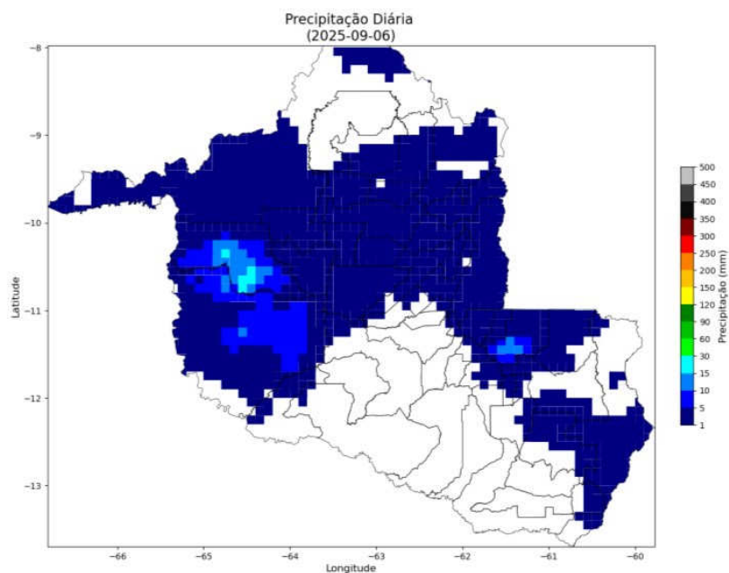
Figura 3 – Mapas de precipitação para os dias entre 30/08 e 06/09.
