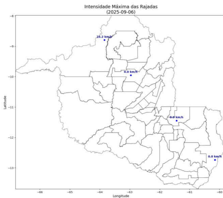
Figura 4 – Mapas de rajadas para os dias entre 30/08 e 06/09.
