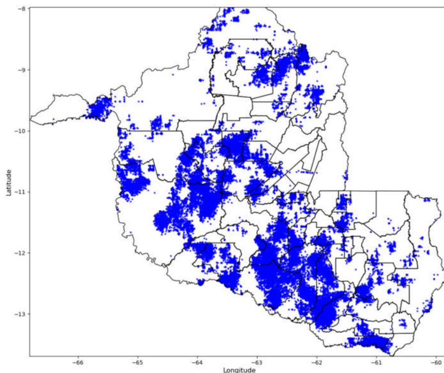
Figura 5 - Descargas Atmosféricas Observadas - 31/08/2025. Fonte: Grupo STORM
