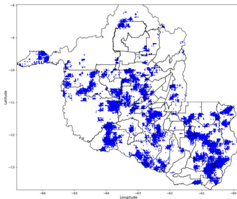
Figura 6 - Descargas Atmosféricas Observadas - 01/09/2025. Fonte: Grupo STORM
