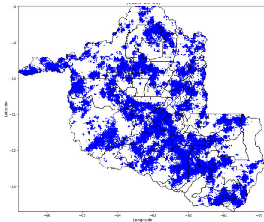
Figura 8 - Descargas Atmosféricas Observadas - 03/09/2025. Fonte: Grupo STORM
