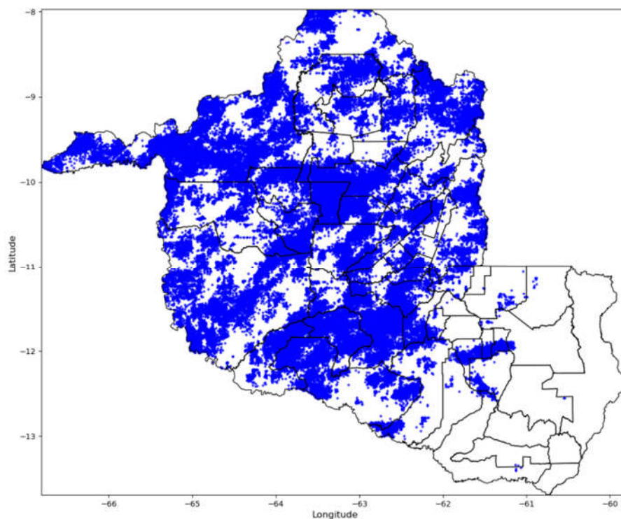
Figura 7 - Descargas Atmosféricas Observadas - 02/09/2025. Fonte: Grupo STORM
