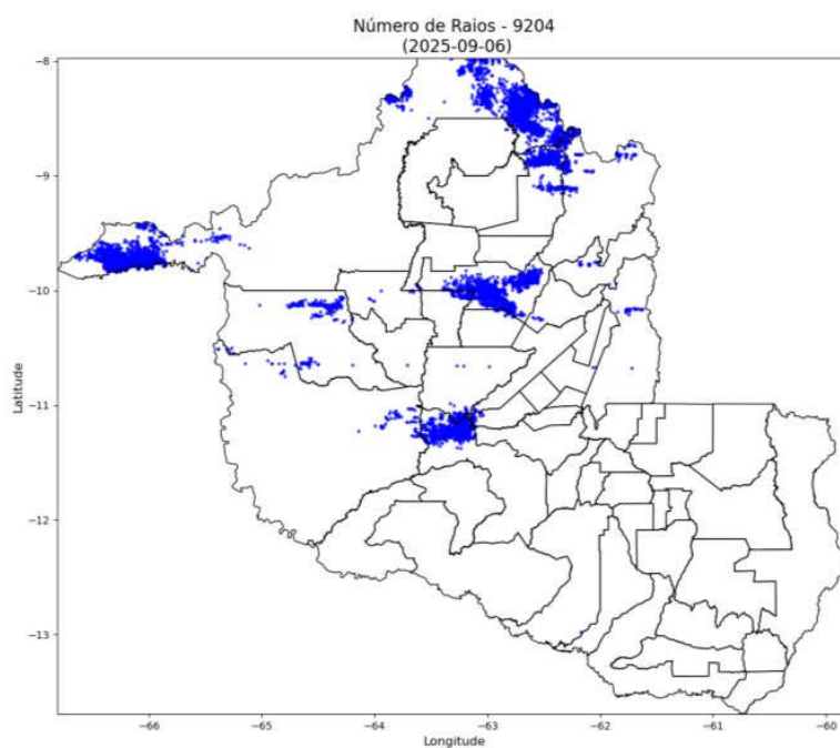
Figura 2 – Mapas de descargas atmosféricas para os dias entre 30/08 e 06/09.
