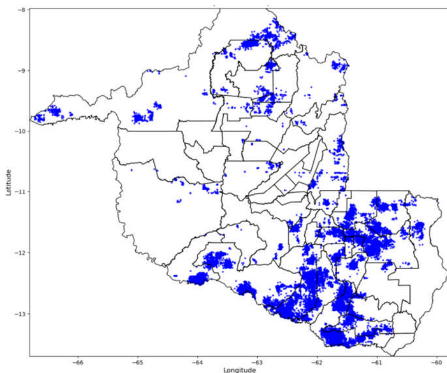
Figura 4 - Descargas Atmosféricas Observadas - 15/09/2025. Fonte: Grupo STORM
