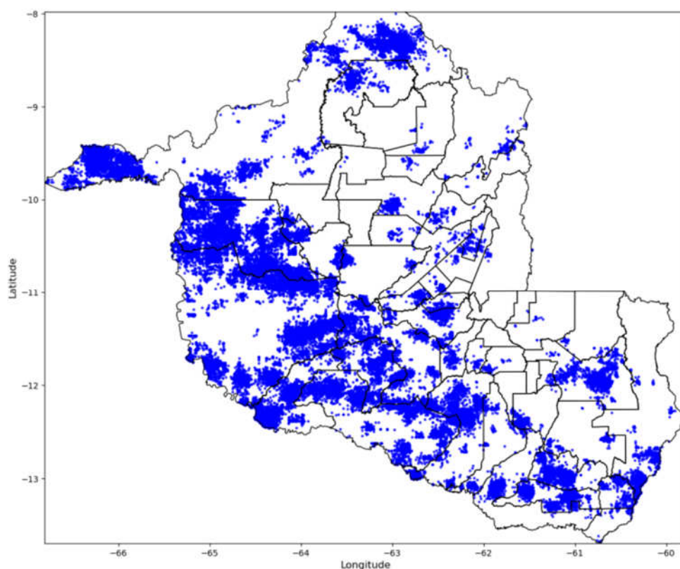
Figura 5 - Descargas Atmosféricas Observadas - 16/09/2025. Fonte: Grupo STORM
