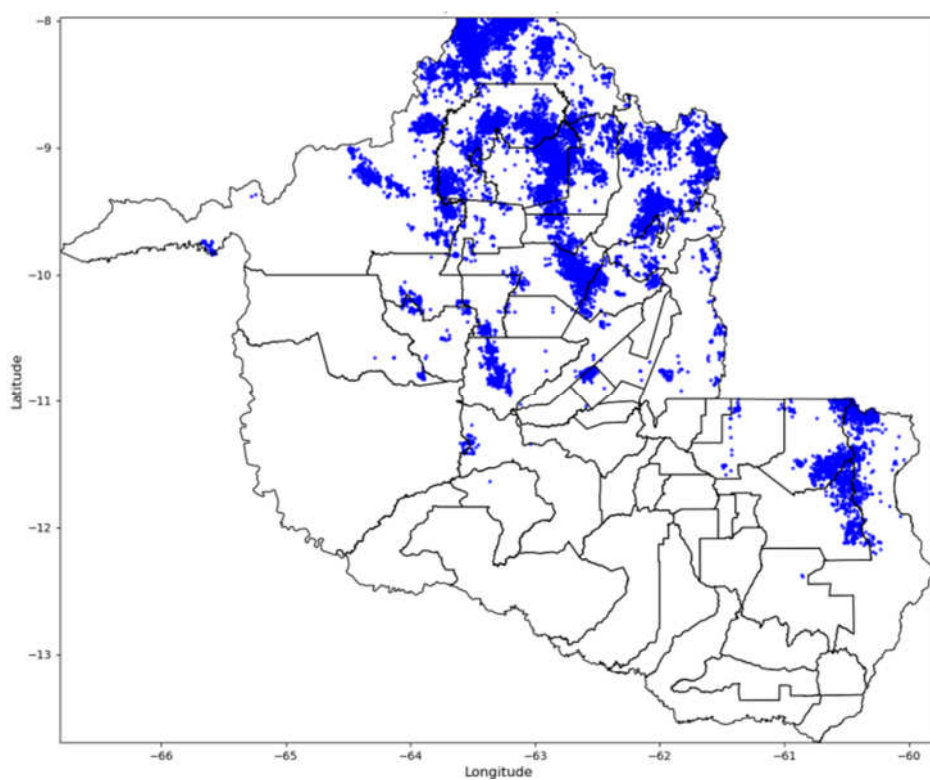
Figura 9 - Descargas Atmosféricas Observadas - 20/09/2025. Fonte: Grupo STORM
