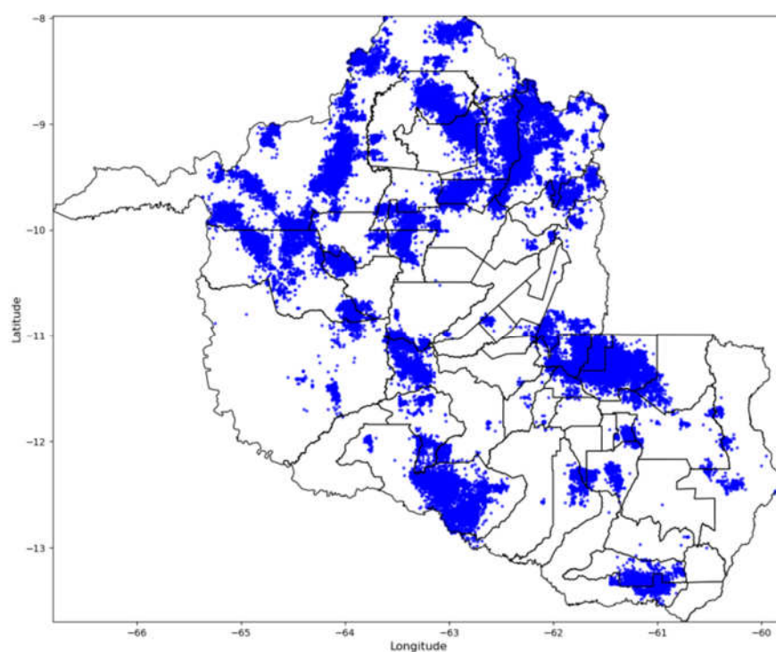
Figura 10 - Descargas Atmosféricas Observadas - 22/09/2025. Fonte: Grupo STORM
