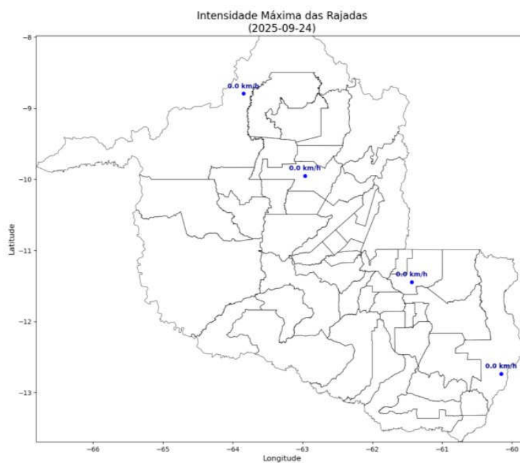
Figura 4 – Mapas de rajadas para os dias entre 15/09 e 24/09. Poucas medições.
