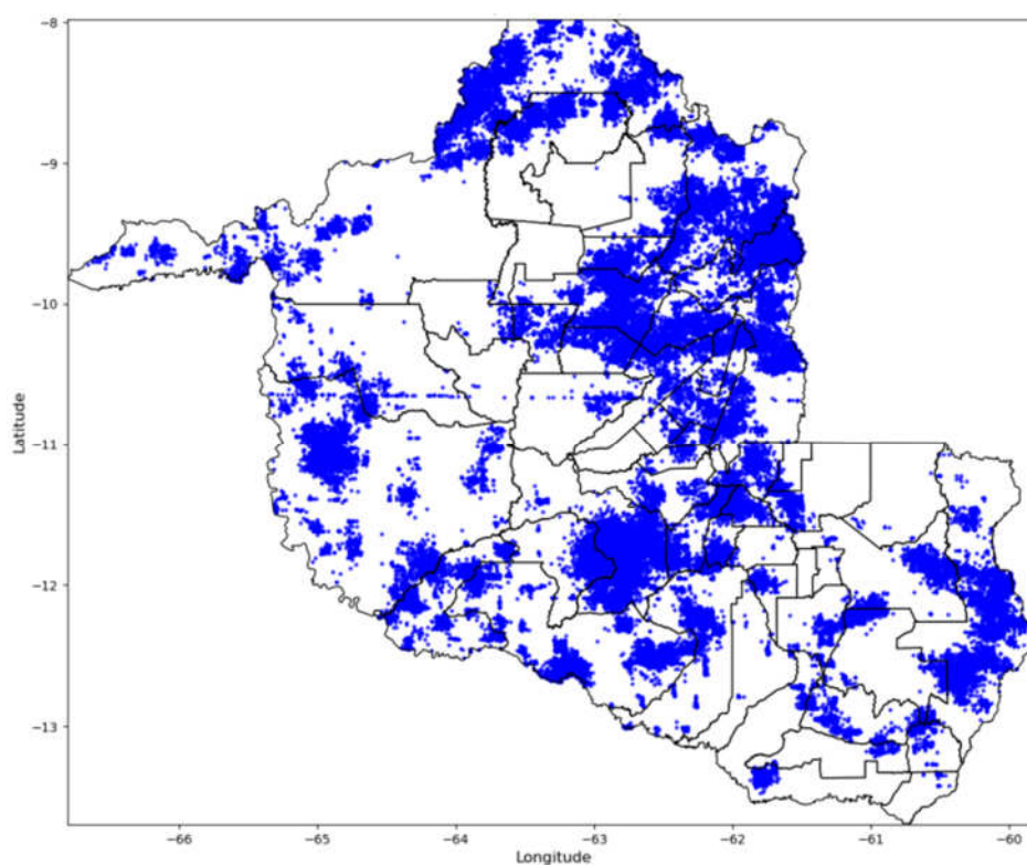
Figura 6 - Descargas Atmosféricas Observadas - 17/09/2025. Fonte: Grupo STORM
