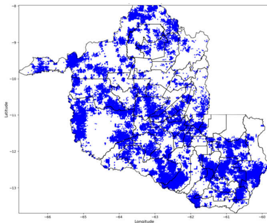
Figura 7 - Descargas Atmosféricas Observadas - 18/09/2025. Fonte: Grupo STORM
