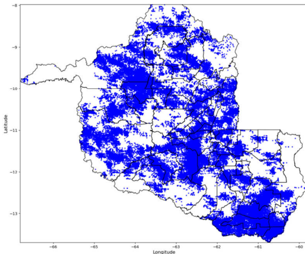
Figura 12 - Descargas Atmosféricas Observadas - 24/09/2025. Fonte: Grupo STORM
