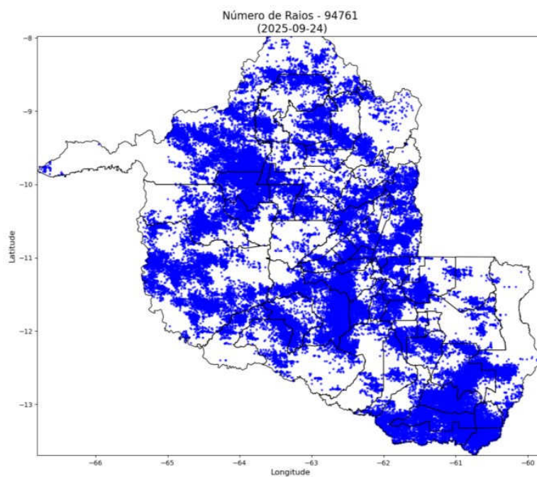
Figura 2 – Mapas de descargas atmosféricas para os dias entre 15/09 e 24/09.
