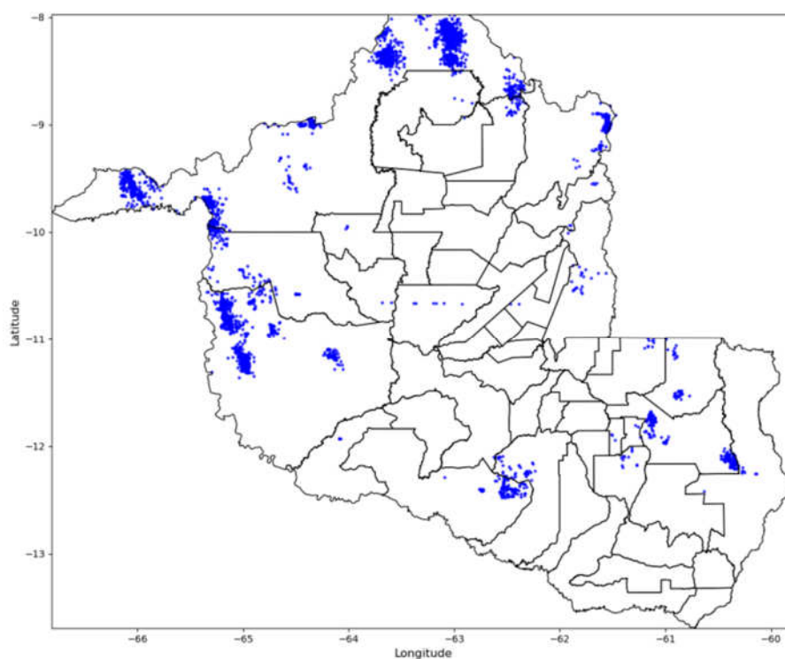
Figura 9 - Descargas Atmosféricas Observadas - 21/09/2025. Fonte: Grupo STORM
