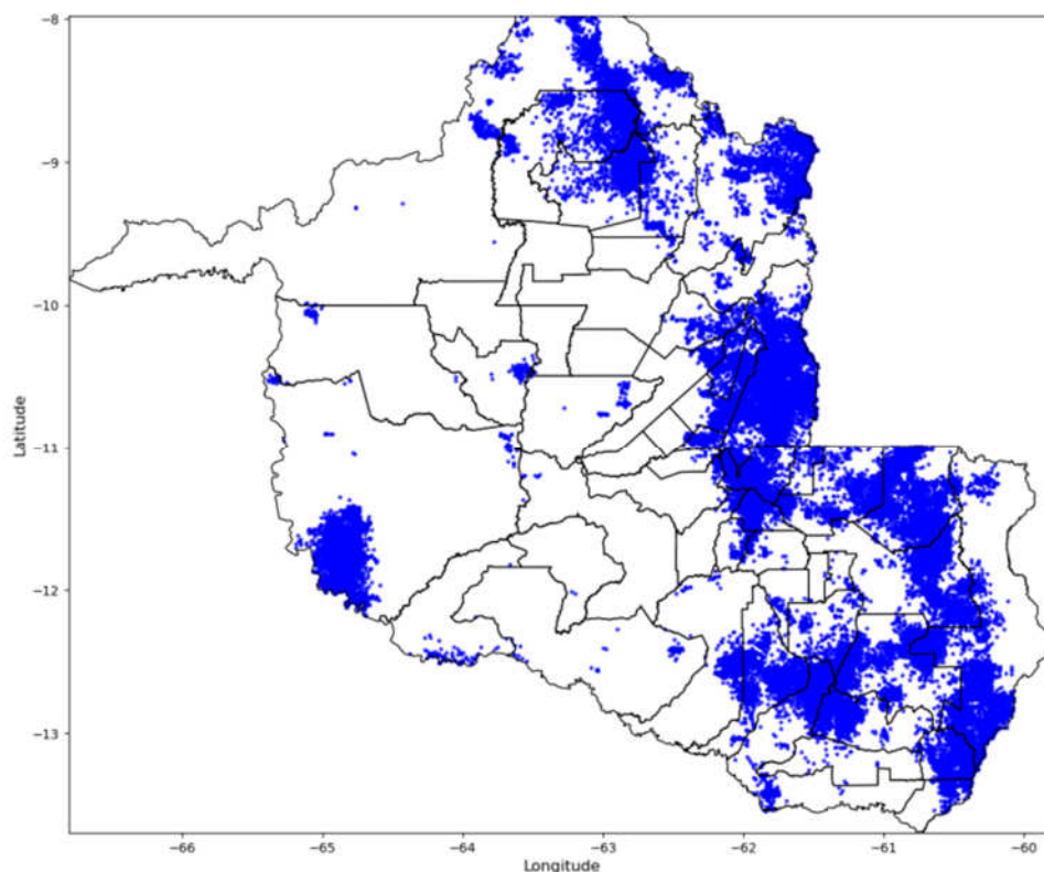
Figura 11 - Descargas Atmosféricas Observadas - 23/09/2025. Fonte: Grupo STORM
