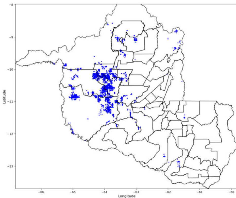
Figura 8 - Descargas Atmosféricas Observadas - 19/09/2025. Fonte: Grupo STORM
