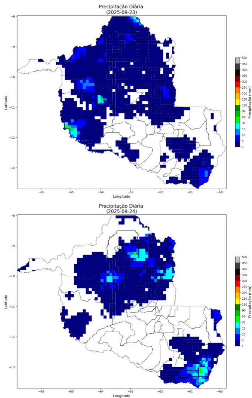
Figura 3 – Mapas de precipitação para os dias entre 15/09 e 24/09.
