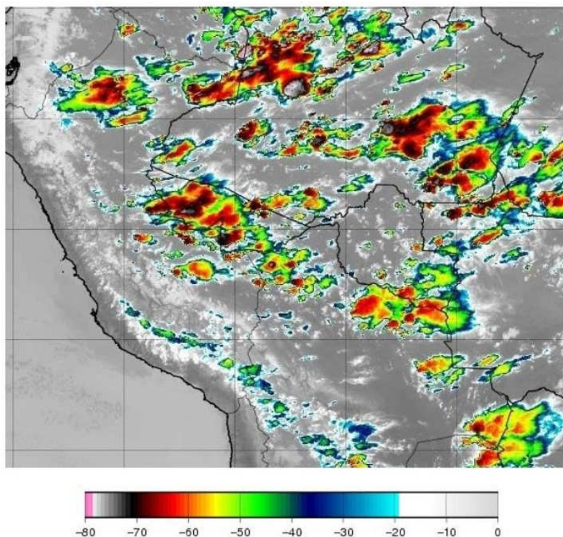
Figura 1 - Imagens de satélite no infravermelho com realce do satélite GOES-19 às 21:00 UT do dia 15/09. As cores indicam diferentes temperaturas dos topos das nuvens.
