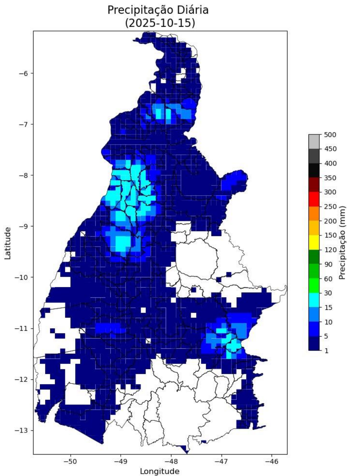
Figura 3 – Mapa de precipitação acumulada para os dias: 07 a 15/10.
