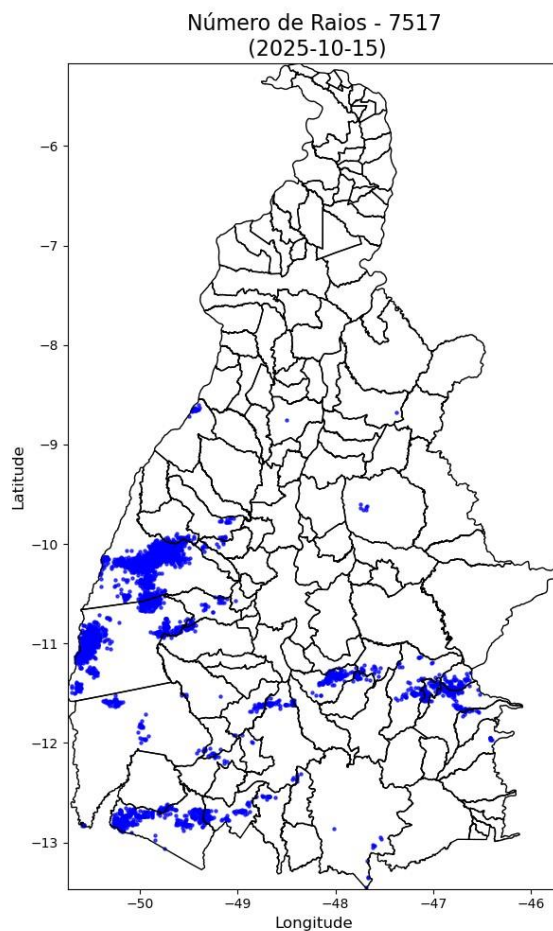
Figura 2 – Mapa de descargas atmosféricas para os dias 07 a 15/10.
