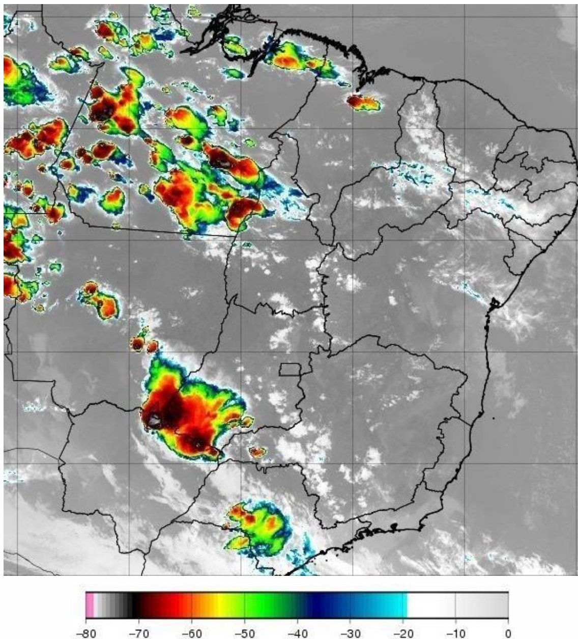
Figura 1 - Imagem de satélite no infravermelho com realce do satélite GOES-16 às 21:00 UT do dia 07/10. As cores indicam diferentes temperaturas dos topos das nuvens.
