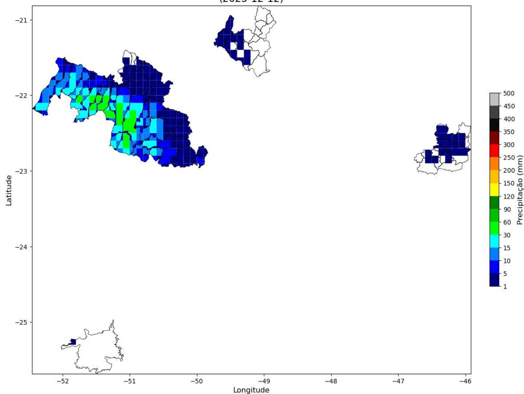
Precipitação Diária (2025-12-12)
