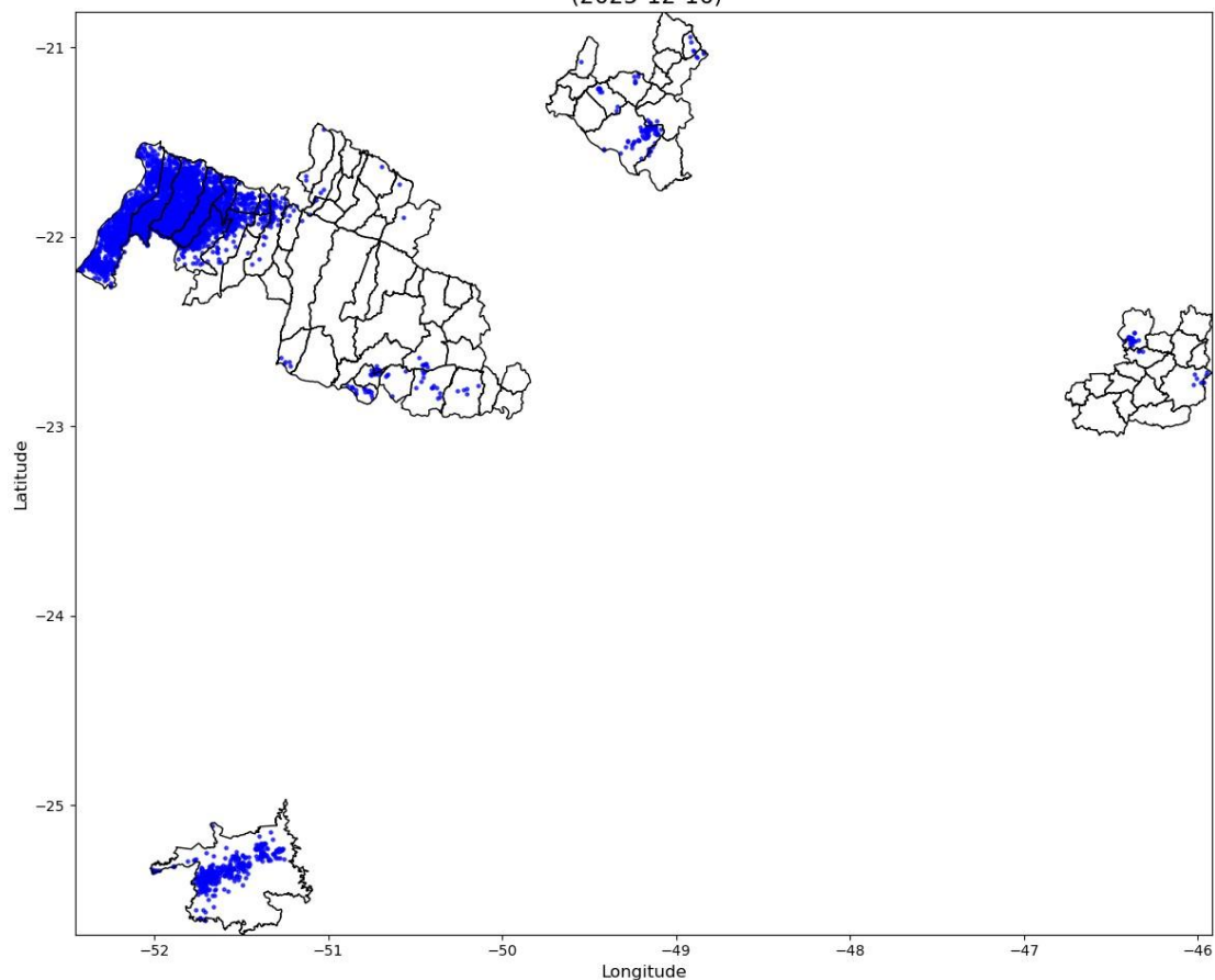
Número de Raios - 8825 (2025-12-16)
