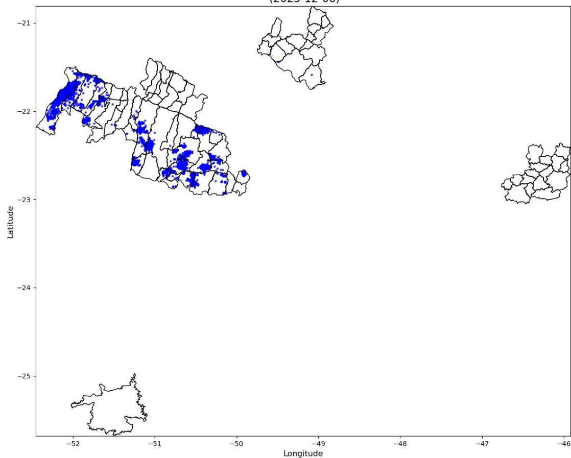
Número de Raios - 7231 (2025-12-06)
