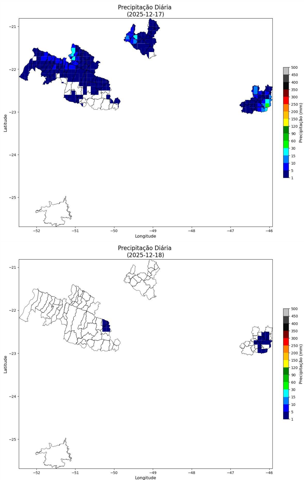
Figura 3 – Mapa de precipitação para os dias de 05 a 18/12.
