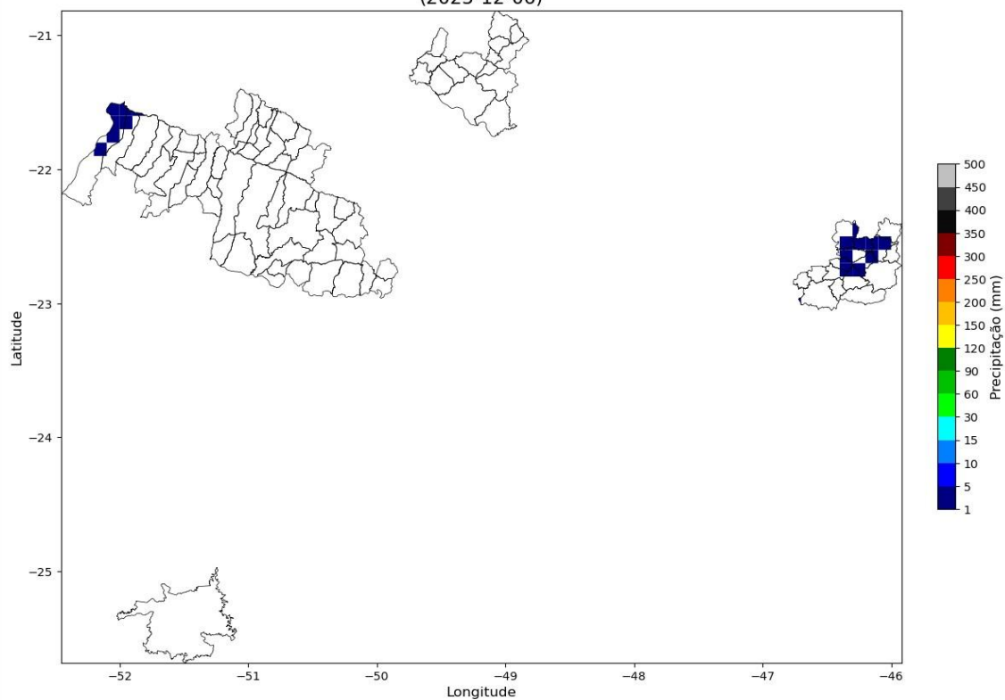
Precipitação Diária (2025-12-06)
