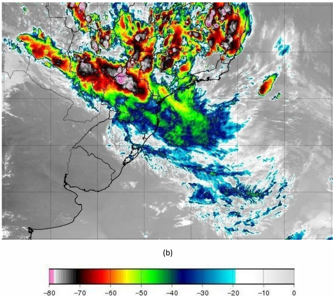
Figura 1 - Imagem de satélite no infravermelho com realce do satélite GOES-19 para as 21:00 UT do dia (a) 05/12 e (b) 12/12. As cores indicam diferentes temperaturas dos topos das nuvens.
