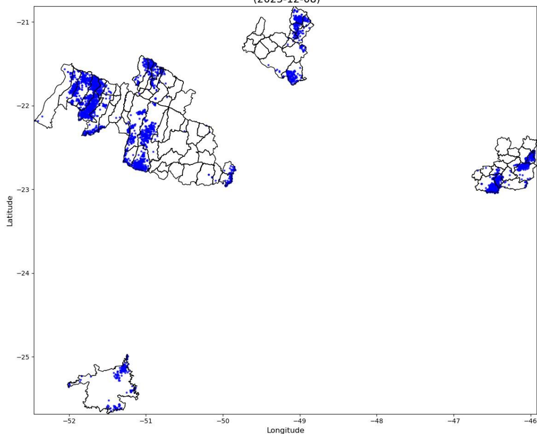
Número de Raios - 4938 (2025-12-08)
