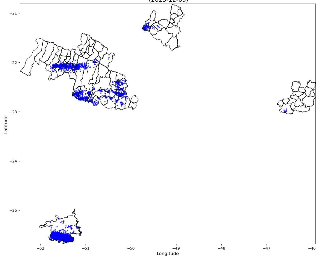
Número de Raios - 5321 (2025-12-09)
