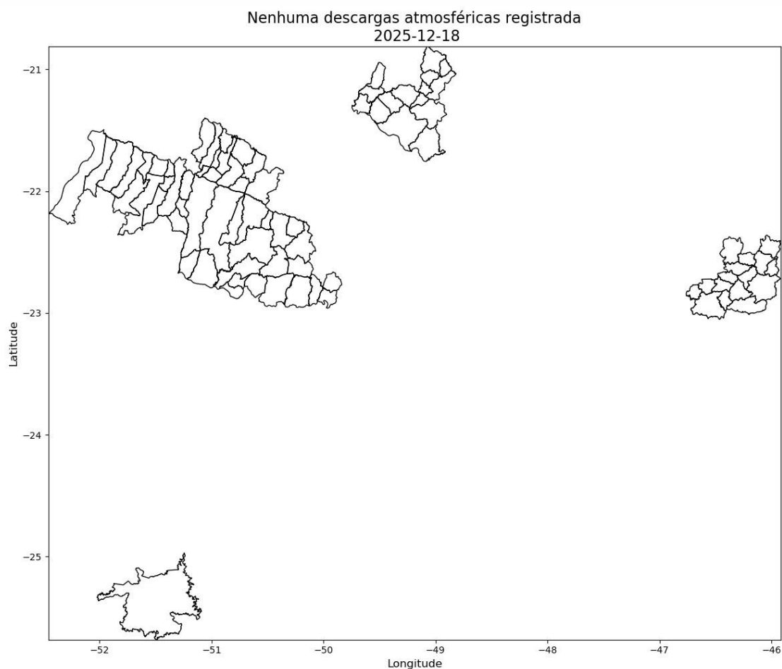
Figura 2 – Mapa de incidência de descargas atmosféricas nuvem-solo e intranuvem para os dias 05 a 18/12. Cada ponto corresponde ao local de ocorrência de uma descarga.
