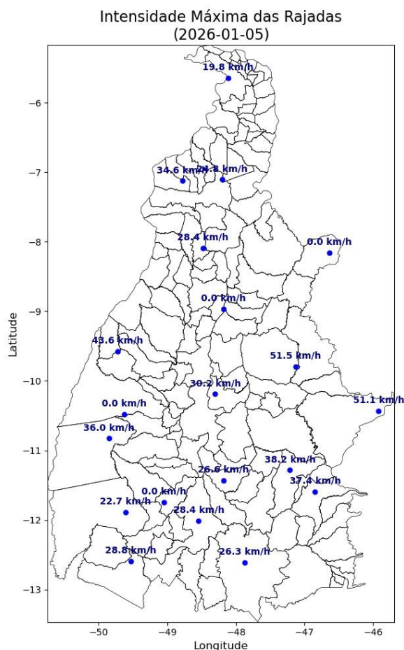
Figura 4 – Mapa da intensidade máxima das rajadas para os dias 23/12 a 05/01.
