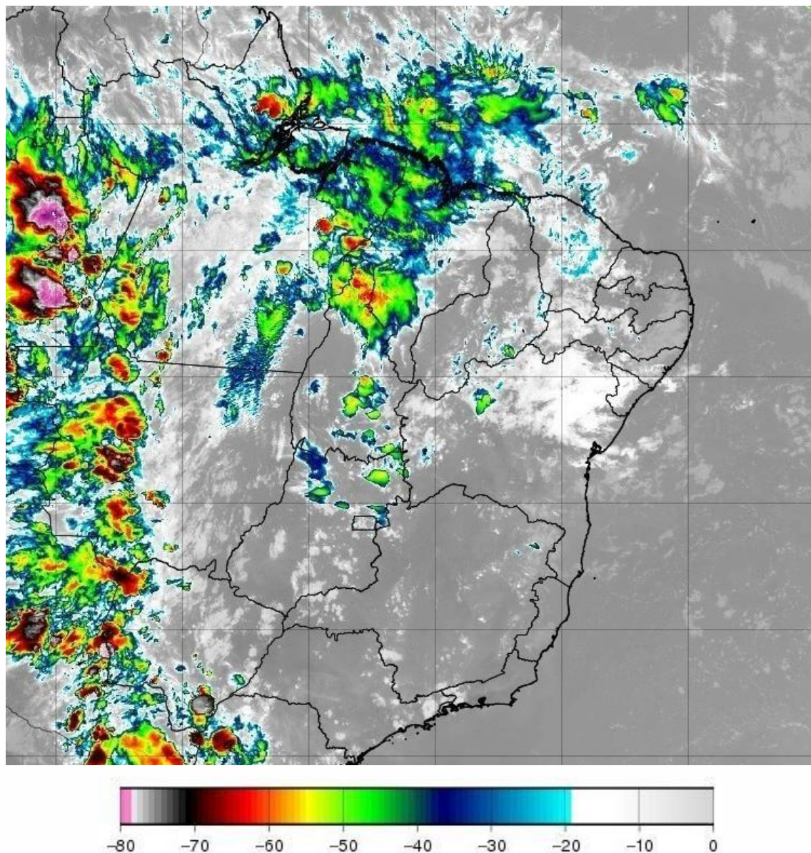
Figura 1 - Imagem de satélite no infravermelho com realce do satélite GOES-19 às 21:00 UT do dia 23/12. As cores indicam diferentes temperaturas dos topos das nuvens. Diferentes cores na imagem na Figura 1 referem-se a diferentes temperaturas de topo das nuvens, conforme indicado na figura, e equivalem a diferentes altitudes. Quanto
