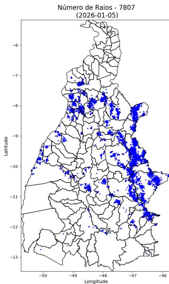
Figura 2 – Mapa de descargas atmosféricas para os dias 23/12 a 05/01.
