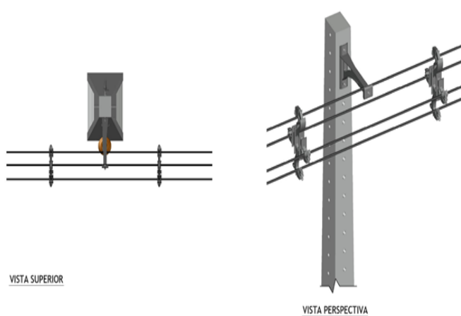
Estrutura CE 1
