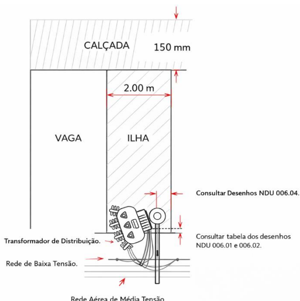
Figura 08. Dimensionamento da ilha para instalação de transformador ao lado de vagas.
