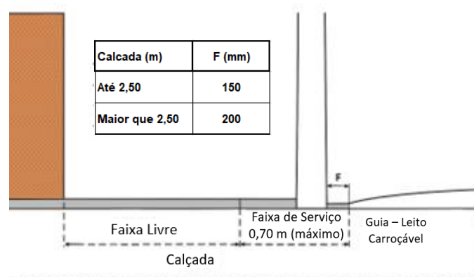
Figura 01. Distância entre postes e meio-fio da rede de distribuição.
