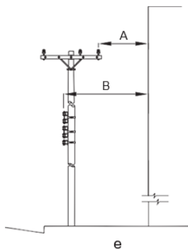
Afastamento horizontal entre os condutores e a parede de edificações
