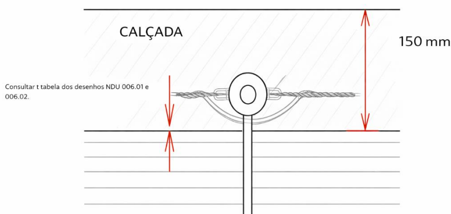
Figura 09. Locação de postes em calçadas.
