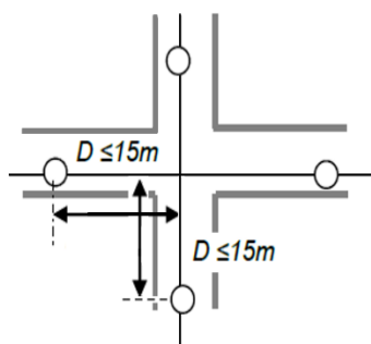
Figura 04. Cruzamento aéreo.
