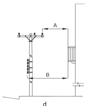
Afastamento horizontal entre os condutores e o piso da sacada, terraço e janela das edificações
