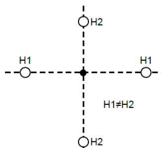
Figura 05. Cruzamento Aéreo - Rede aérea convencional.
