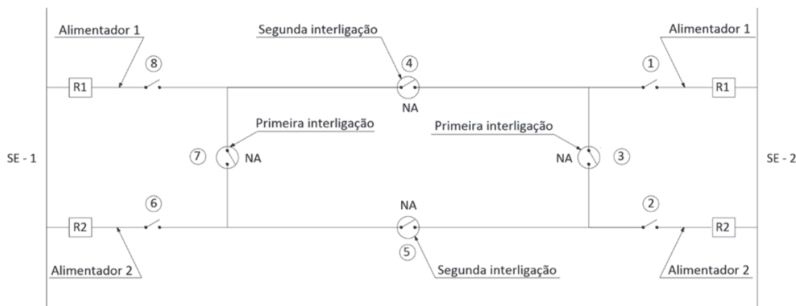
Figura 15 - Interligação de alimentadores.
