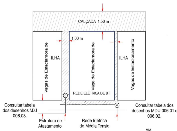
Figura 07. Locação de postes ao lado de vagas de estacionamento.
