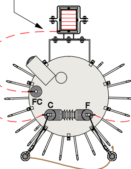
FC ATERRADO
