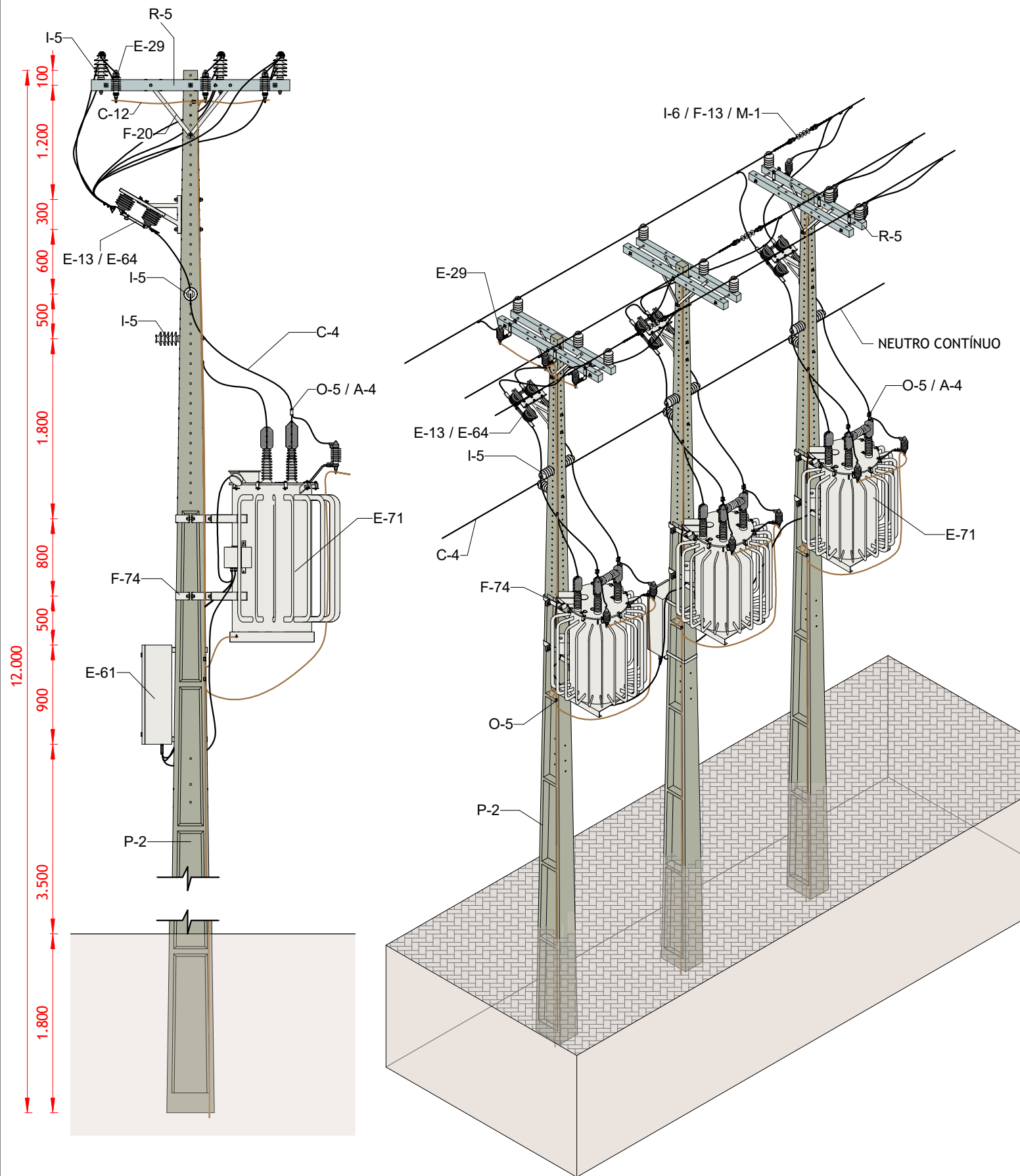
VISTA LATERAL
