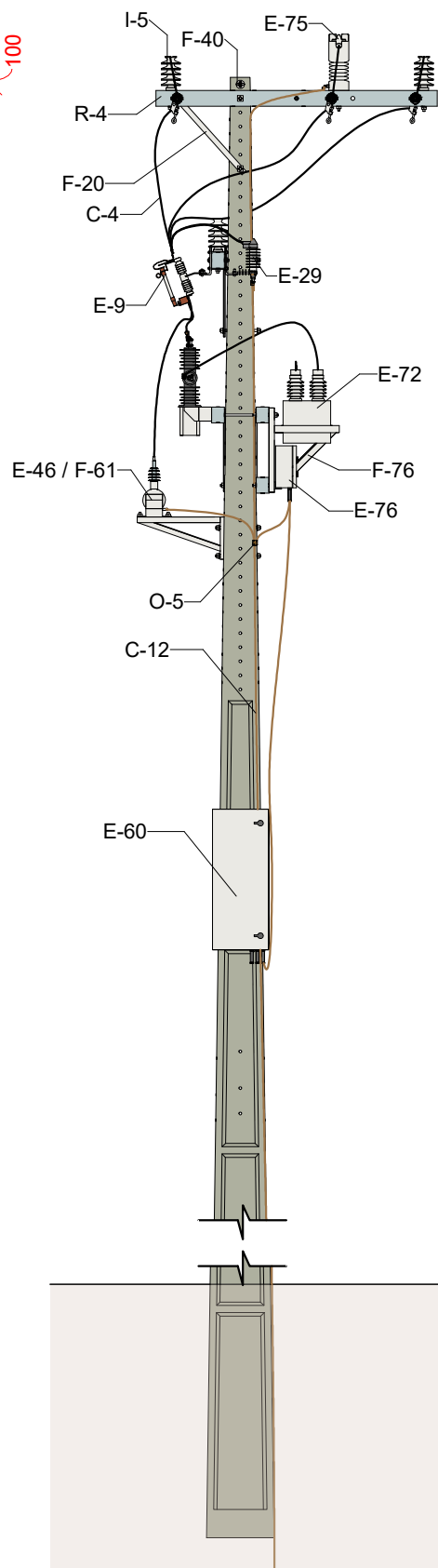
VISTA LATERAL 1 : 50
