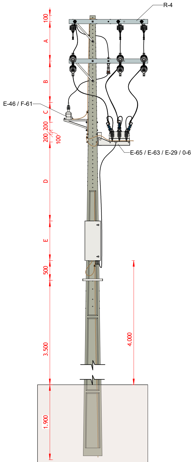
VISTA LATERAL 1 : 50
