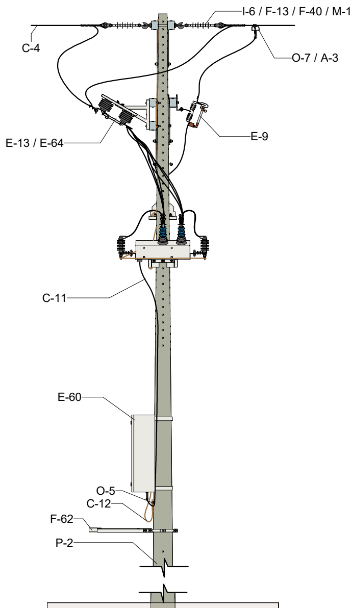
VISTA FRONTAL 1 : 50
