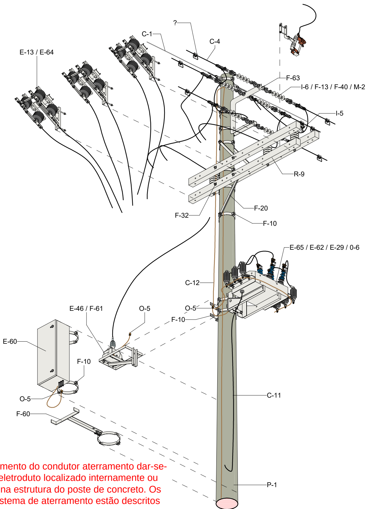
DETALHE MONTAGEM
