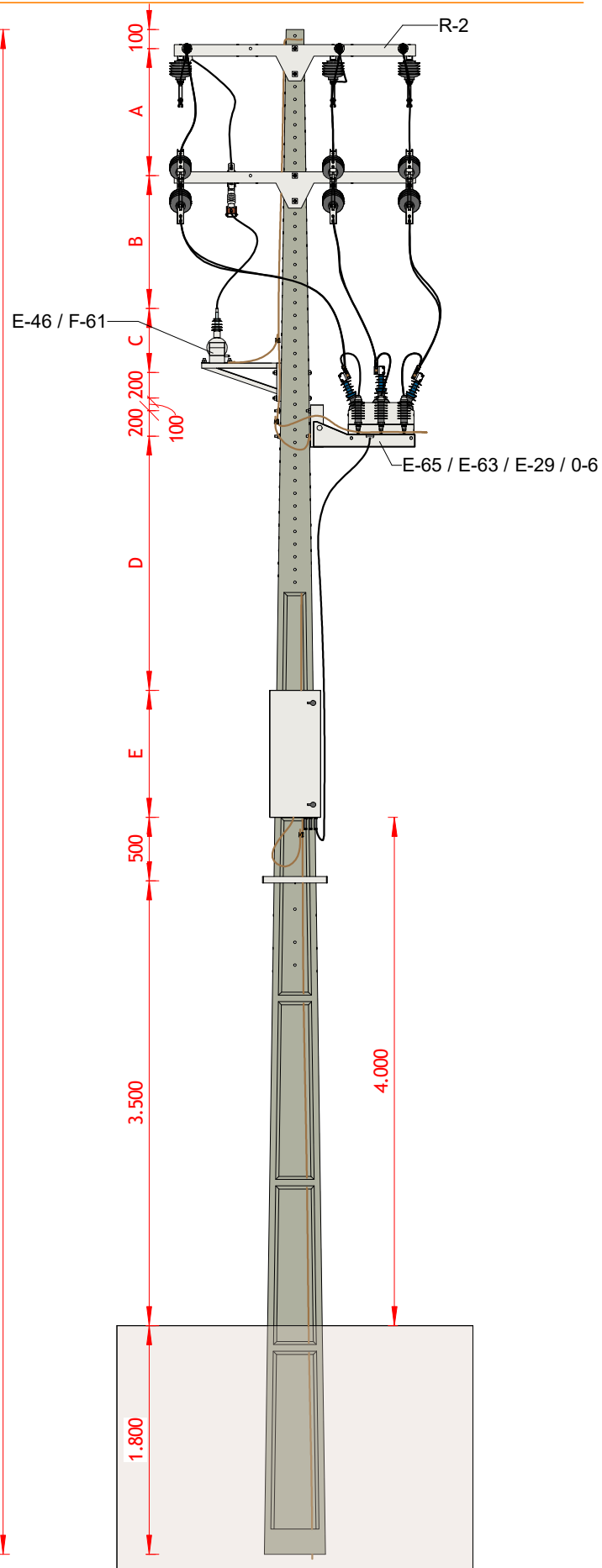
VISTA LATERAL
