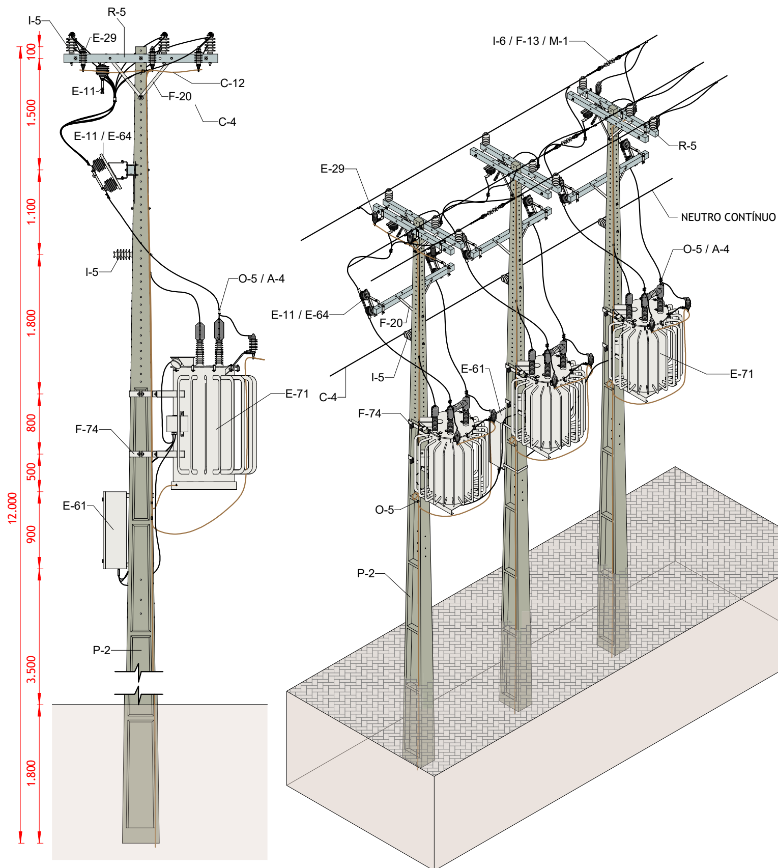
VISTA LATERAL
