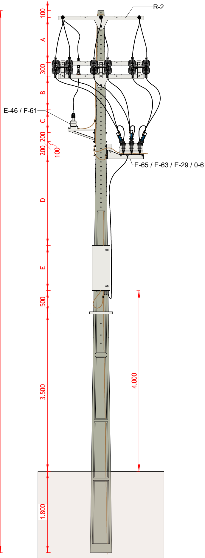
VISTA LATERAL
