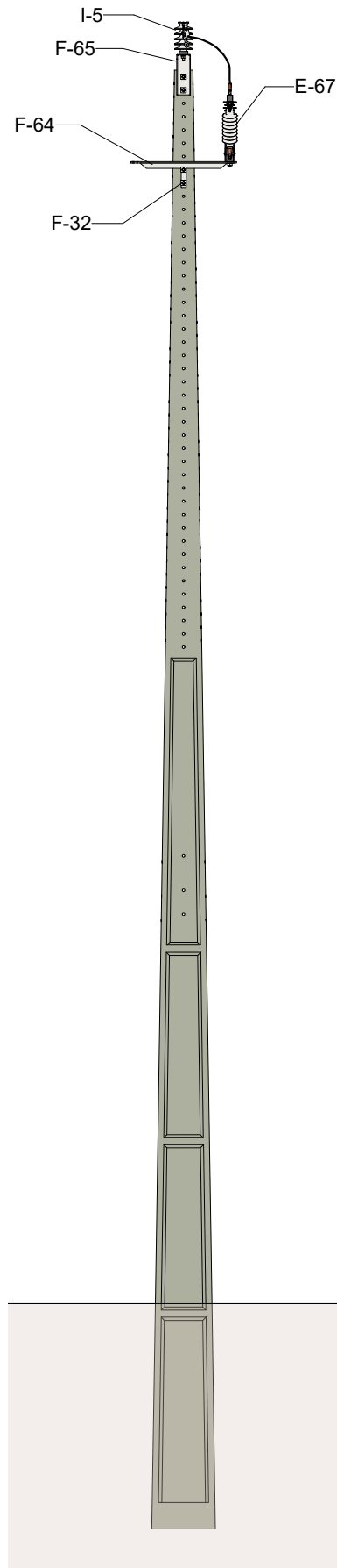
VISTA LATERAL 1 : 50
