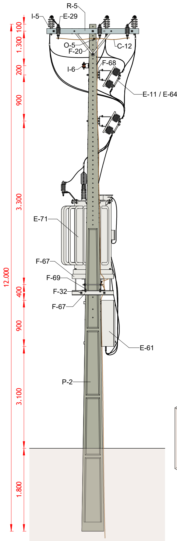
VISTA LATERAL
