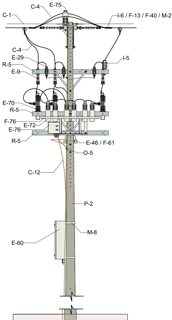
VISTA FRONTAL 1 : 50
