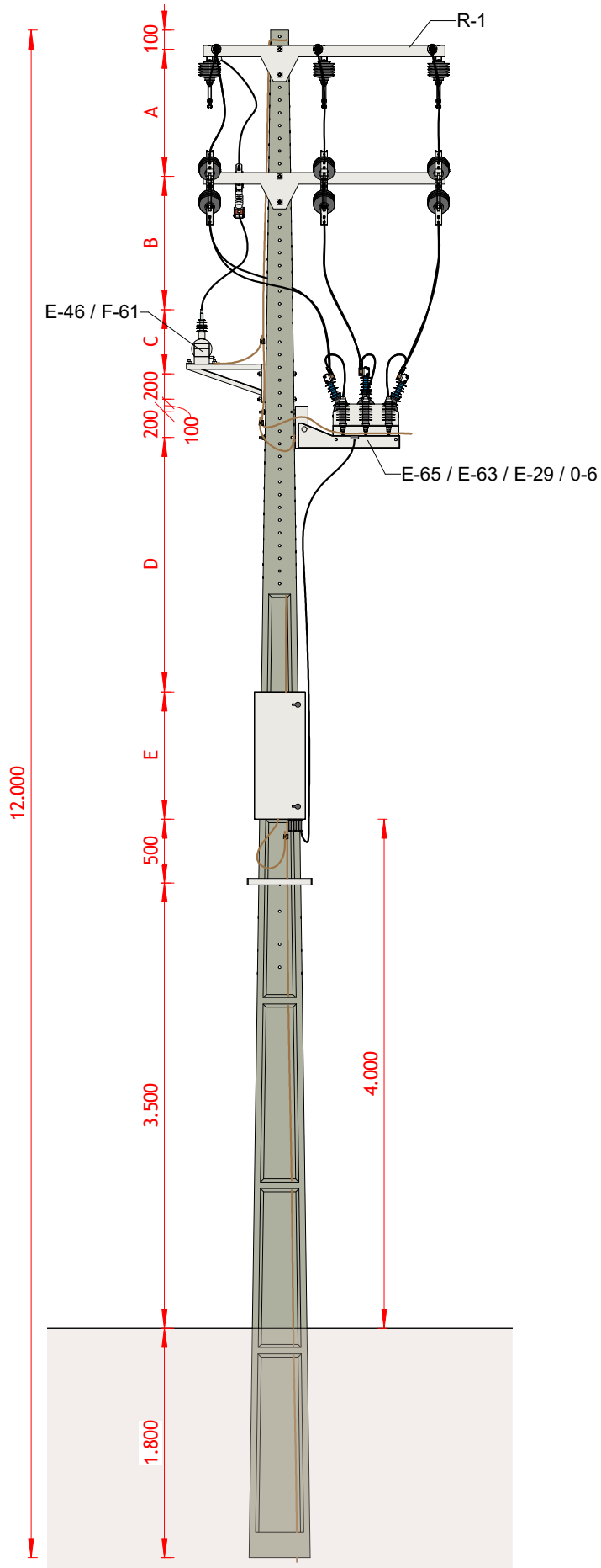
VISTA LATERAL
