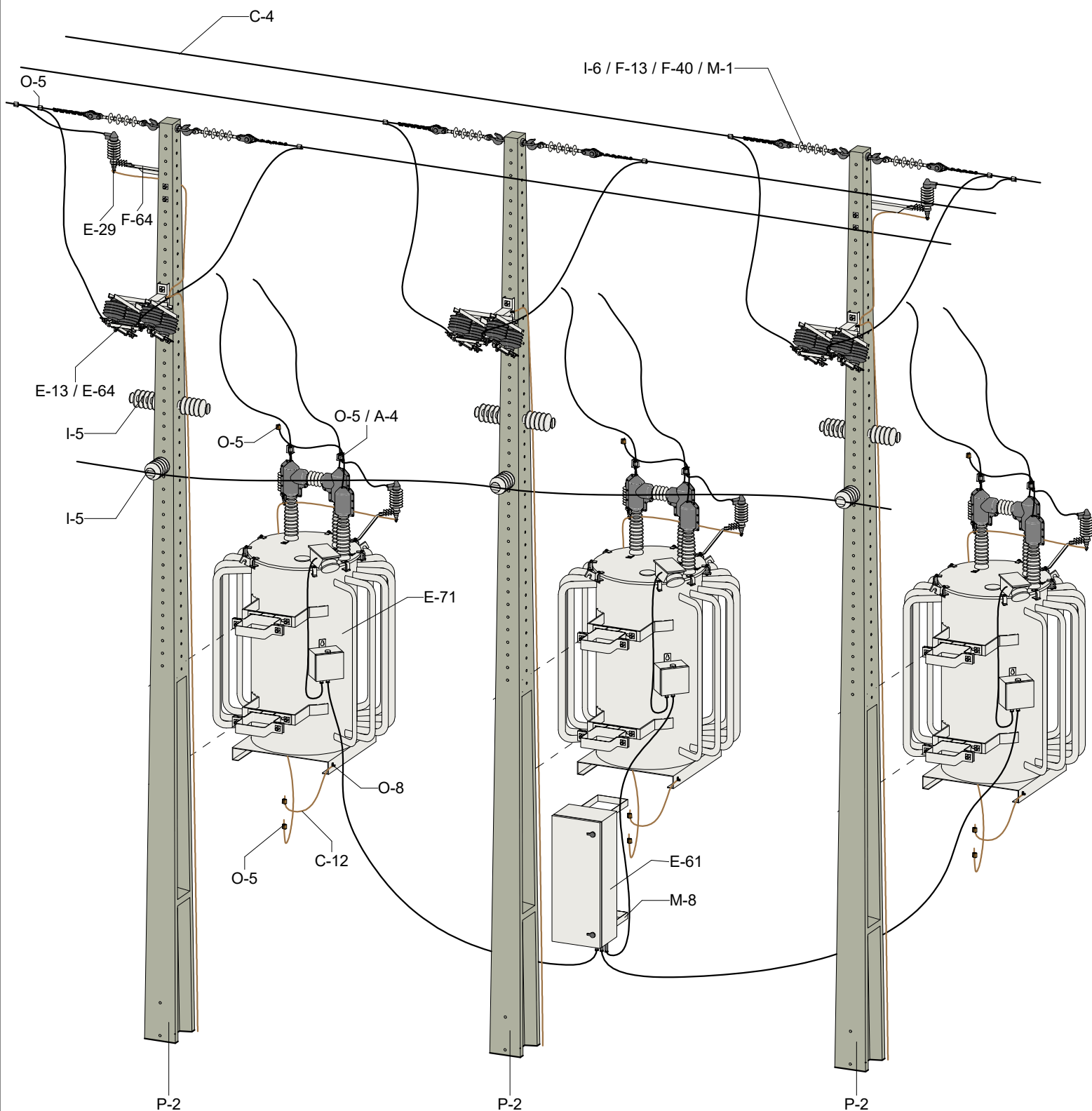
DETALHE MONTAGEM
