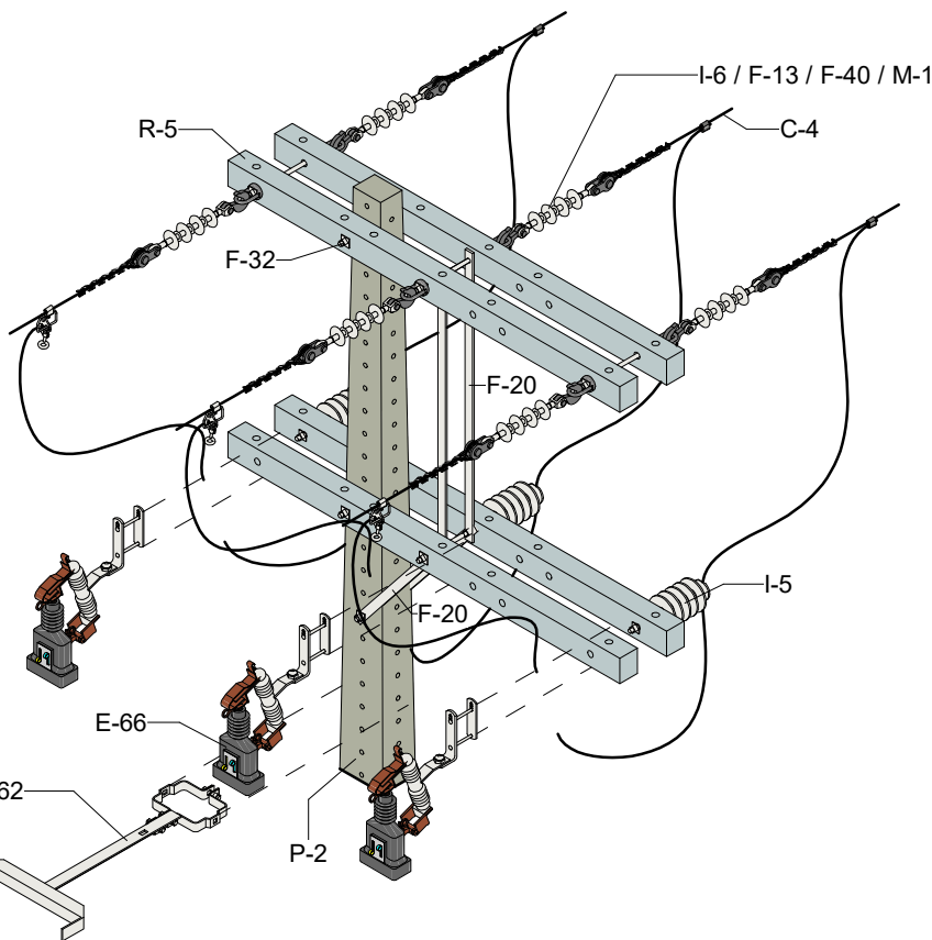
DETALHE MONTAGEM
