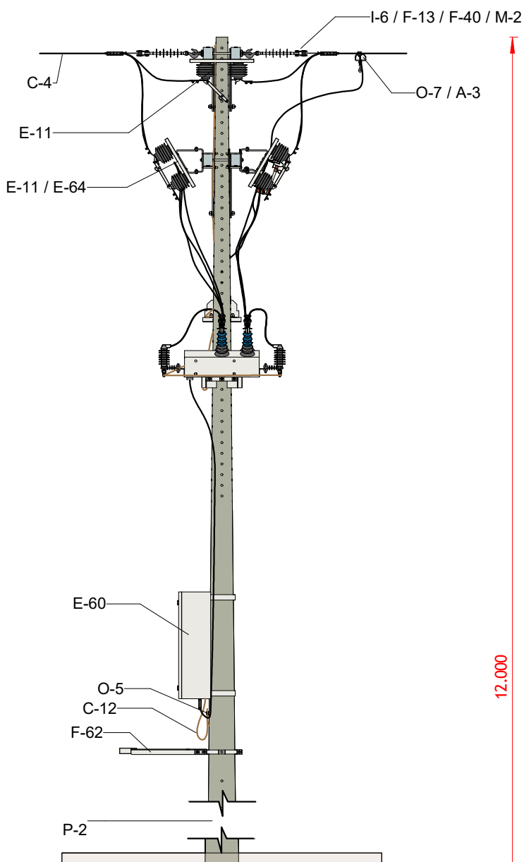
VISTA FRONTAL 1 : 50
