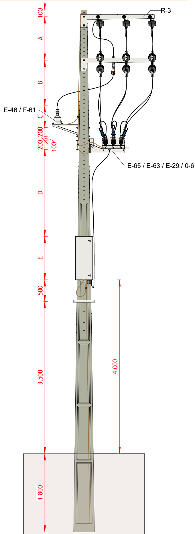
VISTA LATERAL
