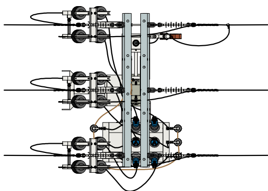
VISTA SUPERIOR 1 : 50
