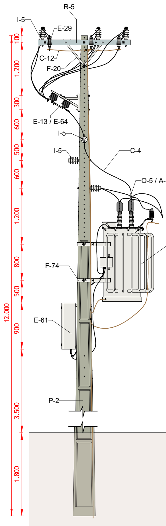
VISTA LATERAL
