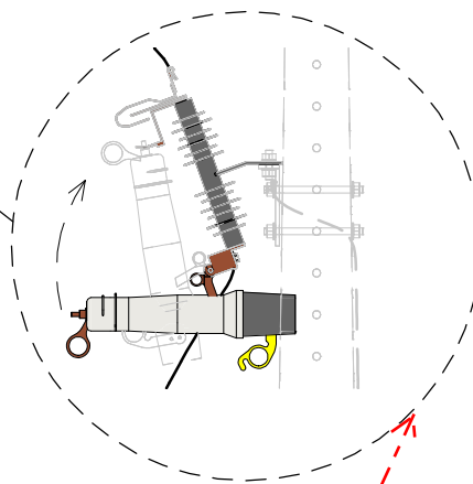
DET. DESARMADO
