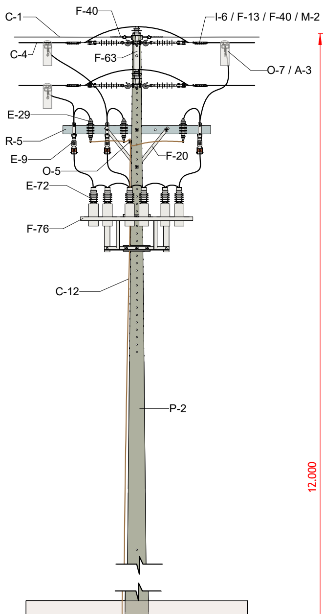
VISTA FRONTAL 1 : 50
