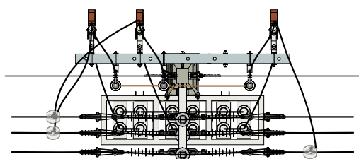
VISTA SUPERIOR 1 : 50
