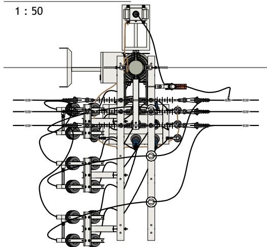
VISTA SUPERIOR 1 : 50
