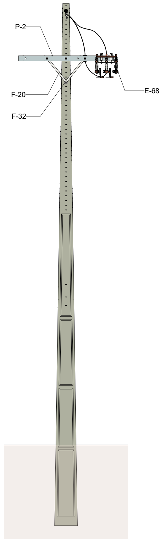
VISTA LATERAL 1 : 50
