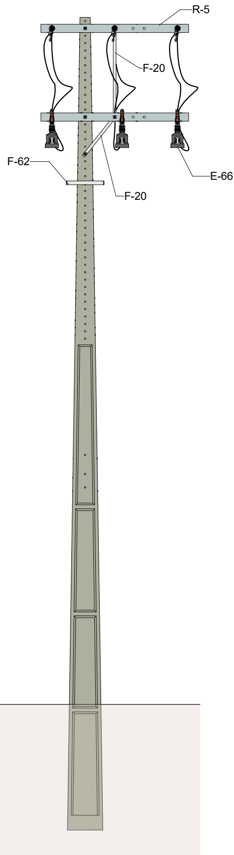
VISTA LATERAL
