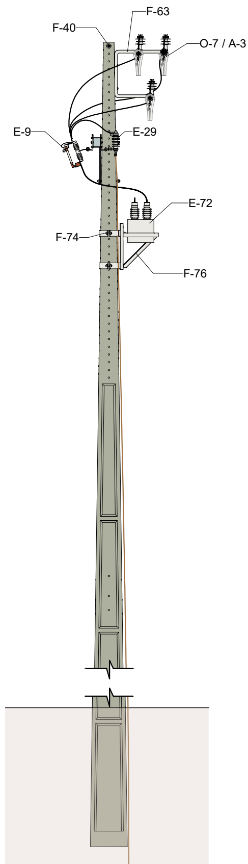
VISTA LATERAL 1 : 50
