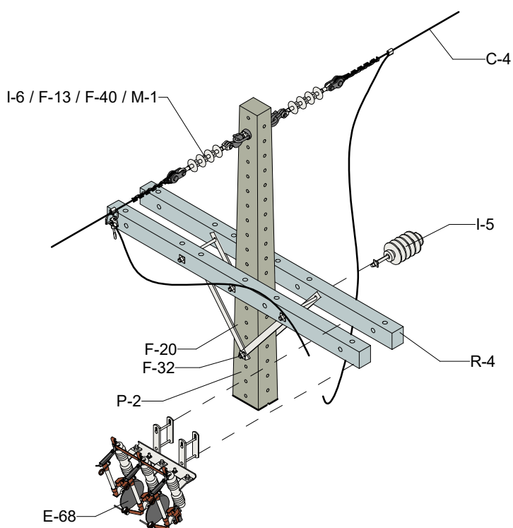
DETALHE MONTAGEM
