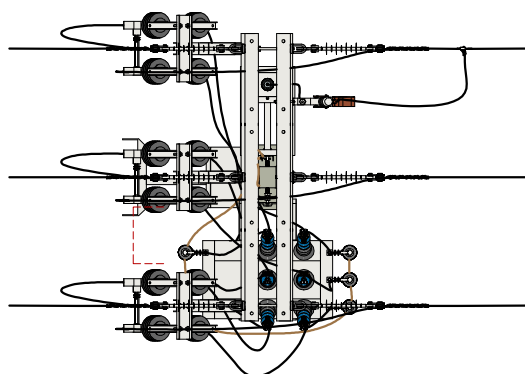
VISTA SUPERIOR
