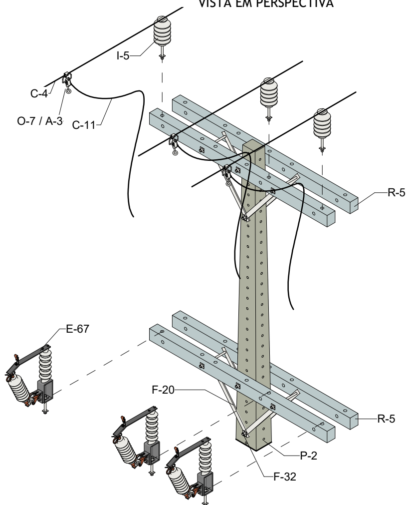
DETALHE MONTAGEM
