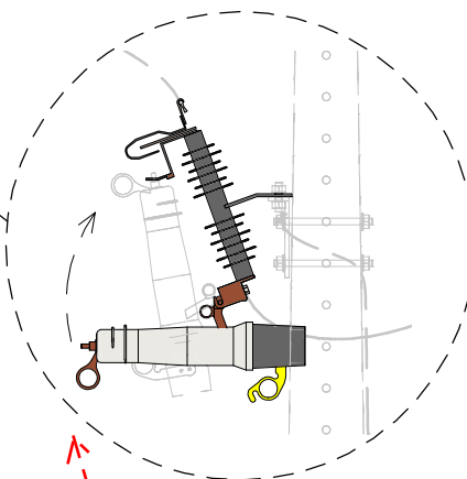
DET. DESARMADO 1 : 20
