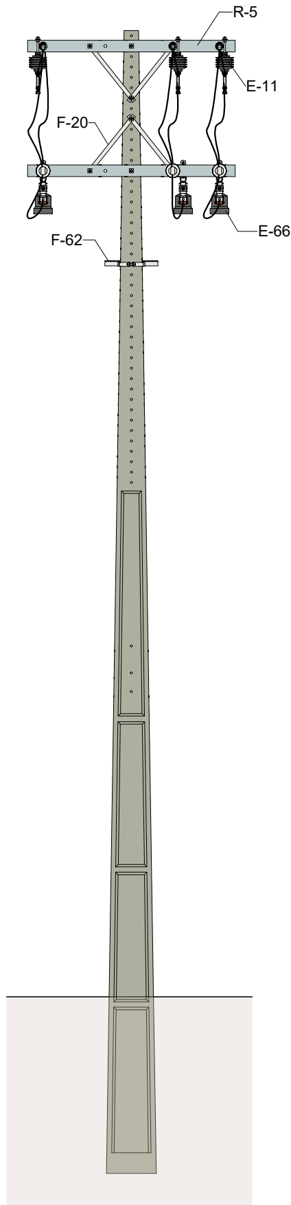
VISTA LATERAL
