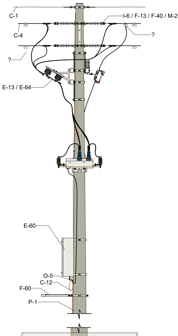
VISTA FRONTAL 1 : 50
