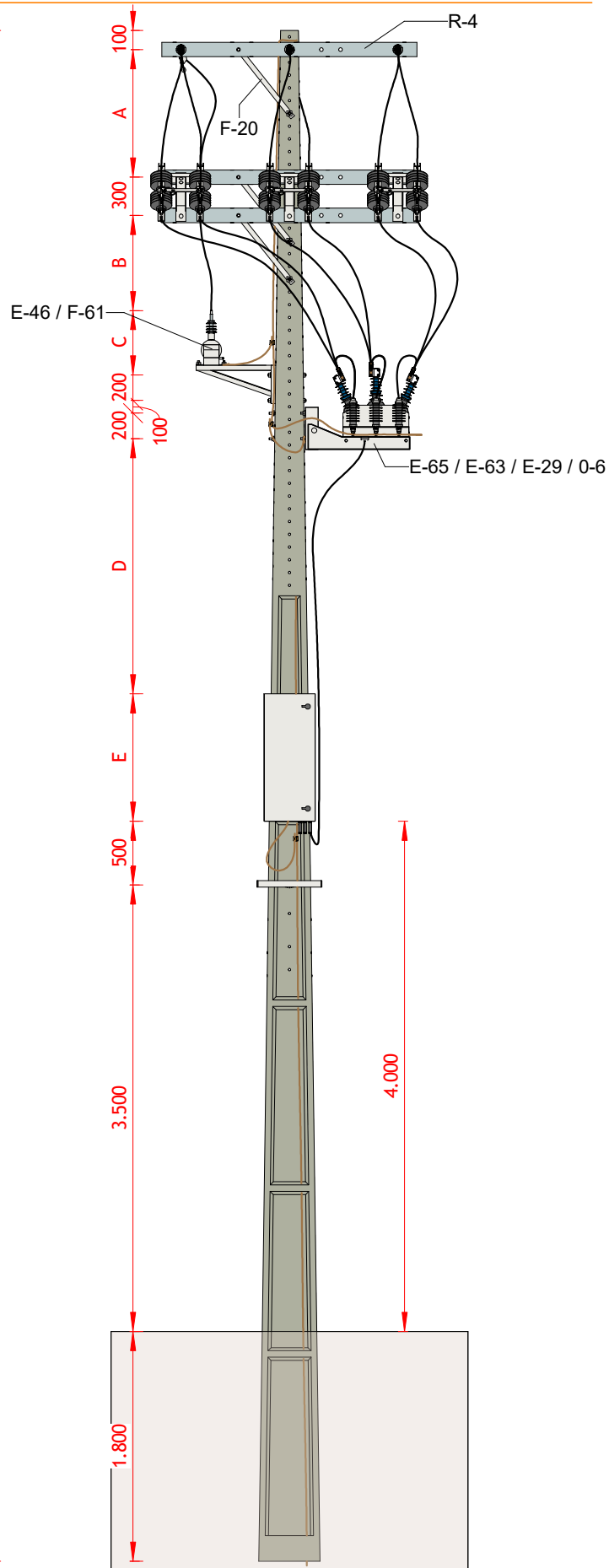
VISTA LATERAL 1 : 50
