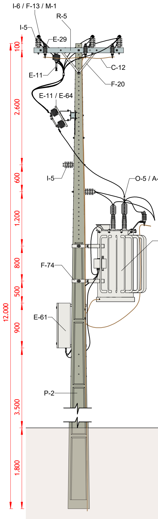
VISTA LATERAL
