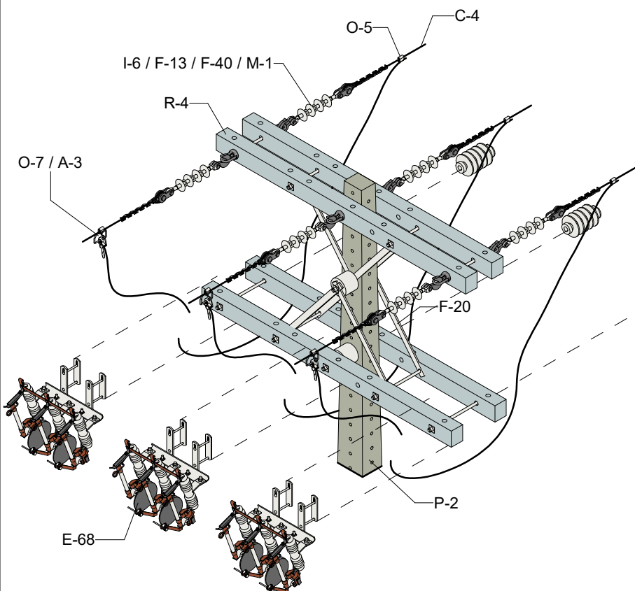
DETALHE MONTAGEM
