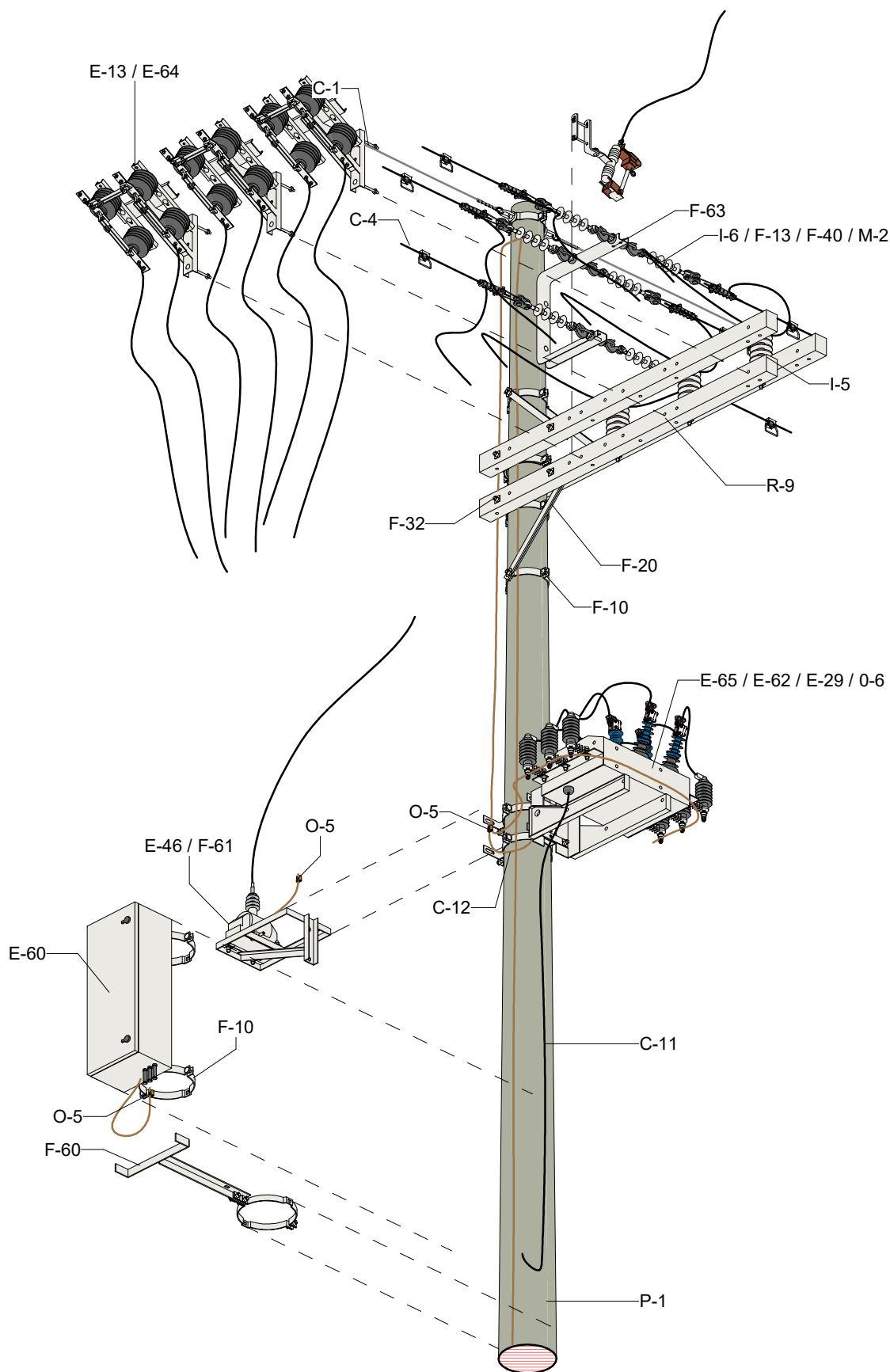
DETALHE MONTAGEM
