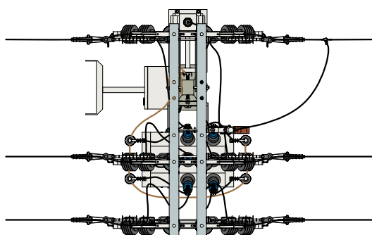
VISTA SUPERIOR 1 : 50
