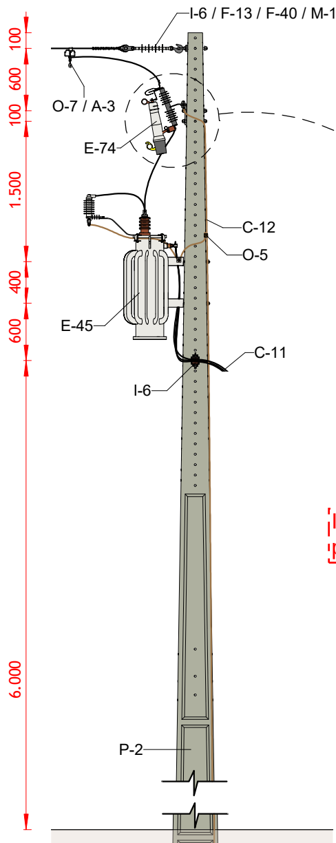
VISTA LATERAL
