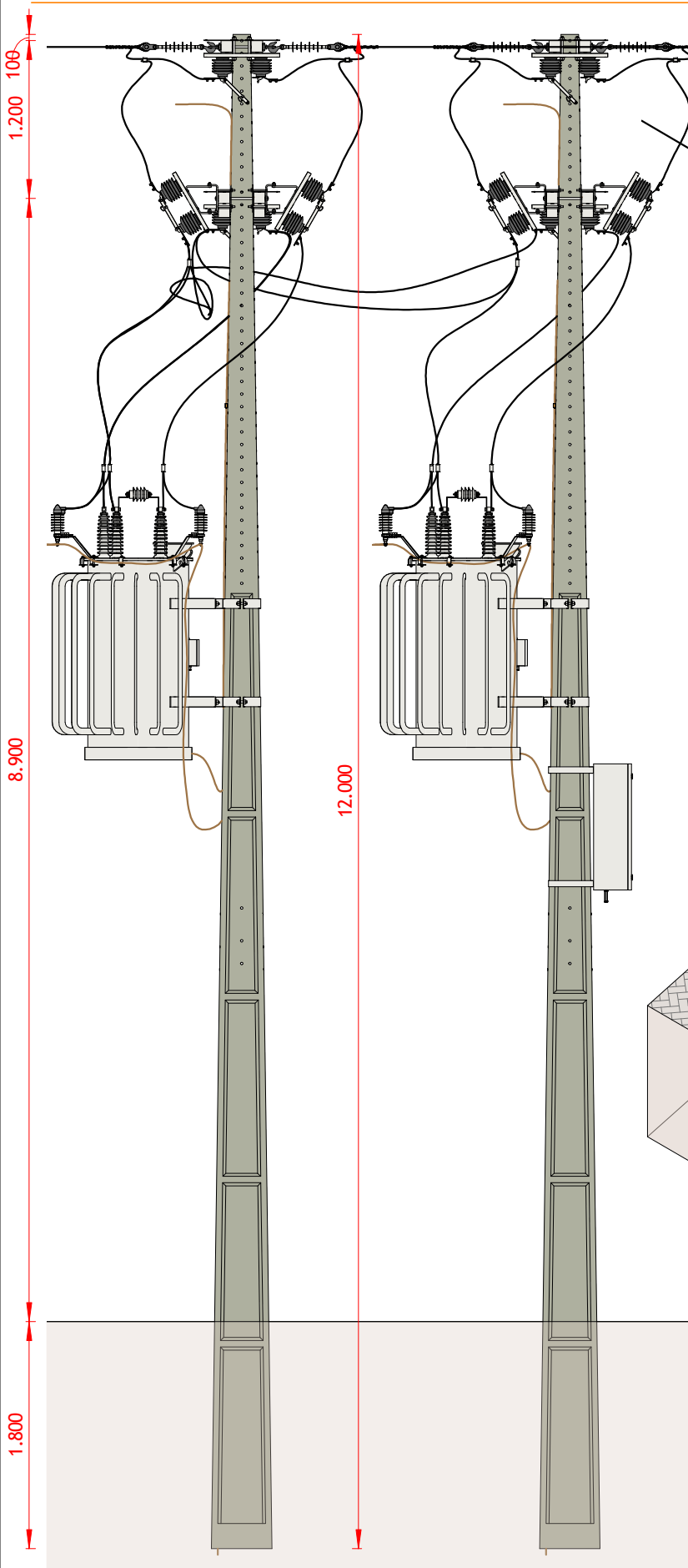
VISTA LATERAL
