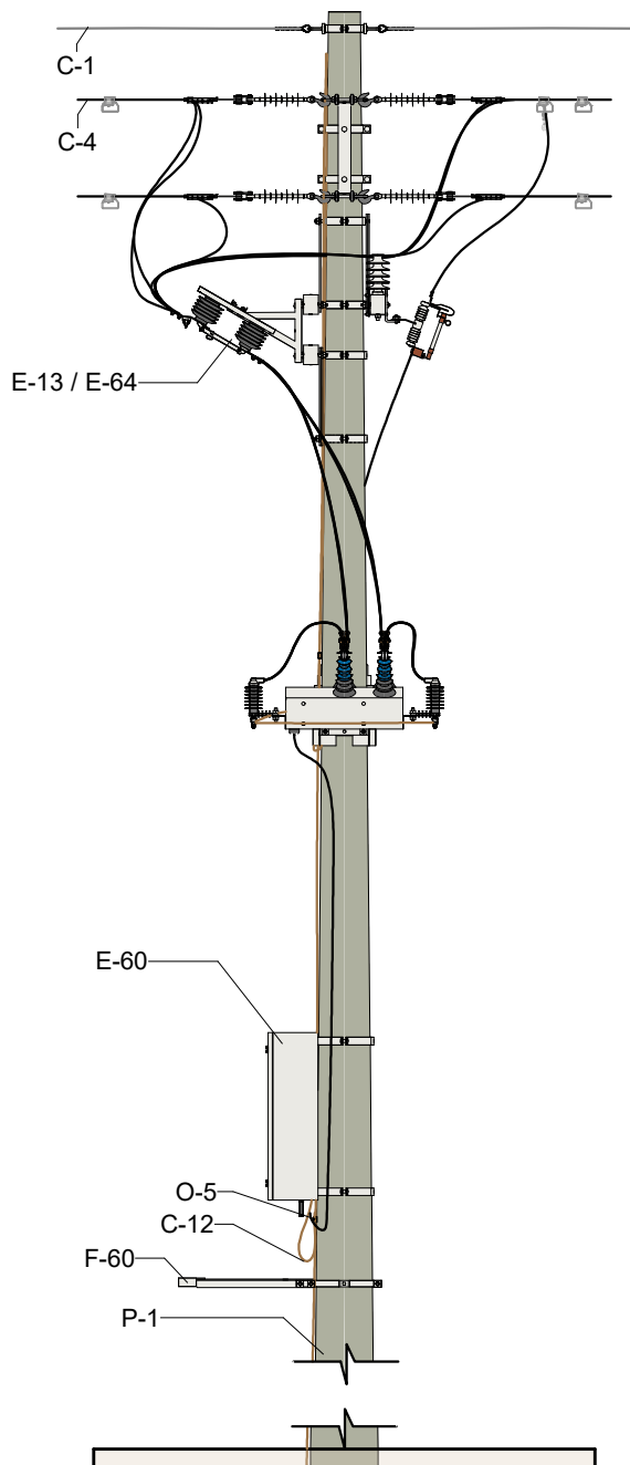
VISTA FRONTAL 1 : 50
