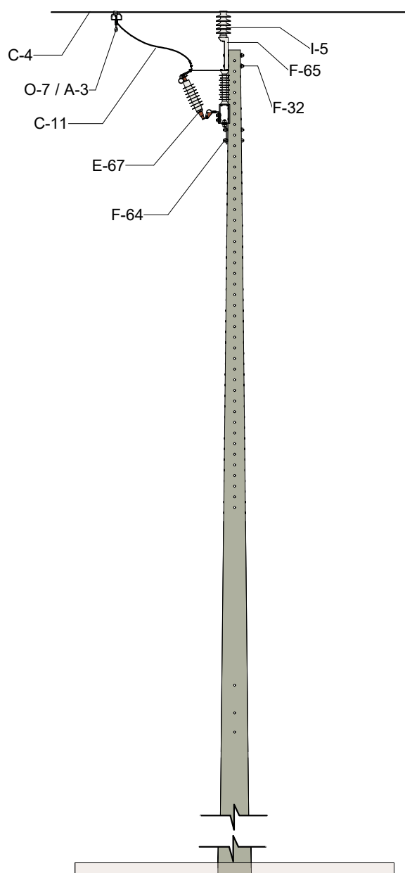
VISTA FRONTAL 1 : 50
