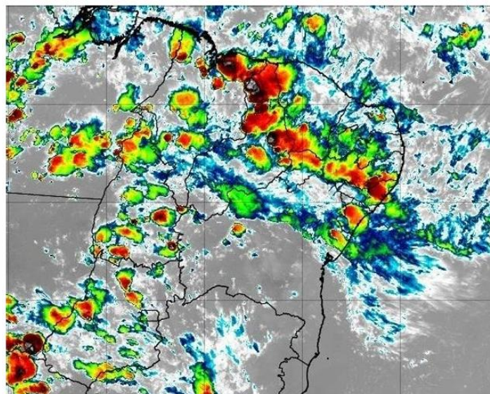
Figura 3 - Imagem de satélite no infravermelho com realce do satélite GOES-19 as 21::00 UT do dia 18/02. As cores indicam diferentes temperaturas dos topos das nuvens.
