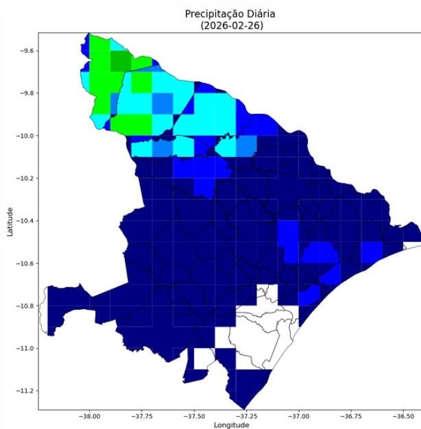
Figura 14 - Mapa de precipitação observada de 26 de fevereiro.
