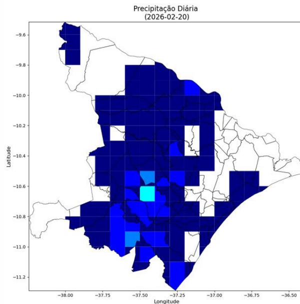
Figura 9 - Mapa de precipitação observada dia 20 de fevereiro.
