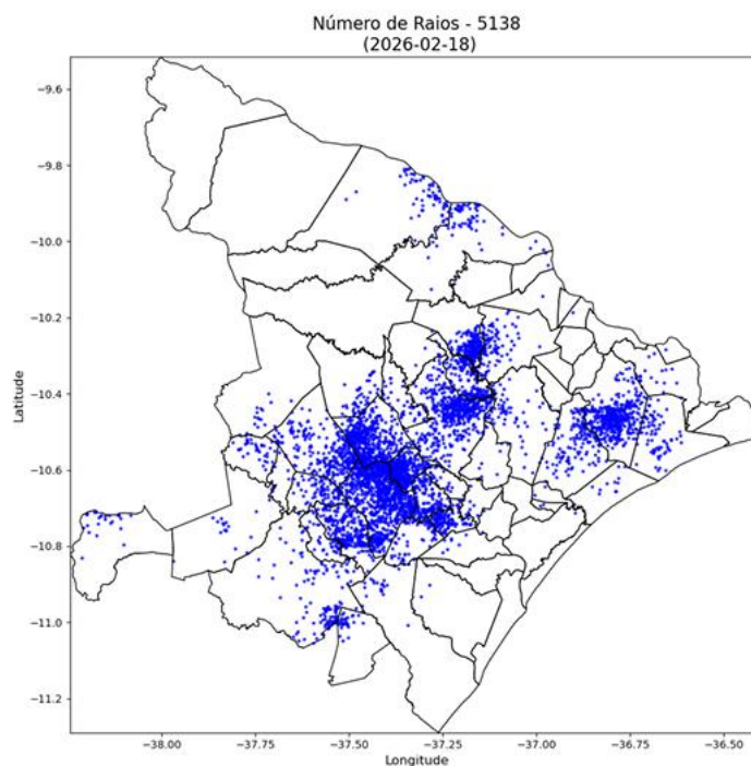
Figura 21 - Registros de descargas atmosféricas no dia 18 de fevereiro.
