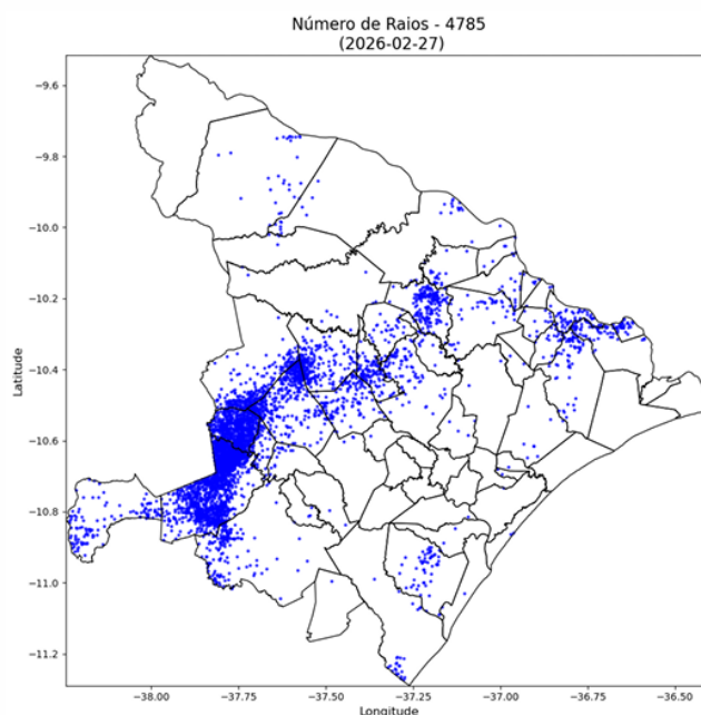
Figura 28 - Registros de descargas atmosféricas no dia 27 de fevereiro.
