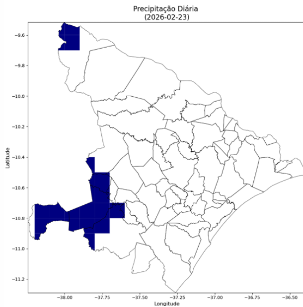
Figura 12 - Mapa de precipitação observada dia 23 de fevereiro.
