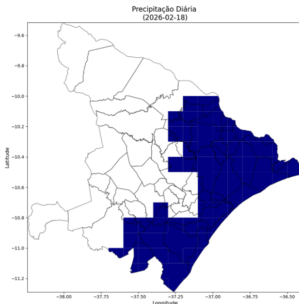
Figura 7 - Mapa de precipitação observada dia 18 de fevereiro.
