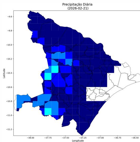
Figura 10 - Mapa de precipitação observada dia 21 de fevereiro.
