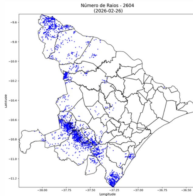
Figura 27 - Registros de descargas atmosféricas no dia 26 de fevereiro.
