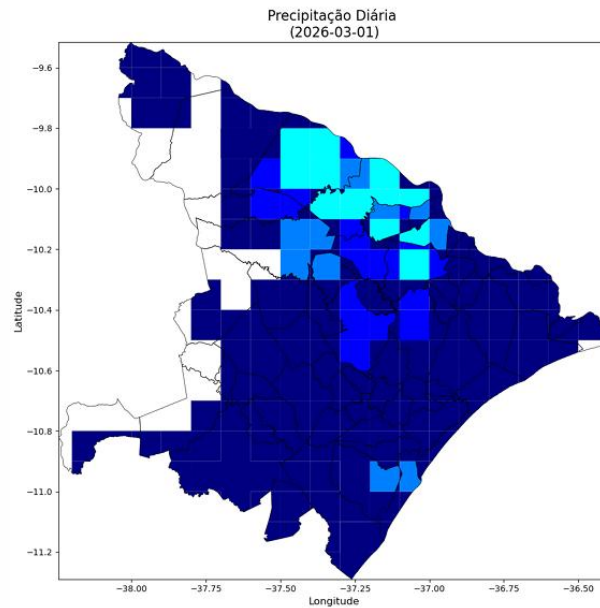
Figura 17 - Mapa de precipitação observada de 01 de março.
