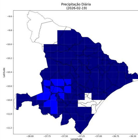
Figura 8 - Mapa de precipitação observada dia 19 de fevereiro.
