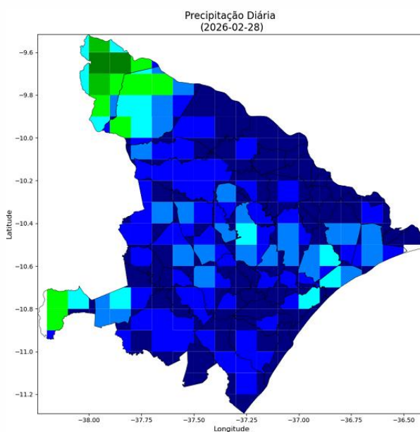
Figura 16 - Mapa de precipitação observada de 28 de fevereiro.
