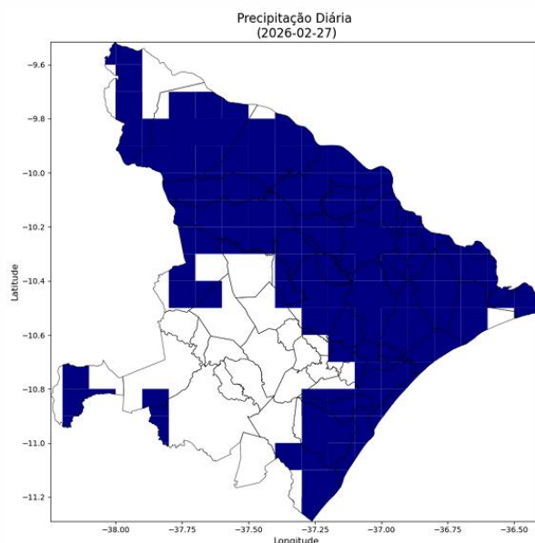
Figura 15 - Mapa de precipitação observada de 27 de fevereiro.
