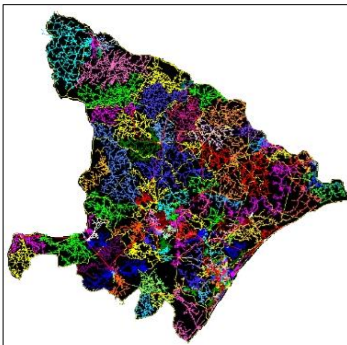
Figura 2 - Mapa Geoelétrico da Região
