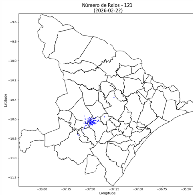
Figura 25 - Registros de descargas atmosféricas no dia 22 de fevereiro.
