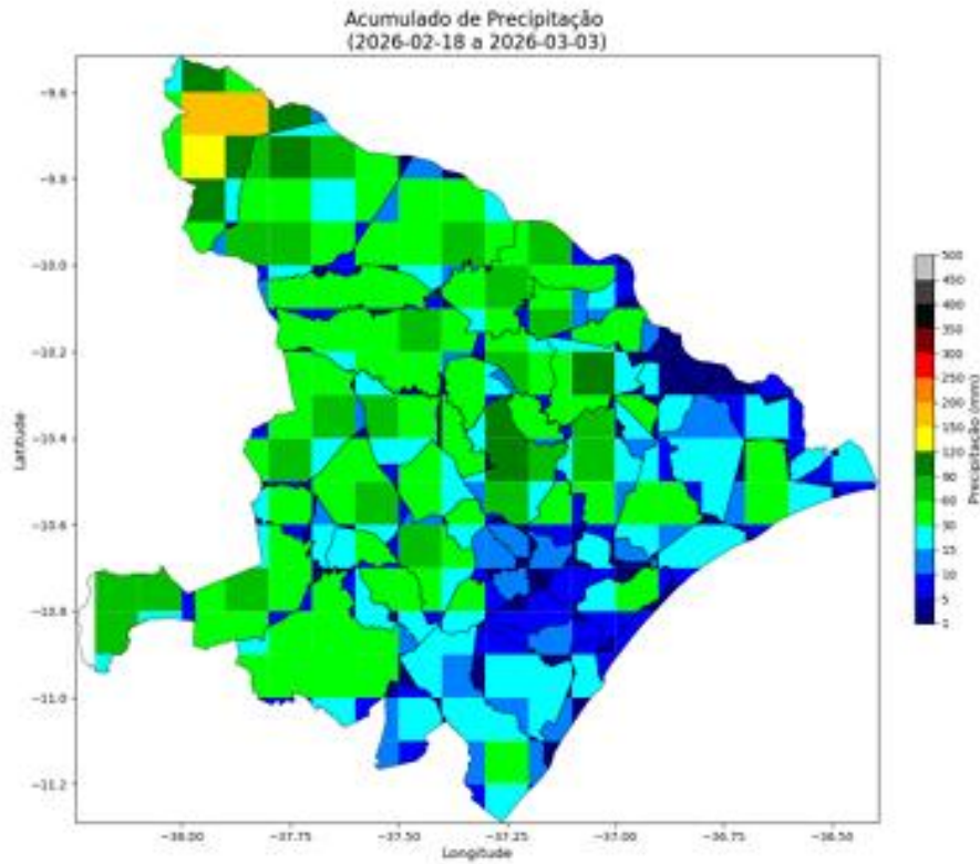
Figura 3 – Mapa de precipitação para os dias 18/02 a 03/03 e o acumulado no período. Dia 25/02 não foi registrado chuvas.
