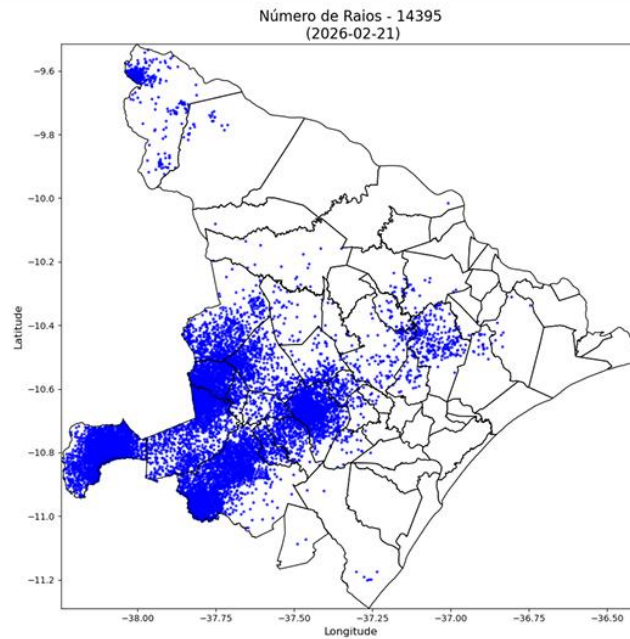
Figura 24 - Registros de descargas atmosféricas no dia 21 de fevereiro.
