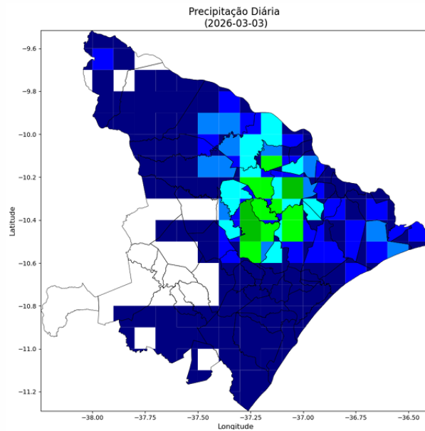
Figura 19 - Mapa de precipitação observada de 03 de março.
