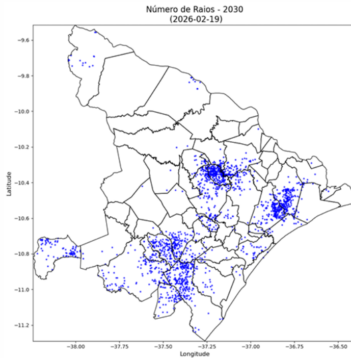
Figura 22 - Registros de descargas atmosféricas no dia 19 de fevereiro.
