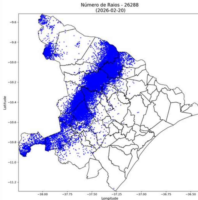
Figura 23 - Registros de descargas atmosféricas no dia 20 de fevereiro.
