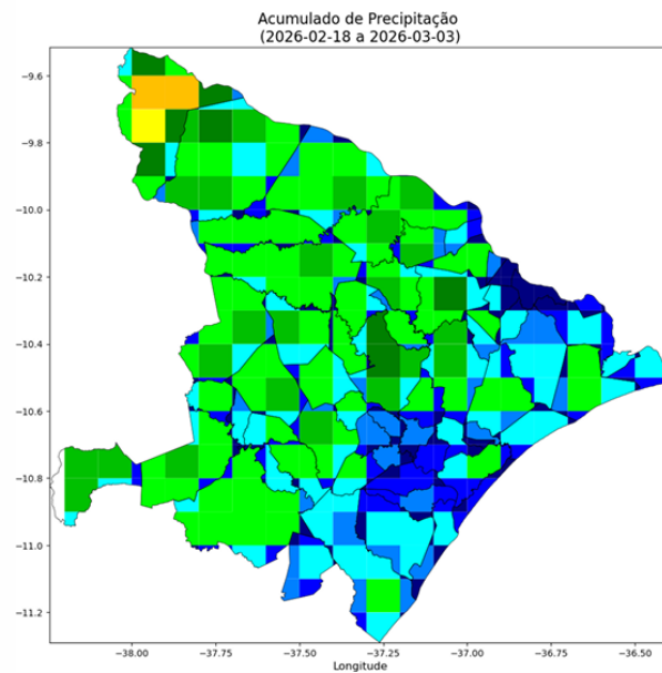
Figura 20 - Mapa de precipitação acumulada de 18 de fevereiro a 03 de março.
