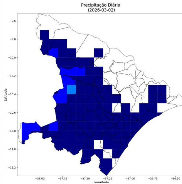
Figura 18 - Mapa de precipitação observada de 02 de março.
