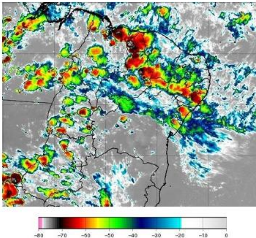
Figura 1 - Imagem de satélite no infravermelho com realce do satélite GOES-19 as 21:00 UT do dia 18/02. As cores indicam diferentes temperaturas dos topos das nuvens.
