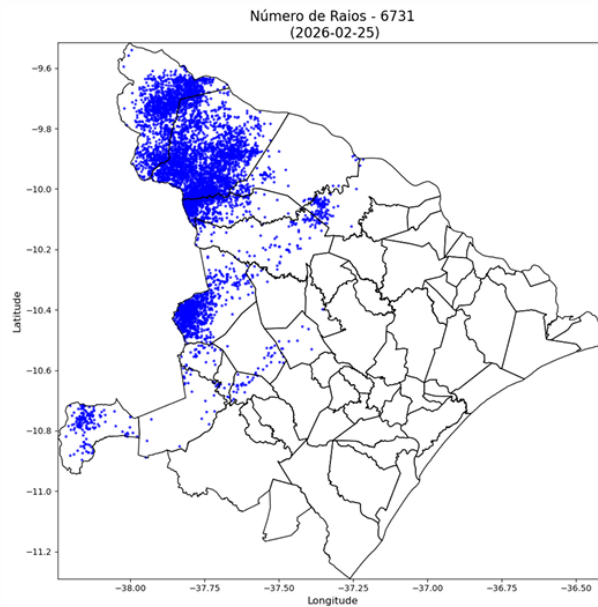
Figura 26 - Registros de descargas atmosféricas no dia 25 de fevereiro.
