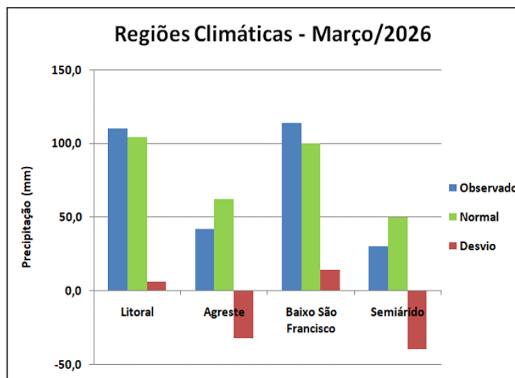
Figura 5 - Precipitação acumulada para o mês de março de 2026
