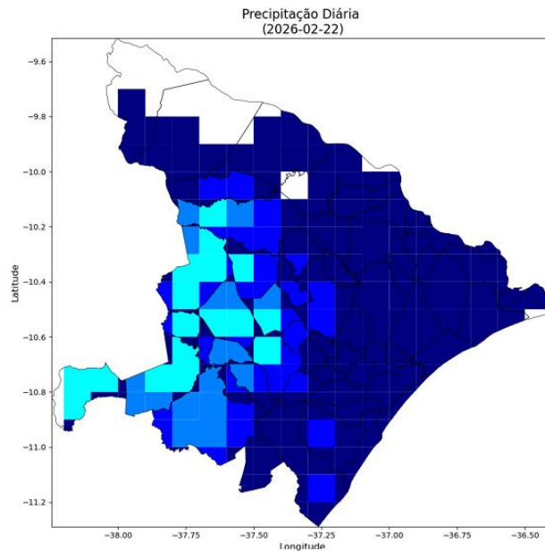
Figura 11 - Mapa de precipitação observada dia 22 de fevereiro.
