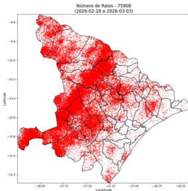
Figura 2 – Mapa de incidência de descargas atmosféricas nuvem-solo e intranuvem para os dias 18/02 a 03/03 e o acumulado no período. Cada ponto corresponde ao local de ocorrência de uma descarga.
