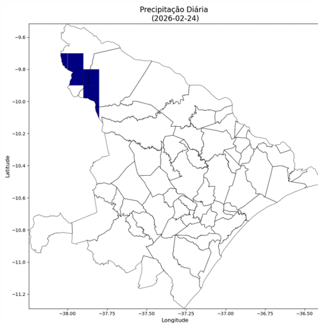
Figura 13 - Mapa de precipitação observada de 24 de fevereiro.
