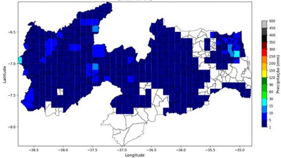
Precipitação Diária (2026-02-17)
