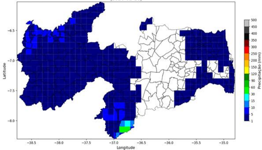
Precipitação Diária (2026-02-19)
