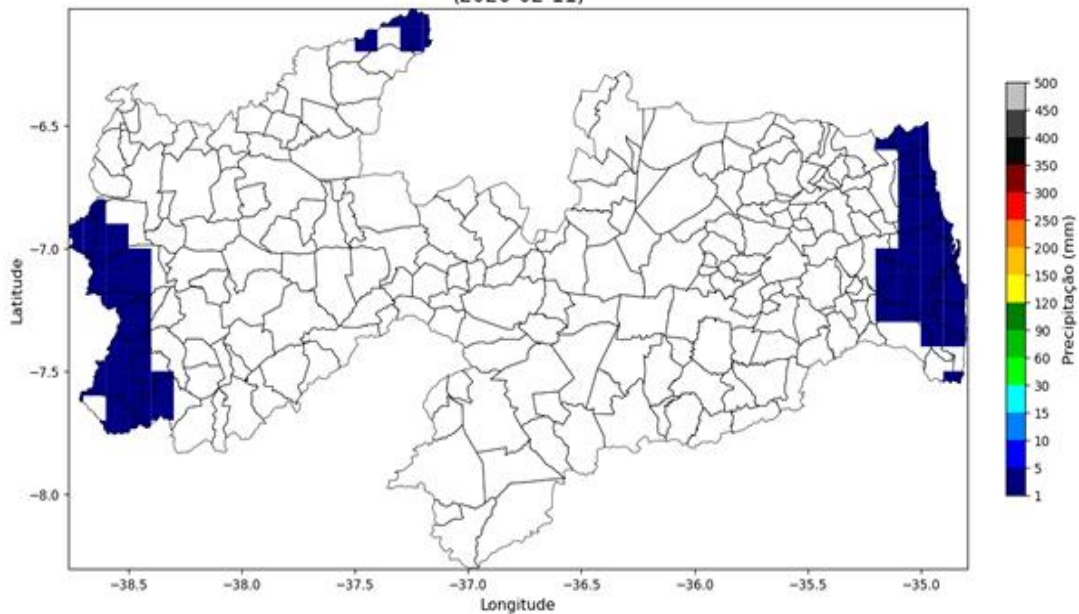
Precipitação Diária (2026-02-11)
