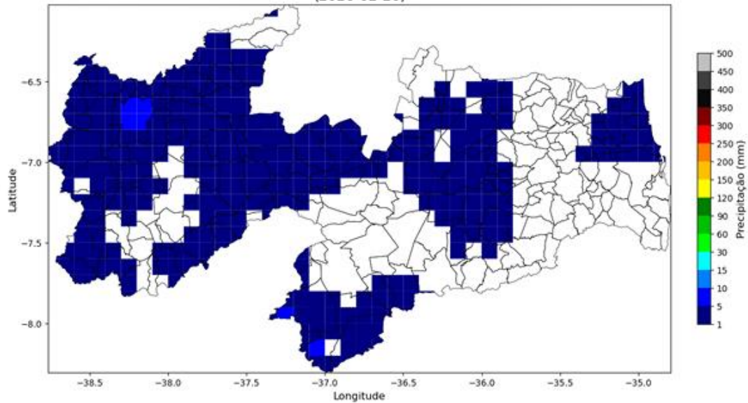
Precipitação Diária (2026-02-21)
