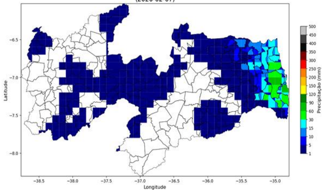
Precipitação Diária (2026-02-07)
