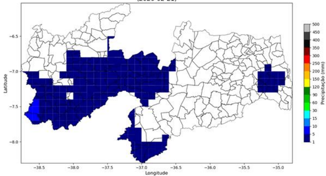
Precipitação Diária (2026-02-21)
