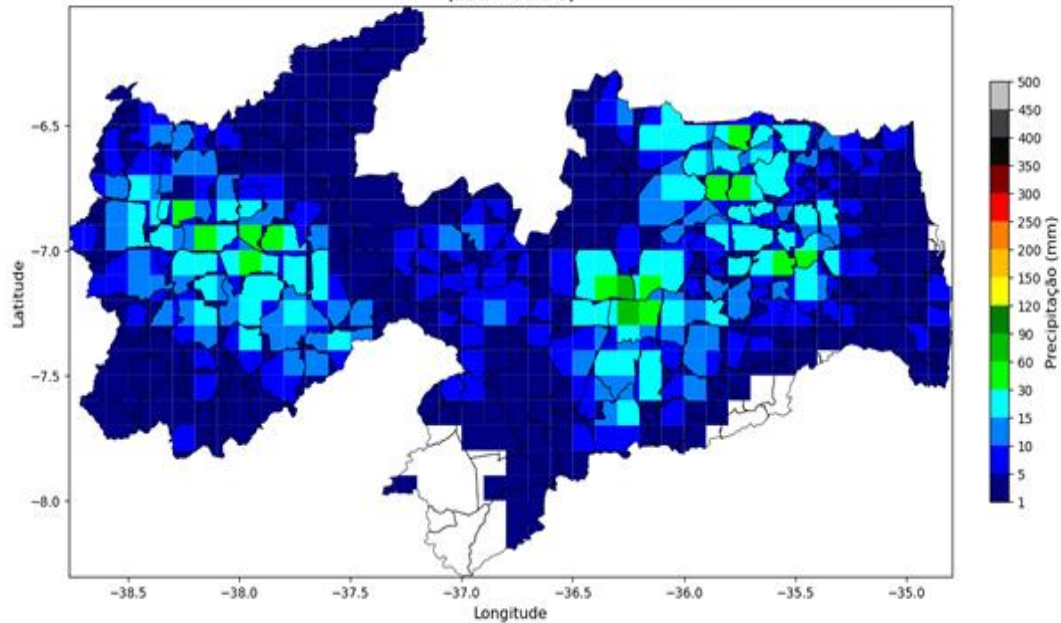
Precipitação Diária (2026-02-07)
