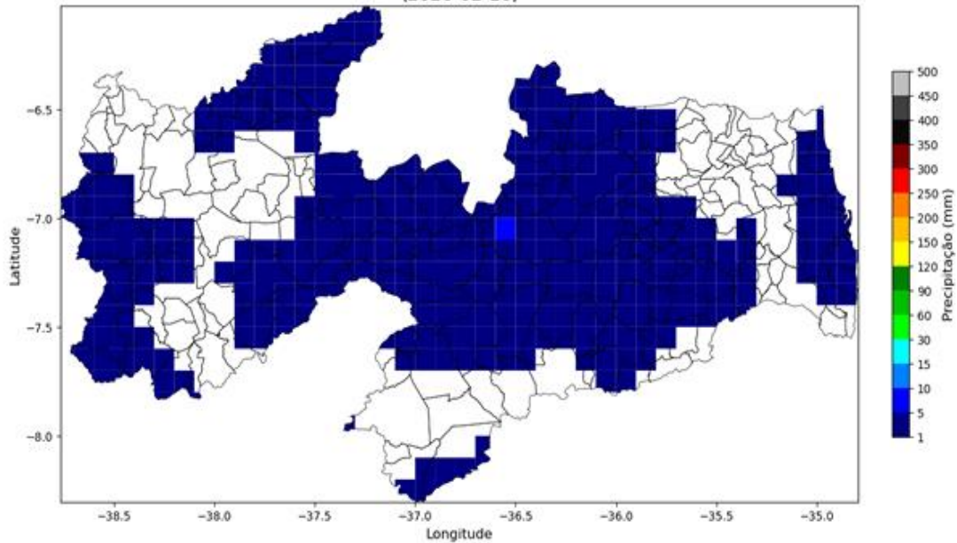
Precipitação Diária (2026-02-11)
