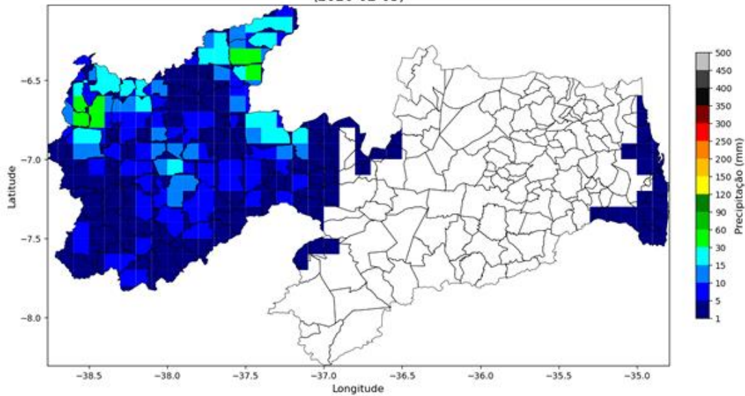
Precipitação Diária (2026-02-05)
