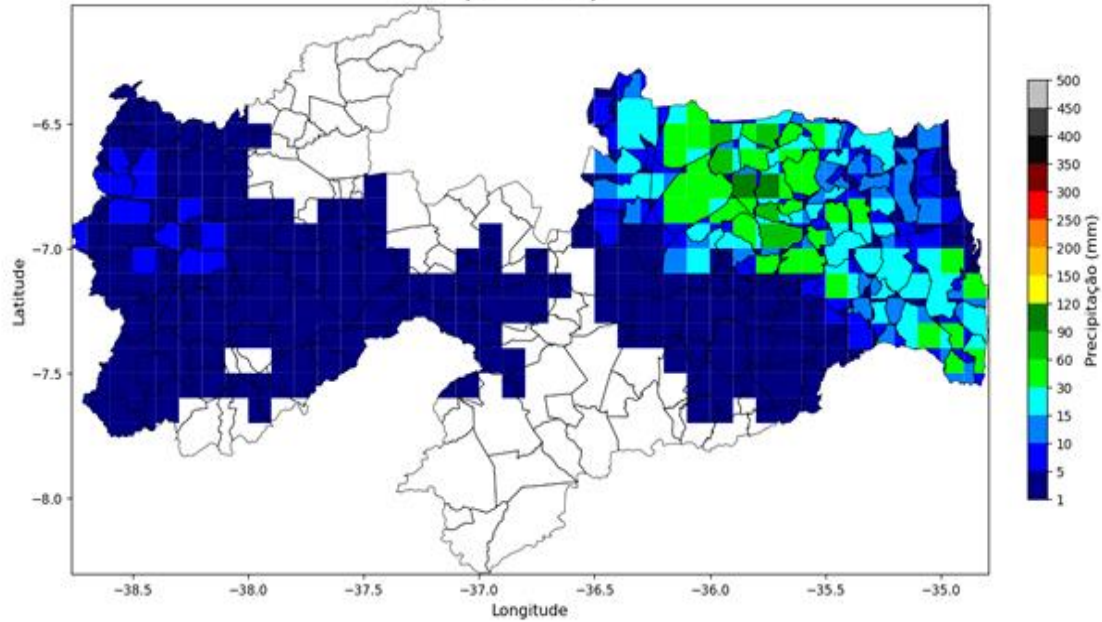
Precipitação Diária (2026-02-13)
