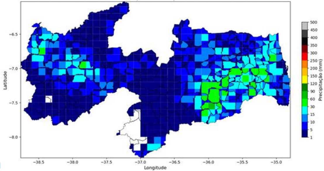
Precipitação Diária (2026-02-09)
