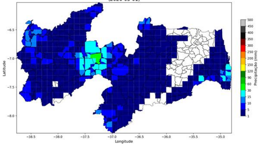
Precipitação Diária (2026-03-01)
