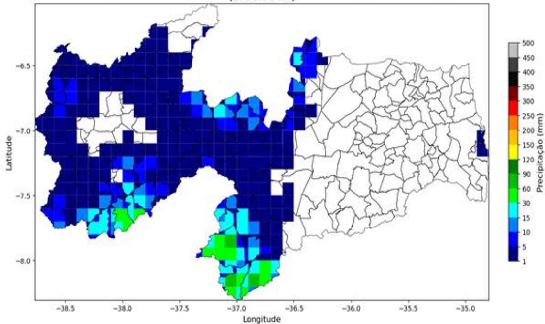
Precipitação Diária (2026-02-27)
