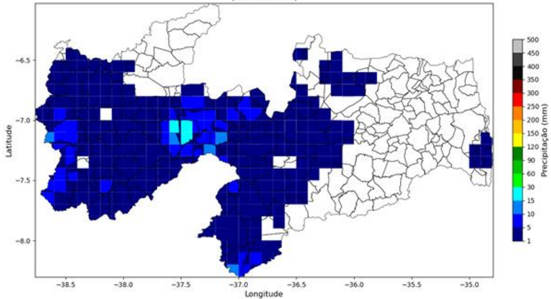
Precipitação Diária (2026-02-23)
