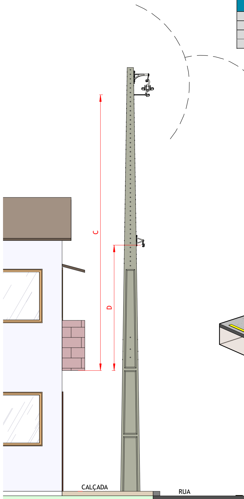
VISTA LATERAL
