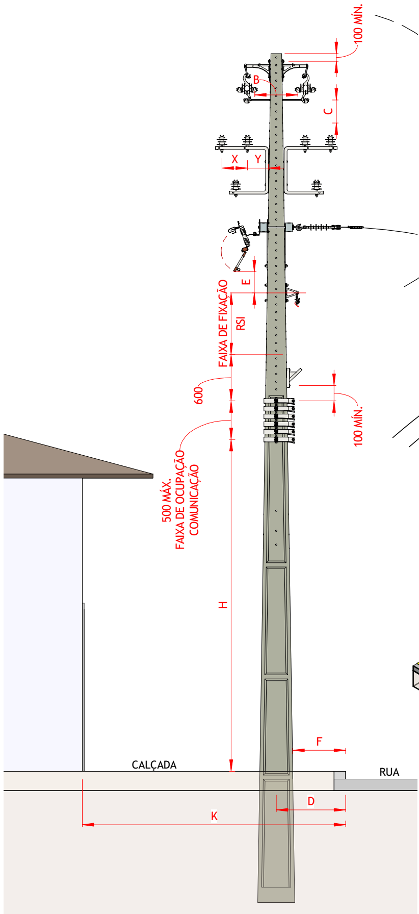
VISTA LATERAL
