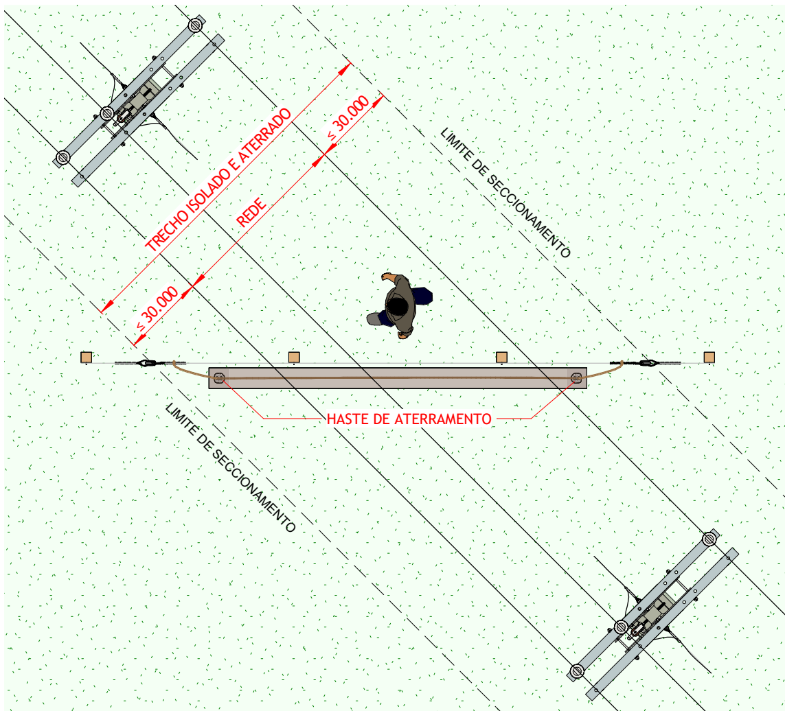
VISTA SUPERIOR
