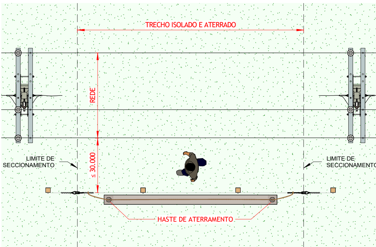
VISTA SUPERIOR
