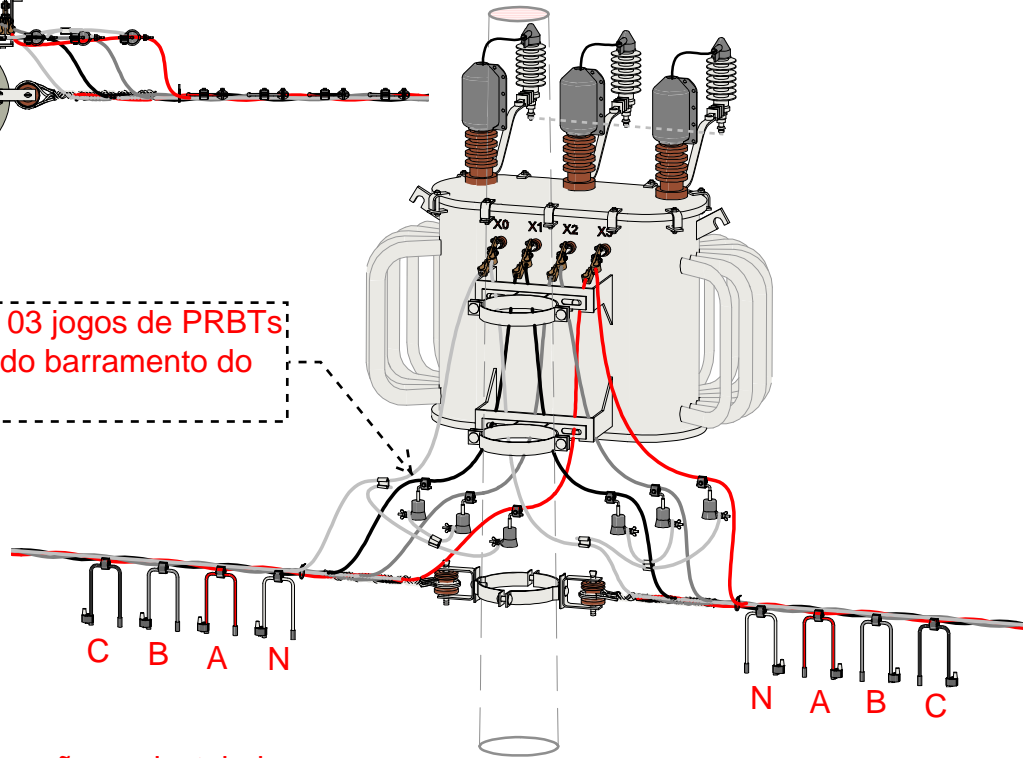
EM PERSPECTIVA
