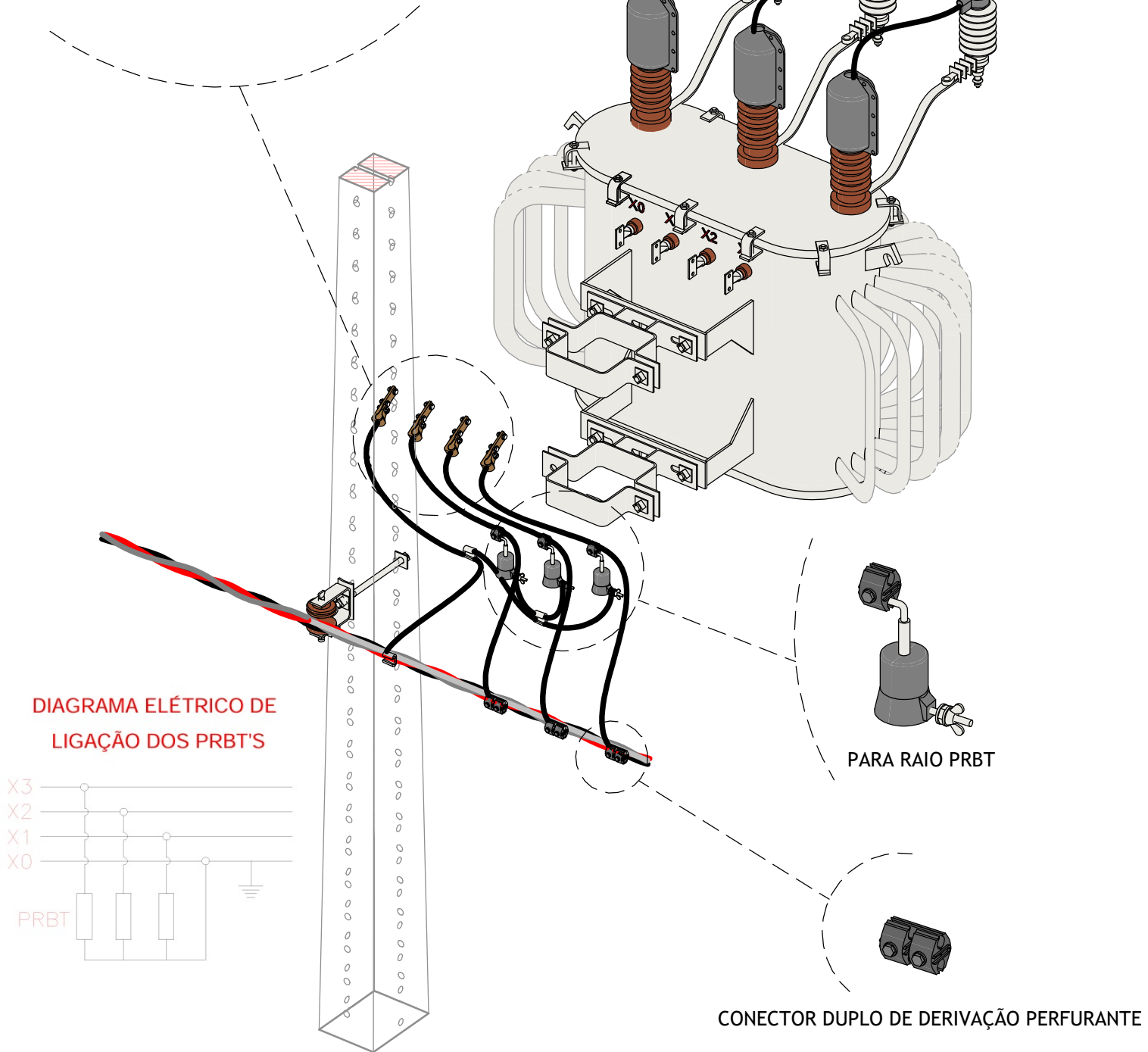
DETALHE MONTAGEM
