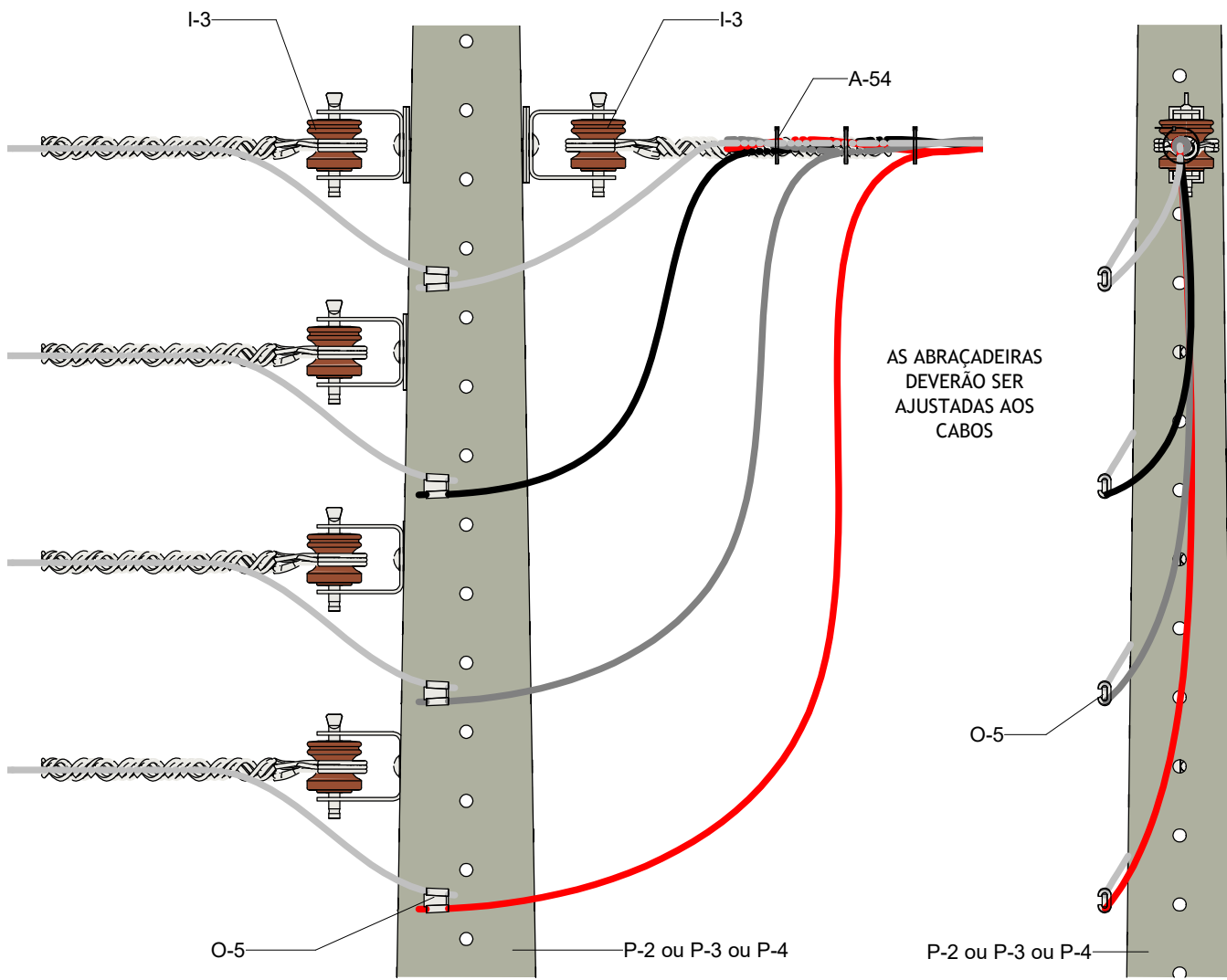
VISTA FRONTAL 1 : 10
