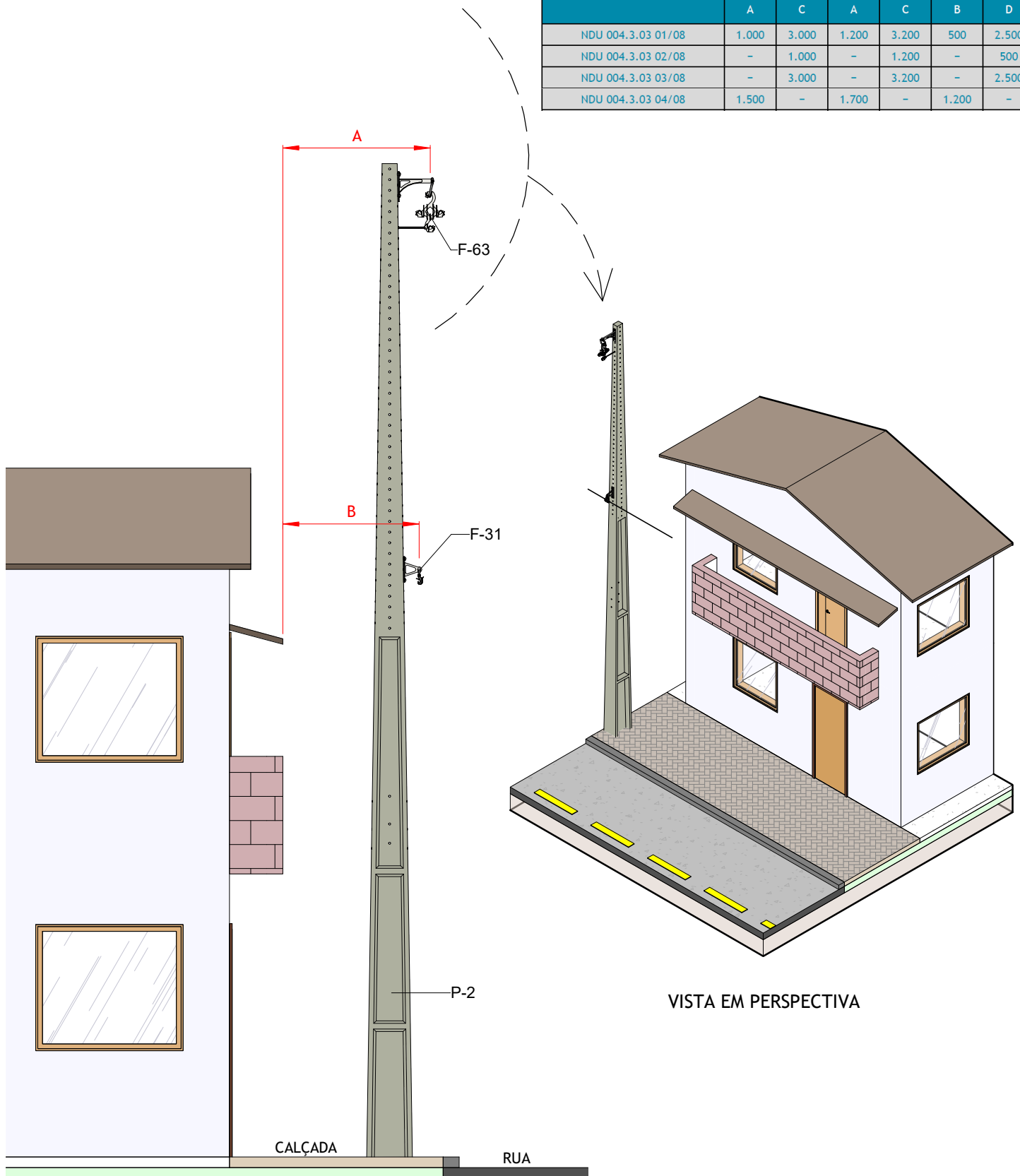
VISTA LATERAL
