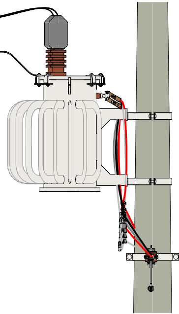
VISTA LATERAL 1 : 25
