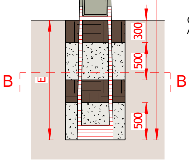
VISTA CORTE A 1 : 50
