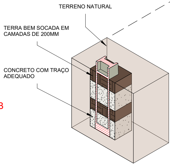
VISTA EM PERSPECTIVA - DETALHE
