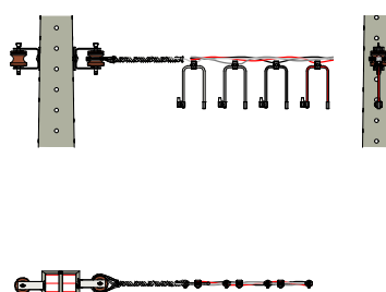
SI3 - FOLHA 09/13
