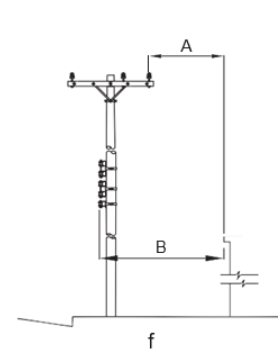
Afastamentos horizontal entre os condutores e a cimalha e o telhado de edificações
