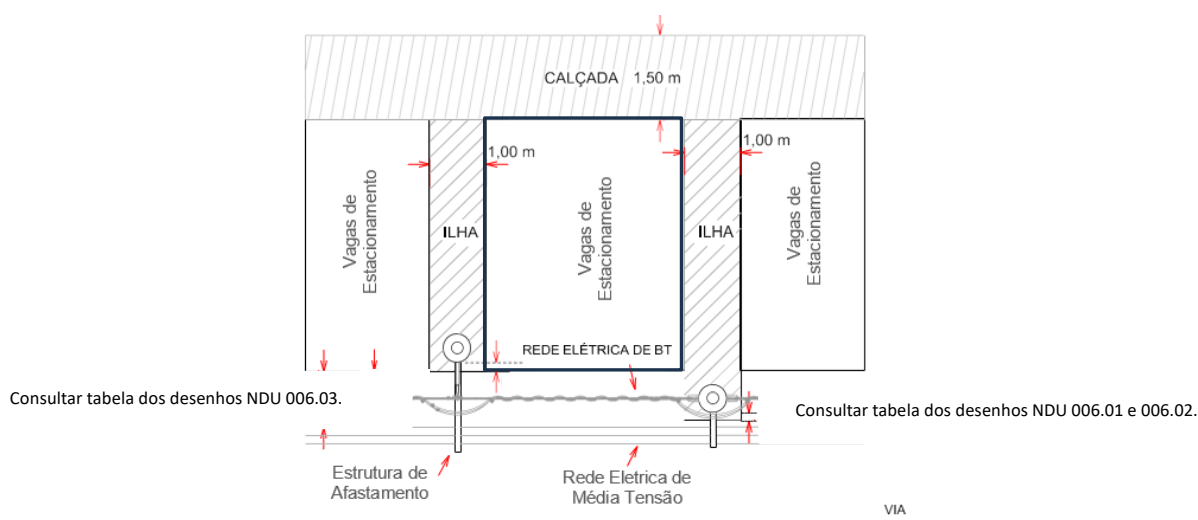
Figura 07. Localização de postes ao lado de vagas de estacionamento.
