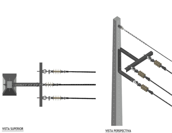
Estrutura CE 3
