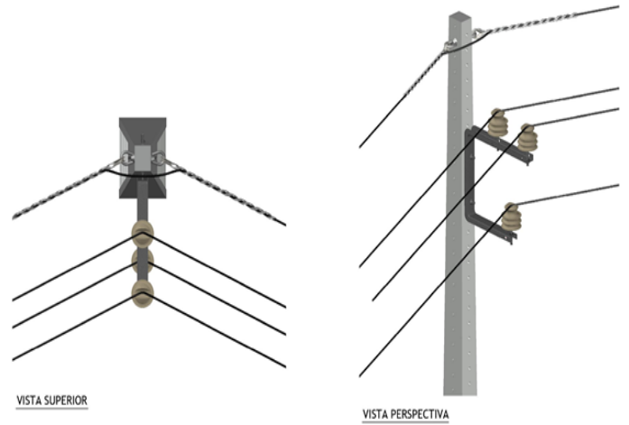
Estrutura CE 2
