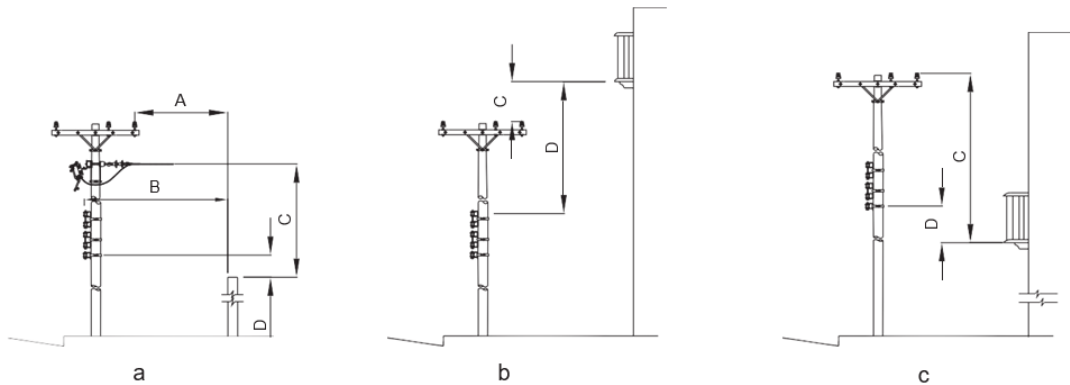
Afastamentos horizontal e vertical entre os condutores e o muro
