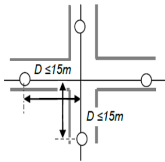
Figura 04. Cruzamento aéreo.
