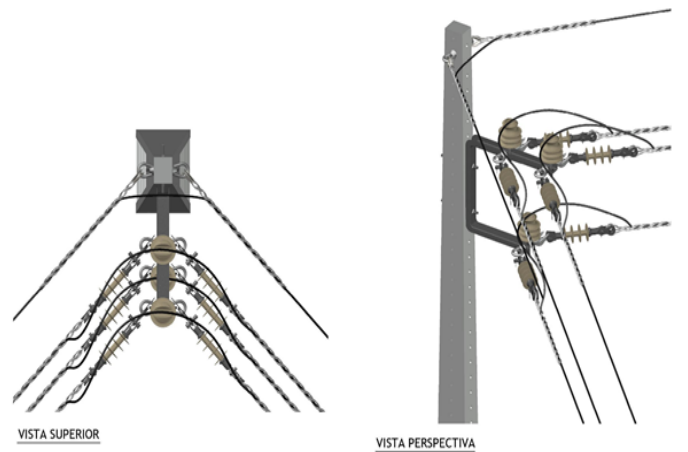
Estrutura CE 4
