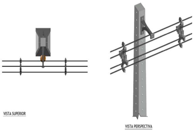
Estrutura CE 1
