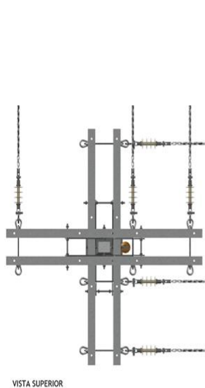
Estrutura N3
