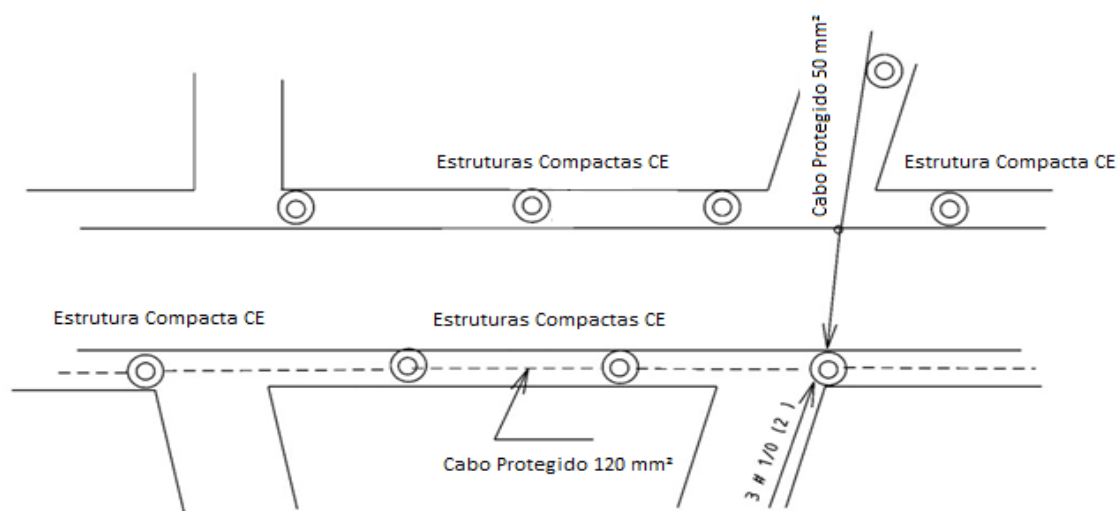
Disposição unilateral
