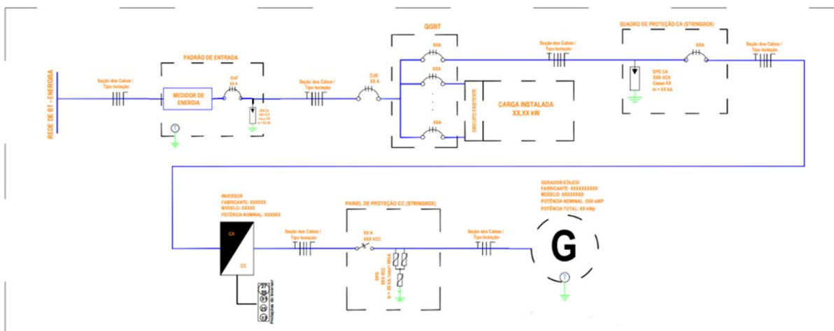
Diagrama Unifilar s/ Transformador de Acoplamento
