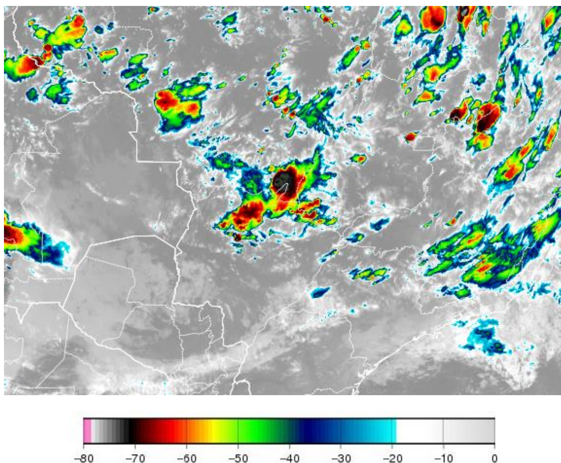
Figura 1 - Imagem de satélite no infravermelho com realce do satélite GOES-19 as 21:00 UT do dia 10/04. As cores indicam diferentes temperaturas dos topos das nuvens.
