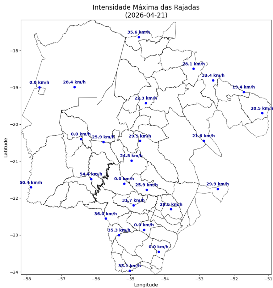
Figura 4 – Mapa de rajadas para os dias 10 a 21/04.
