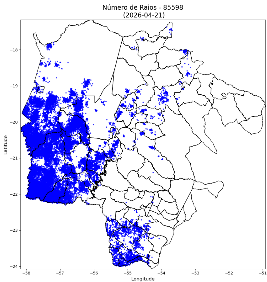
Figura 2 – Mapa de incidência de descargas atmosféricas nuvem-solo e intranuvem para os dias 10 a 21/04.
