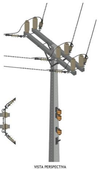
Estrutura N4
