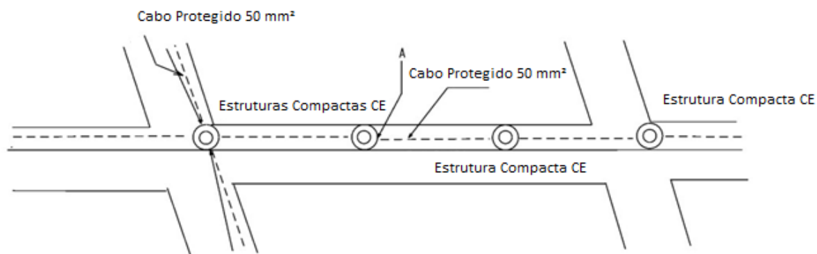
Disposição unilateral
