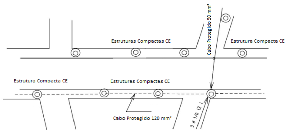
Disposição unilateral
