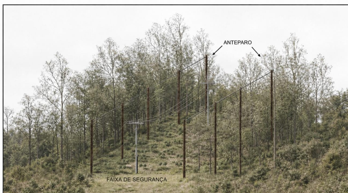
Figura 05. Exemplo de barreira/Anteparo aplicável a árvores de grande porte – Responsabilidade donos das Glebas
