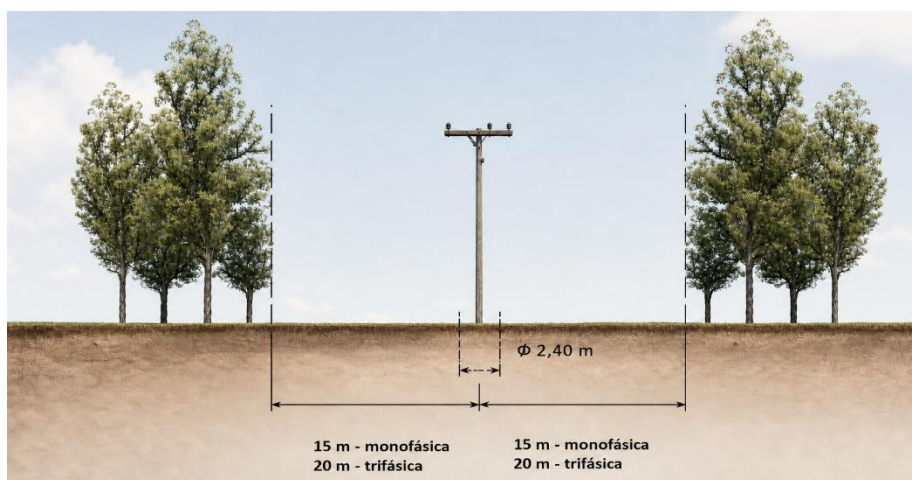
Figura 04. Faixa de segurança para árvores de grande porte (comprimento superior a 10 metros).
